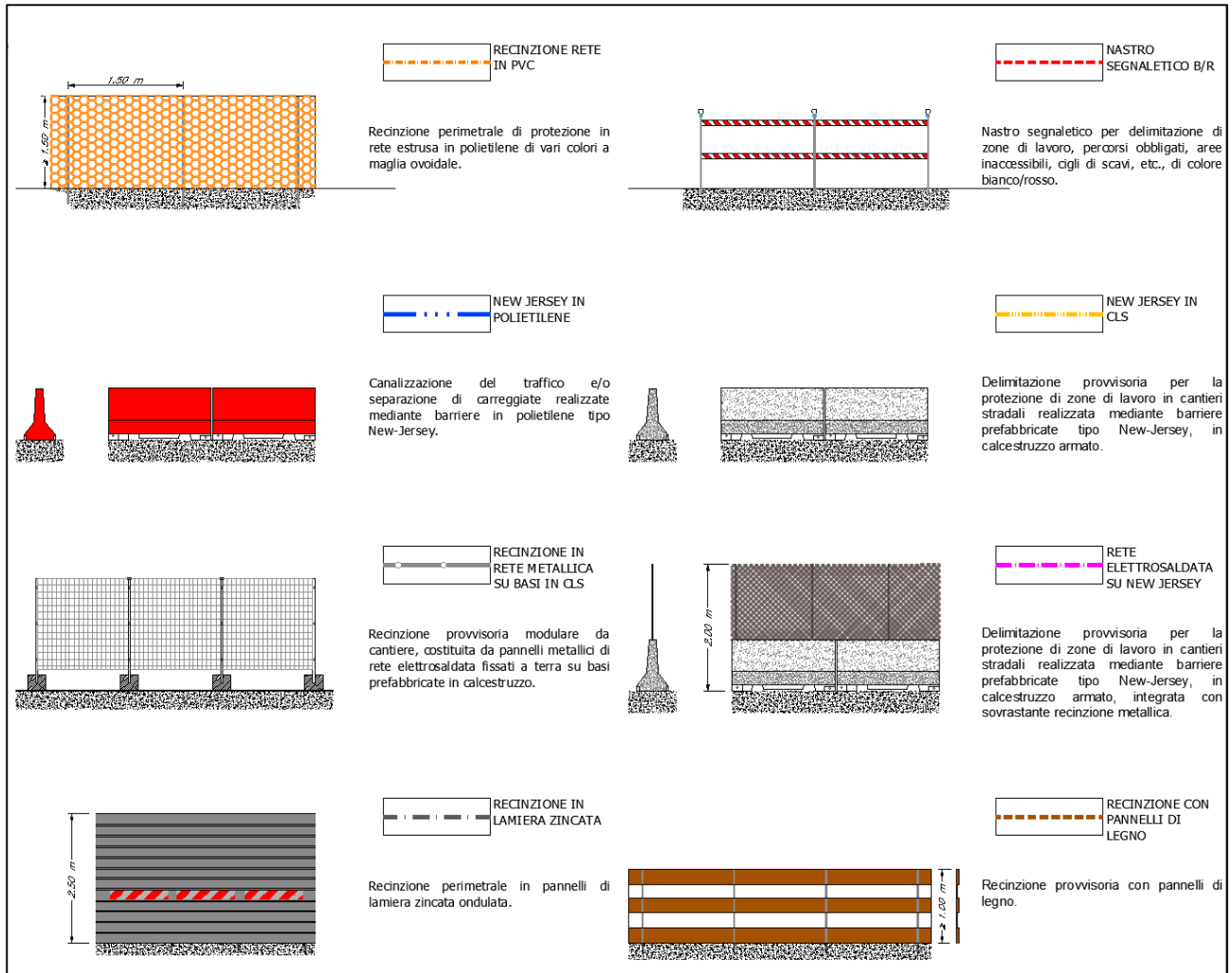
Figura 2-1 Recinzioni tipo
