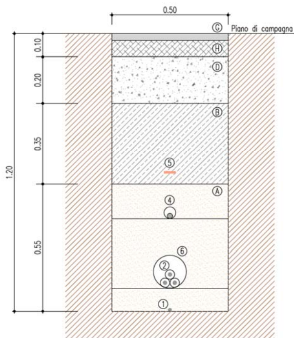
SEZIONE TIPO 1B - SU STRADA ASFALTATA
