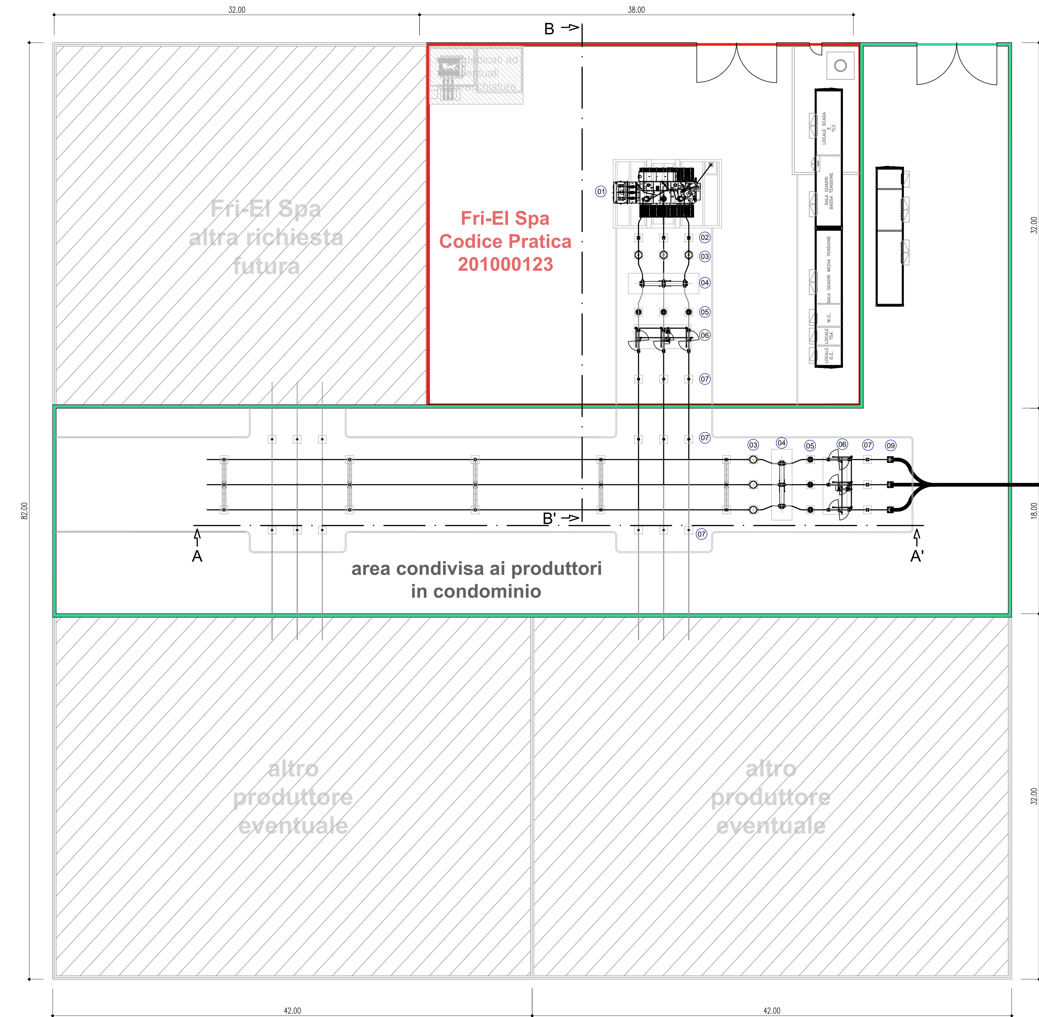
PLANIMETRIA (SCALA 1 : 200)
