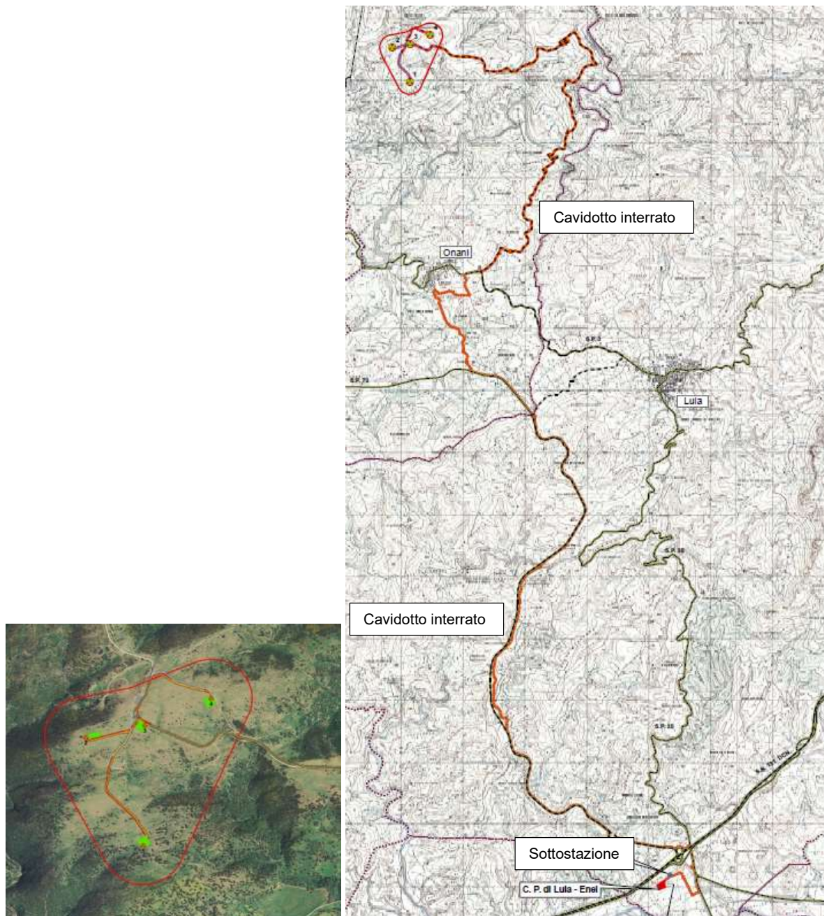
Fig. 3.4 – Alternativa 2: Rappresentazione degli aerogeneratori (Ortofoto e Carta I.G.M.)
