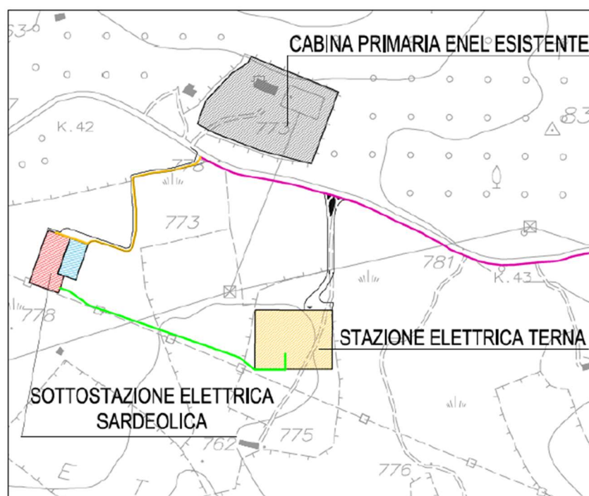
Fig. 3.11 – Inquadramento della sottostazione elettrica Sardeolica S.r.l. (in rosso) e dell'area per il futuro accumulo energetico (in celeste)
