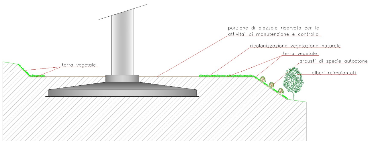
Fig. 5.1 – Interventi di ripristino ambientale nelle piazzole
