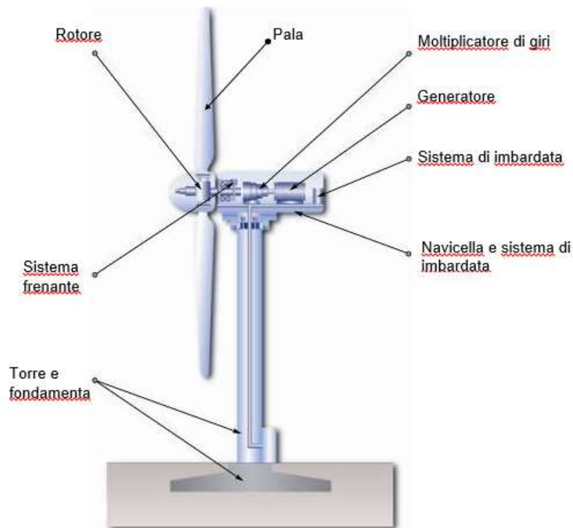
Fig. 3.2 - Schema dell'aerogeneratore
