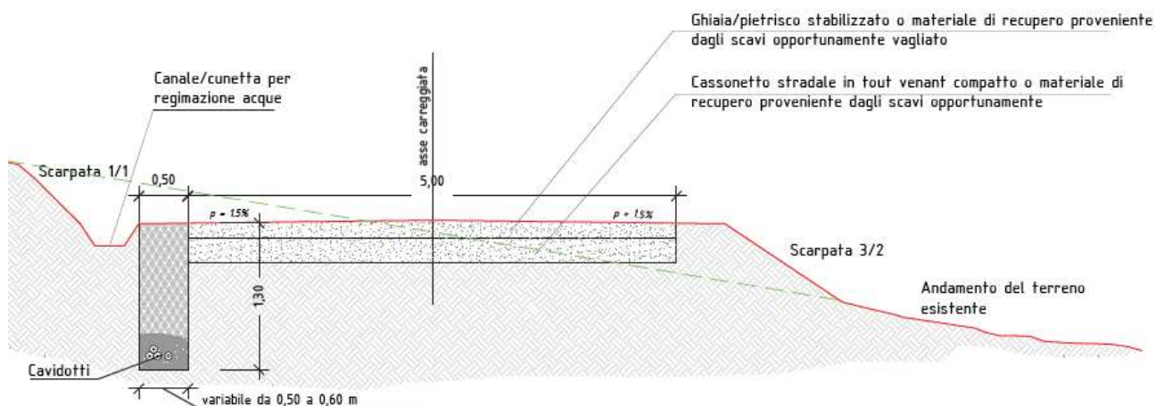
Fig. 3.5 - Sezione tipo per strade di nuova realizzazione
