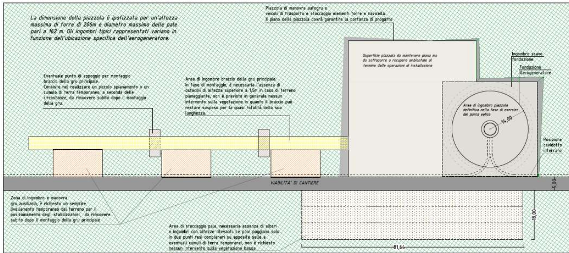
Fig. 3.8 – Piazzola tipo per gli aerogeneratori – fase di cantiere
