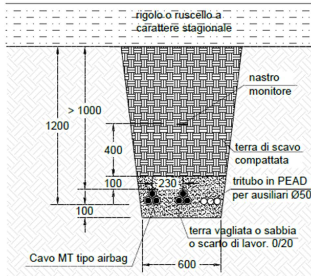
Fig. 3.9 – Attraversamento di rigolo o ruscello con due cavi airbag
