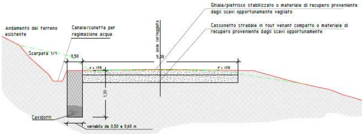
Fig. 3.6 - Sezione tipo per strada preesistente sterrata da adeguare
