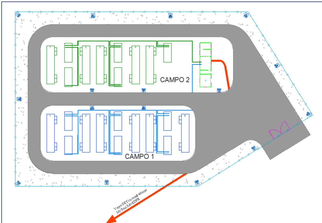
stralcio Layout impianto San Severo (FG)
