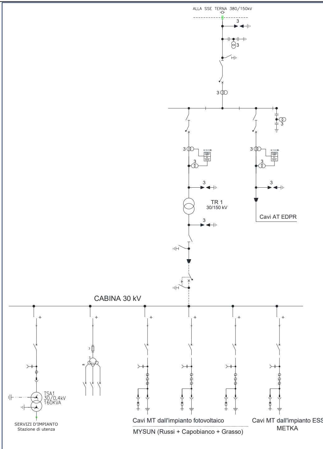
Schema di principio del collegamento dell'impianto ESS alla stazione di rete
