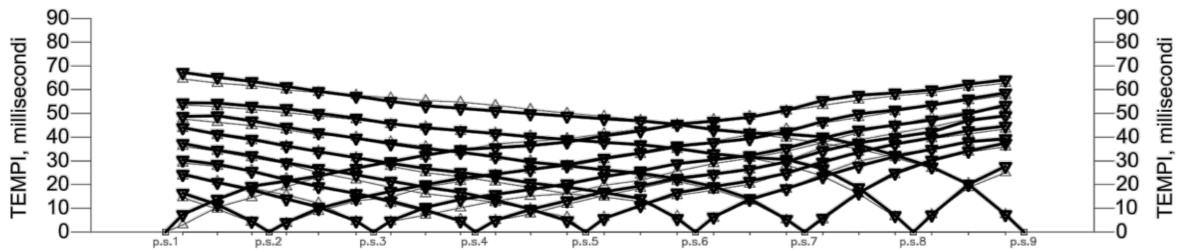
Profilo sismico a rifrazione LS10
