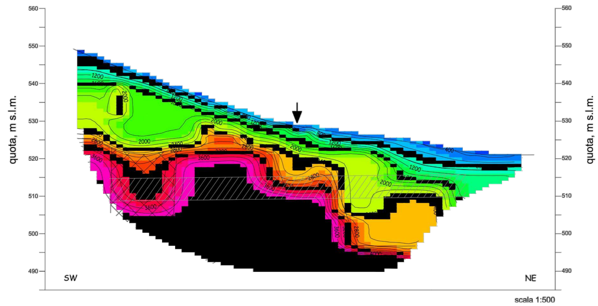
Profilo sismico a rifrazione LS3
