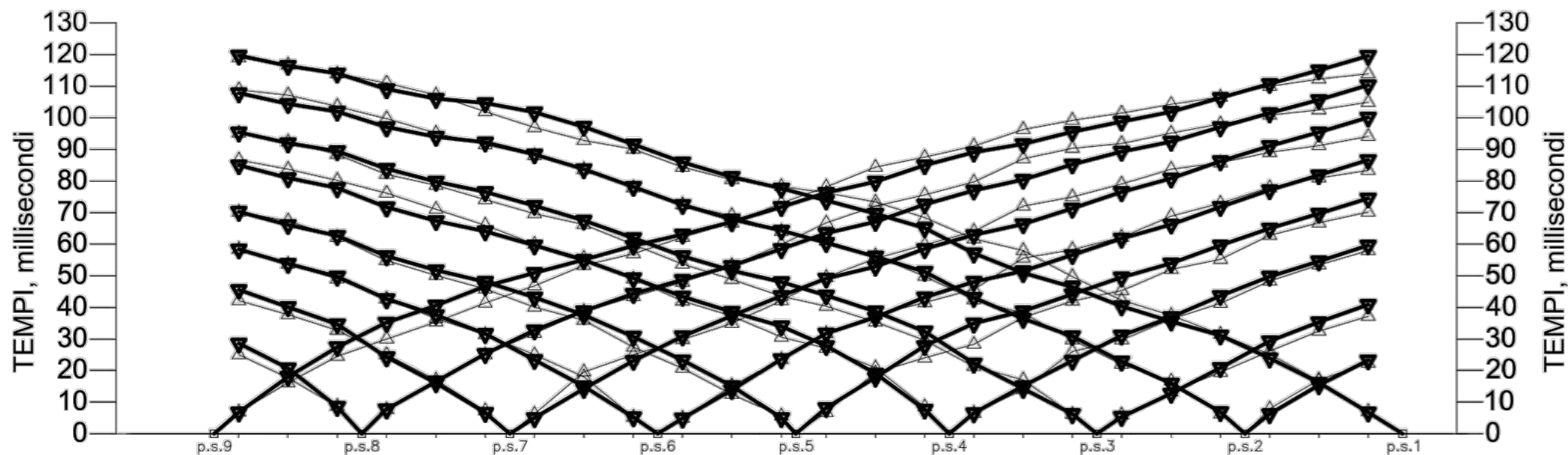
Profilo sismico a rifrazione LS3
