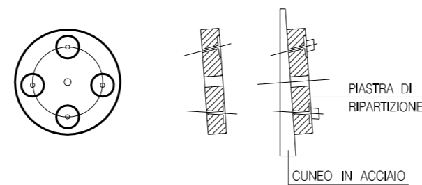
PARTICOLARE PIASTRA
