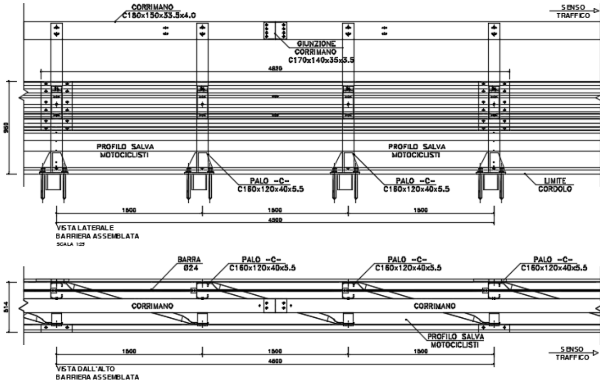
Vista laterale e dall'alto barriera ANAS H4 BPSM
