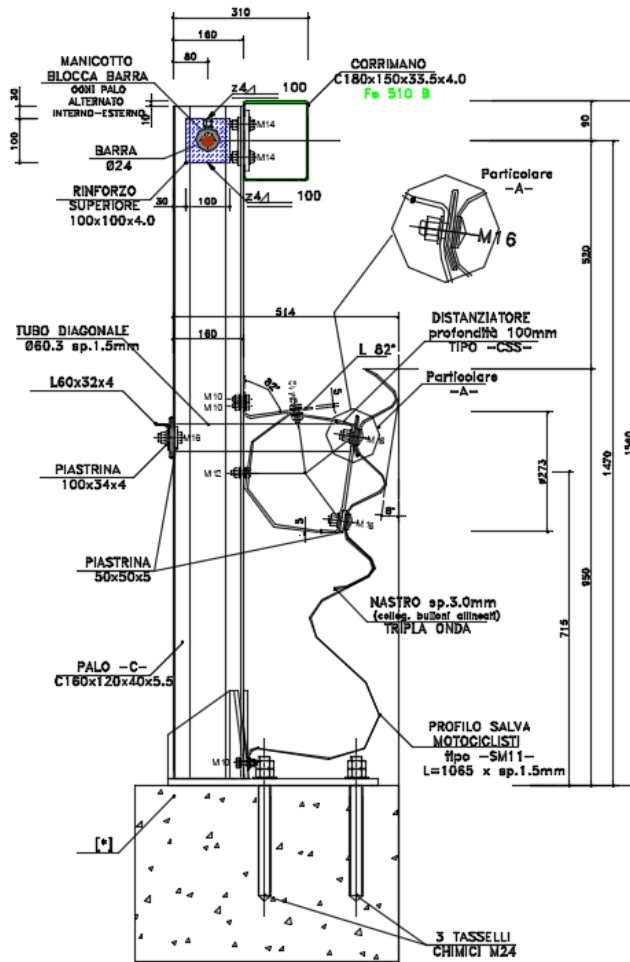
Sezione barriera ANAS H4 BPSM
