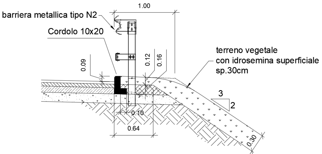
Margine laterale con barriere N2 commerciale
