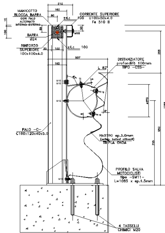
Sezione barriera ANAS H2 BPSM
