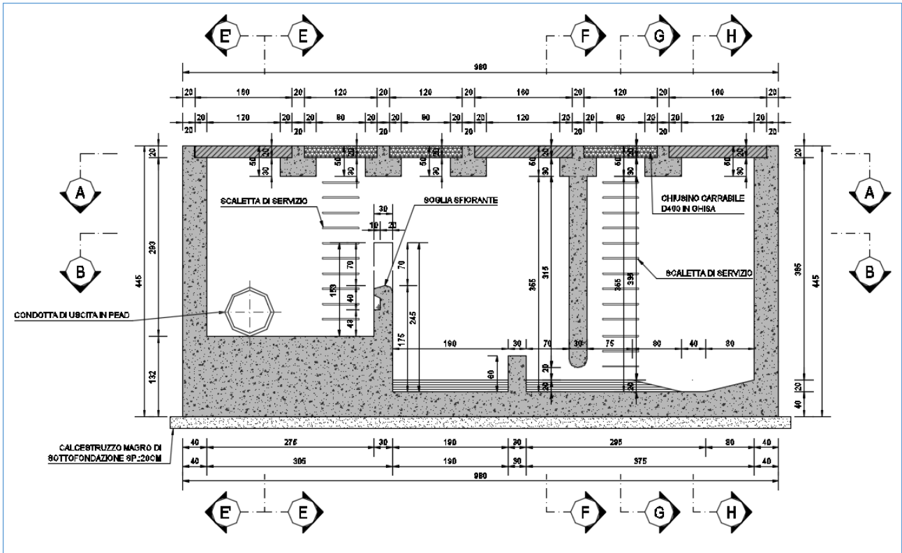
FIGURA 2: SEZIONE LONGITUDINALE
