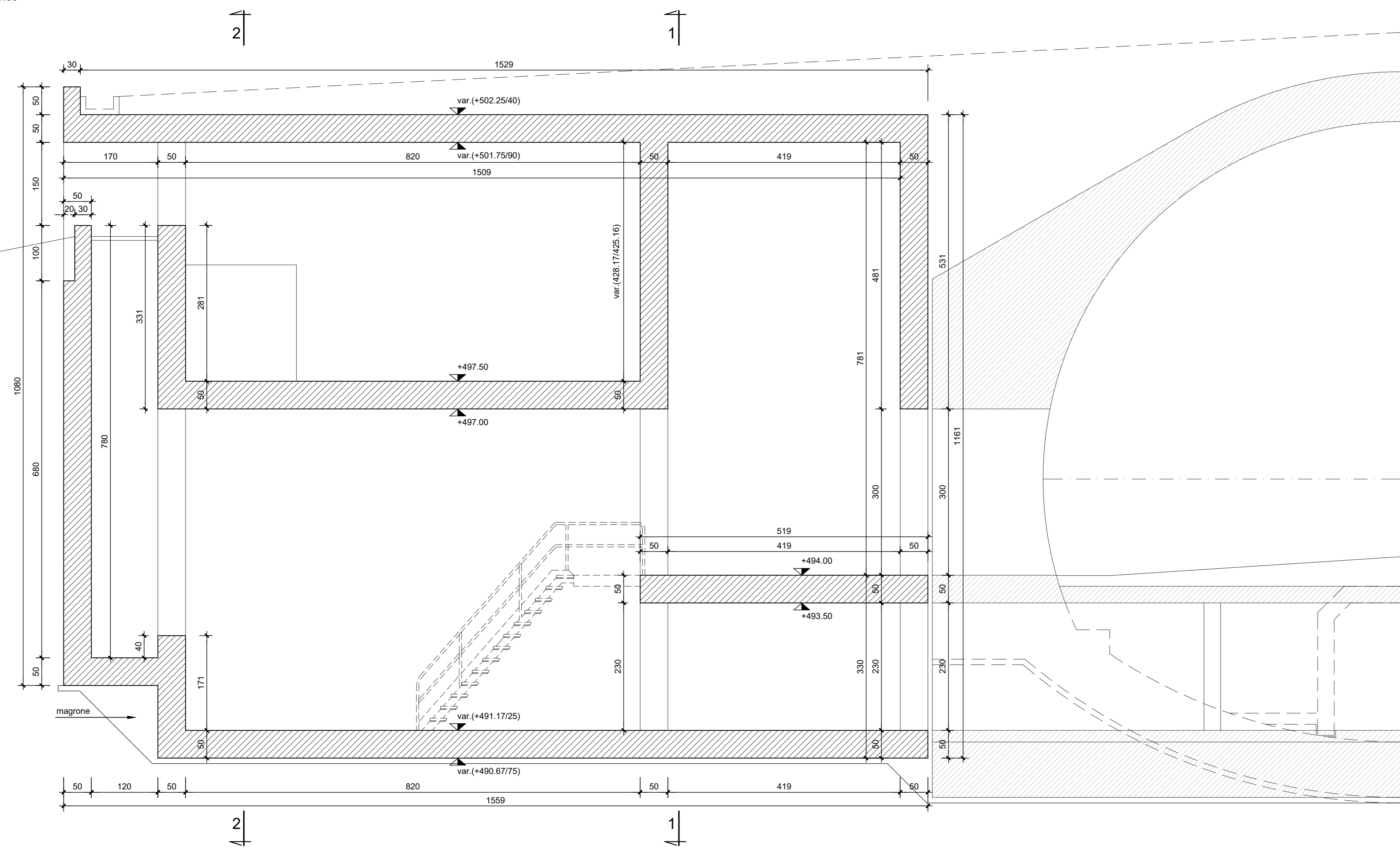
SEZIONE 3-3 SCALA 1:50
