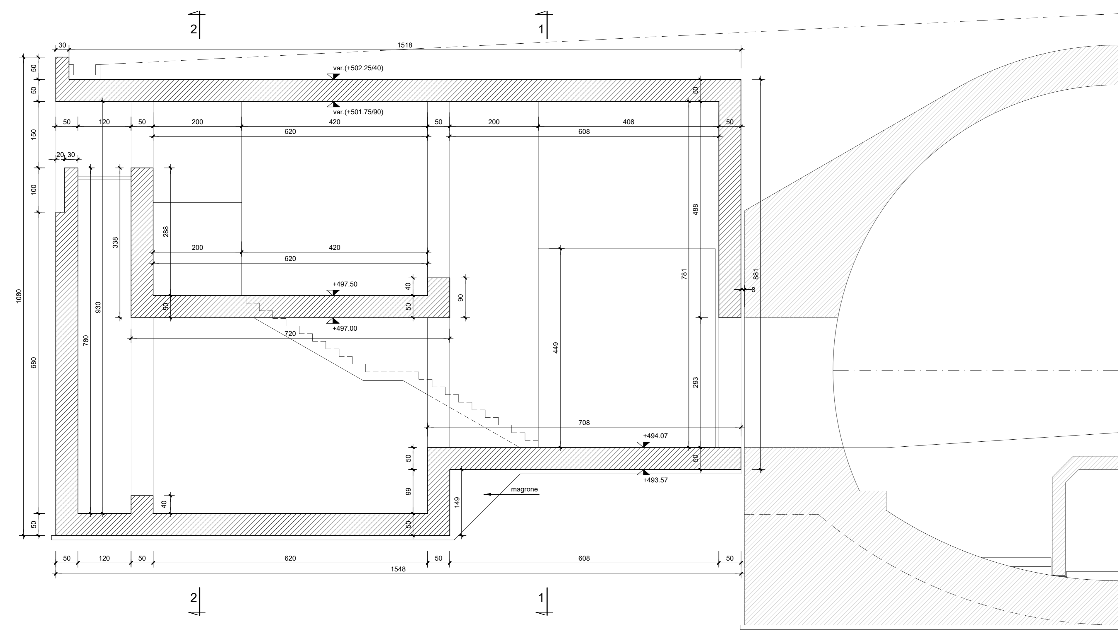
SEZIONE 5-5 SCALA 1:50
