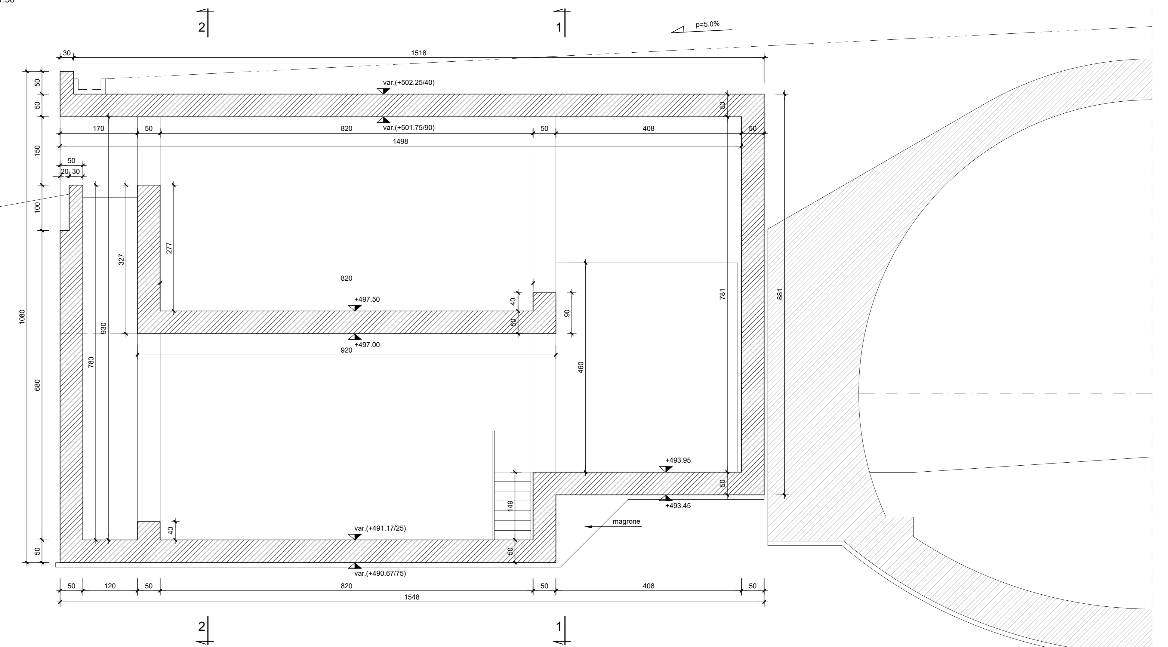
SEZIONE 4-4 SCALA 1:50
