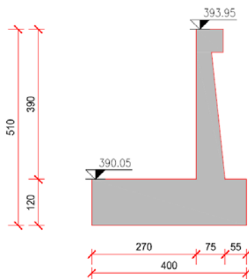
Fig. 1 Sezione trasversale concio
