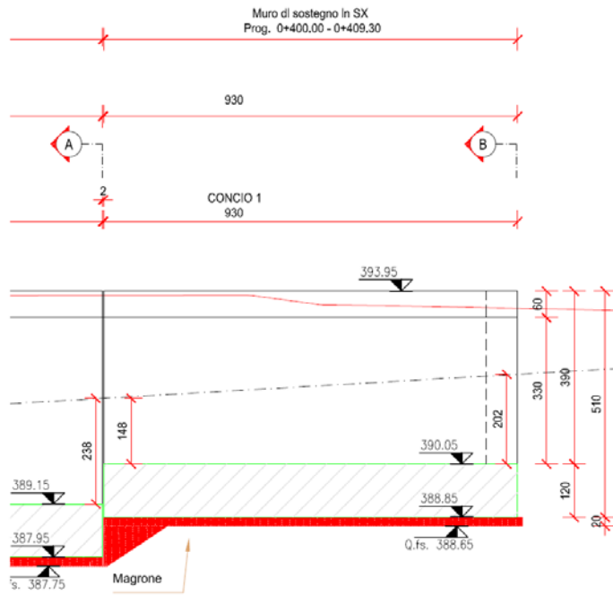
Fig. 2 Sezione longitudinale
