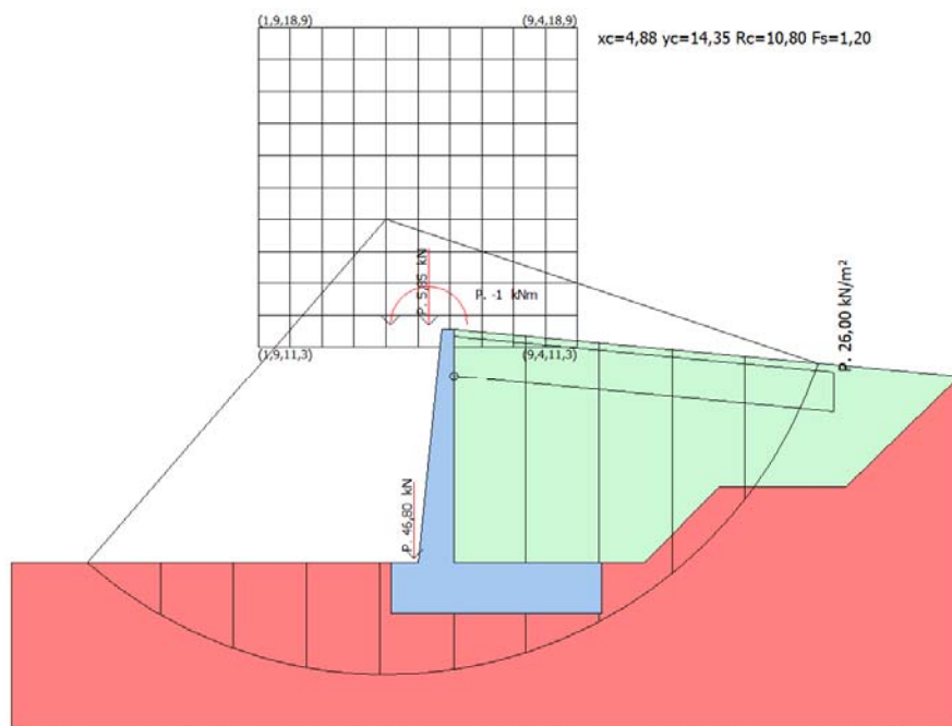
Fig. 8c Modello di calcolo concio 6
