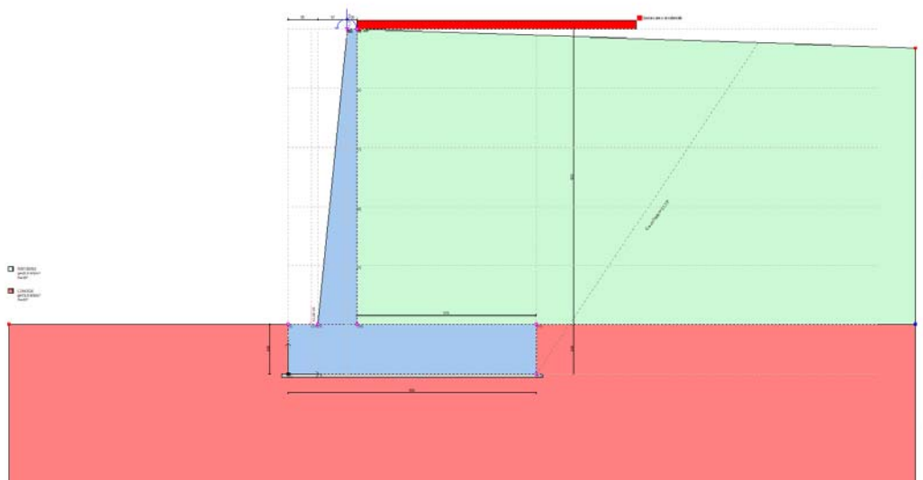
Fig. 7a Modello di calcolo concio 1
