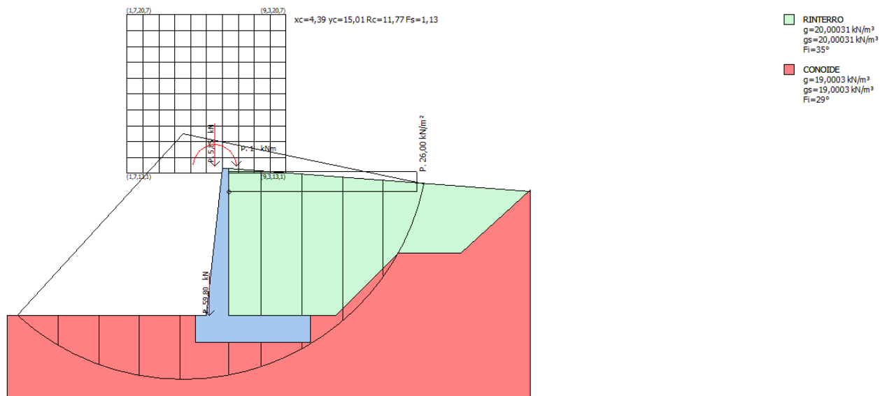
Fig. 8b Modello di calcolo concio 4
