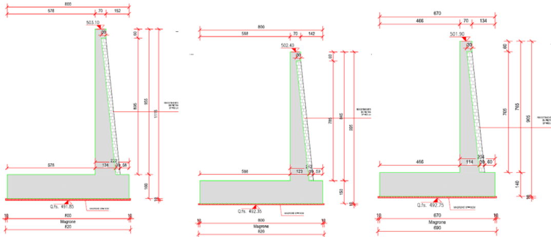
Fig. 1 Sezioni trasversali: inizio concio 1 – inizio concio 2 – concio 3
