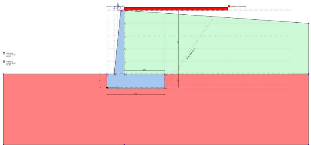
Fig. 7c Modello di calcolo concio 6
