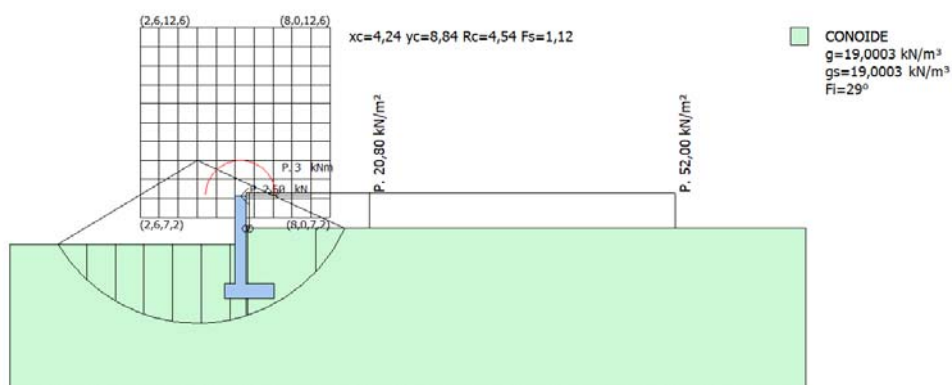
Fig. 7b Modello di calcolo per analisi di stabilità
