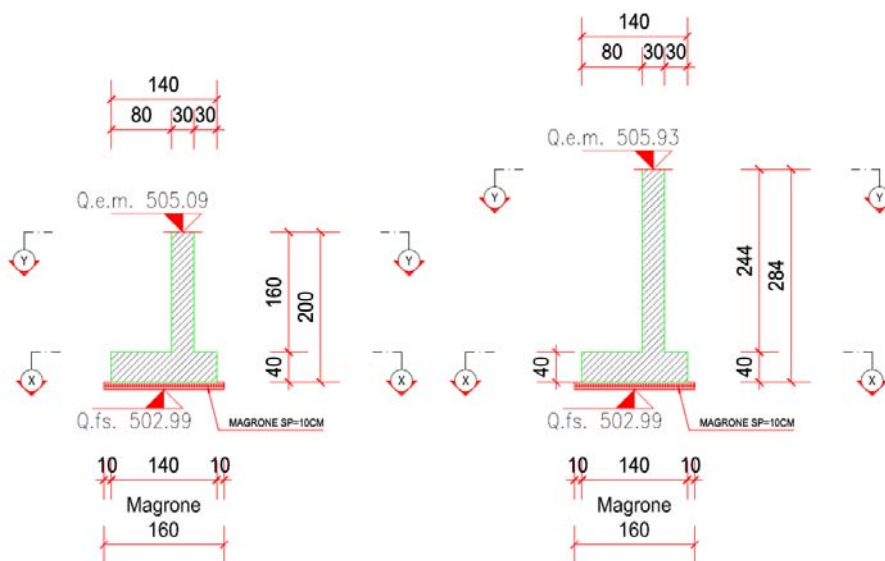
Fig. 1 Sezione longitudinale
