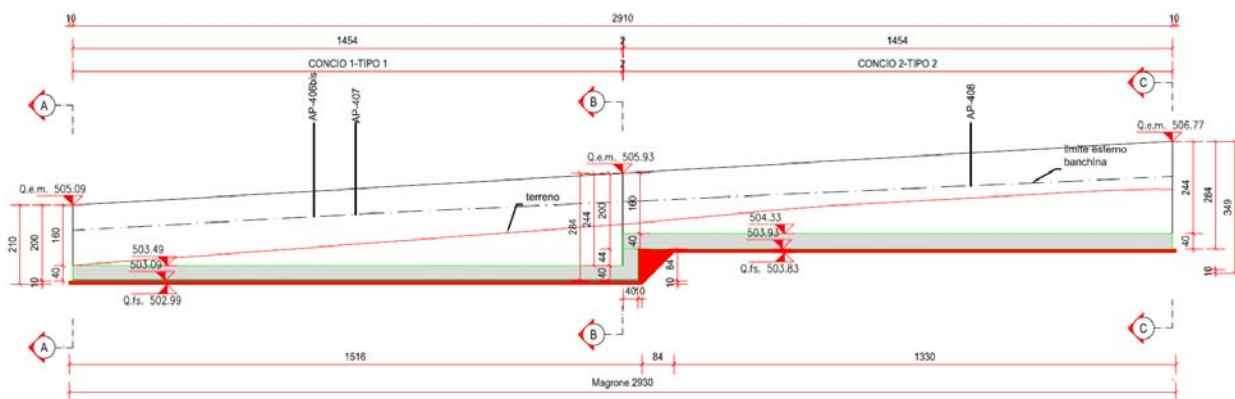
Fig. 1 Sezione longitudinale
