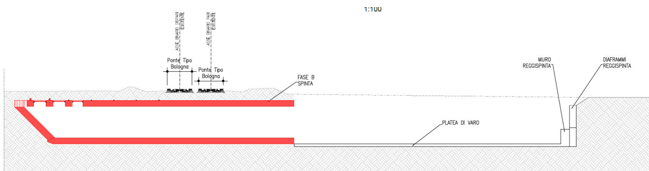
Figura 12 Fase di varo monolite
