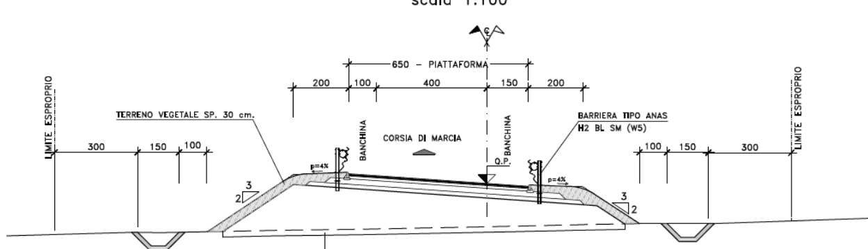
Figura 3.2 Sezione tipo Rampa di svincolo unidirezionale
