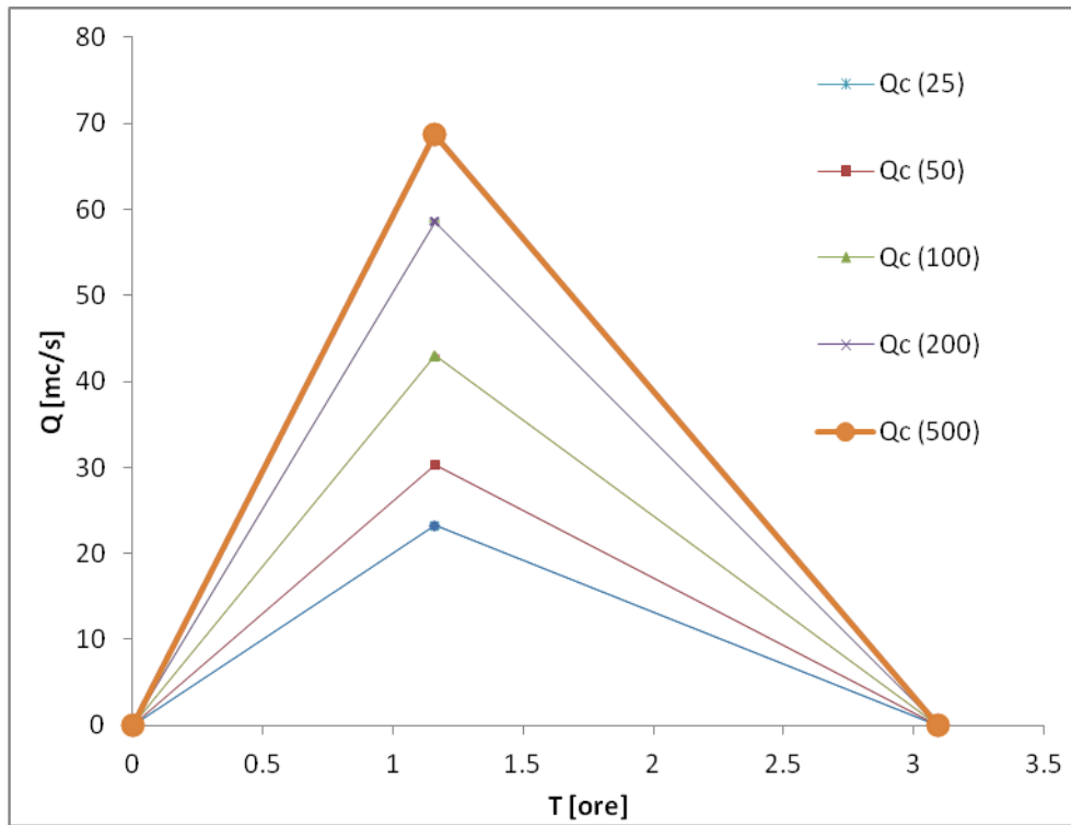
Figura 7.6 Idrogramma di piena Torrente Solera
