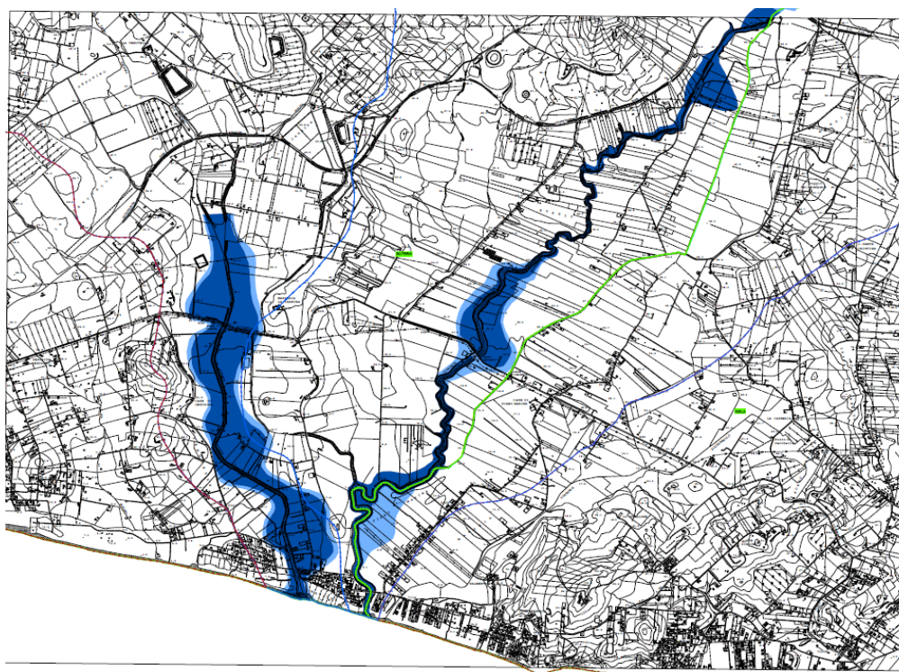
Figura 3.1.2: Carta pericolosità idraulica Torrente Comunelli.
