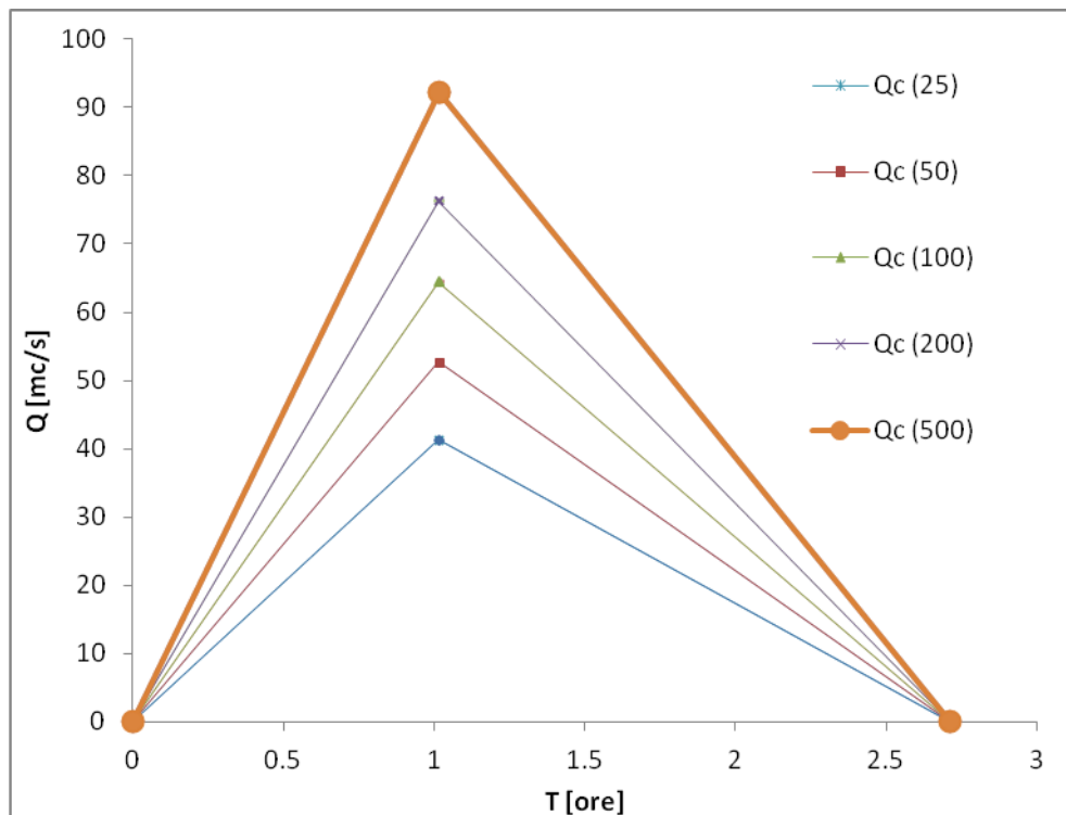
Figura 7.3 Idrogramma di piena Torrente Comunelli EST
