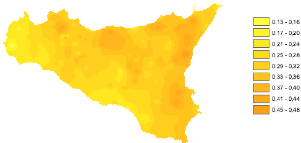
Figura.6.3.3 – Carta dei valori di "n" da PAI
