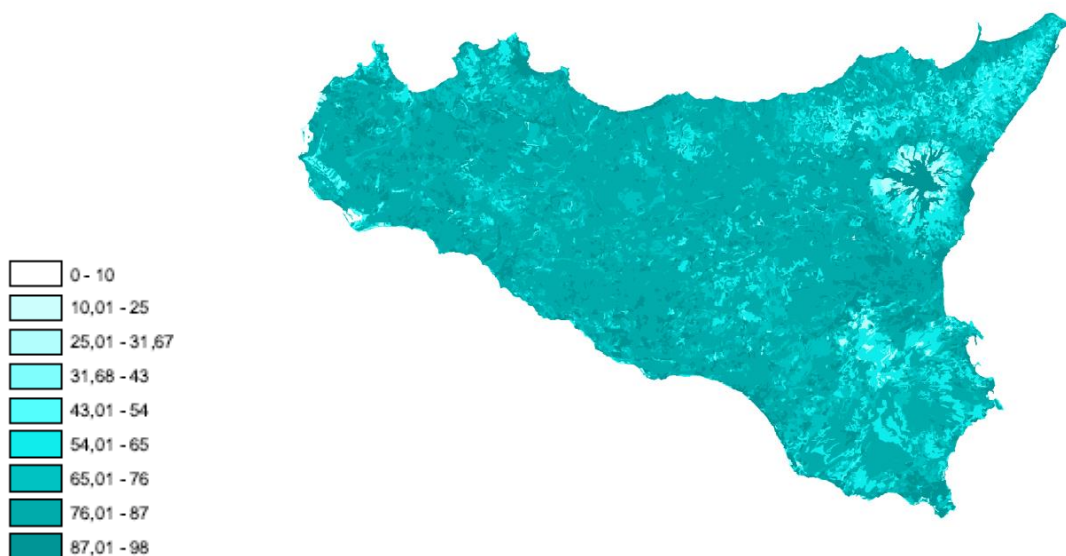
Figura:5.5.1 – Carta Valori di CN da PAI
