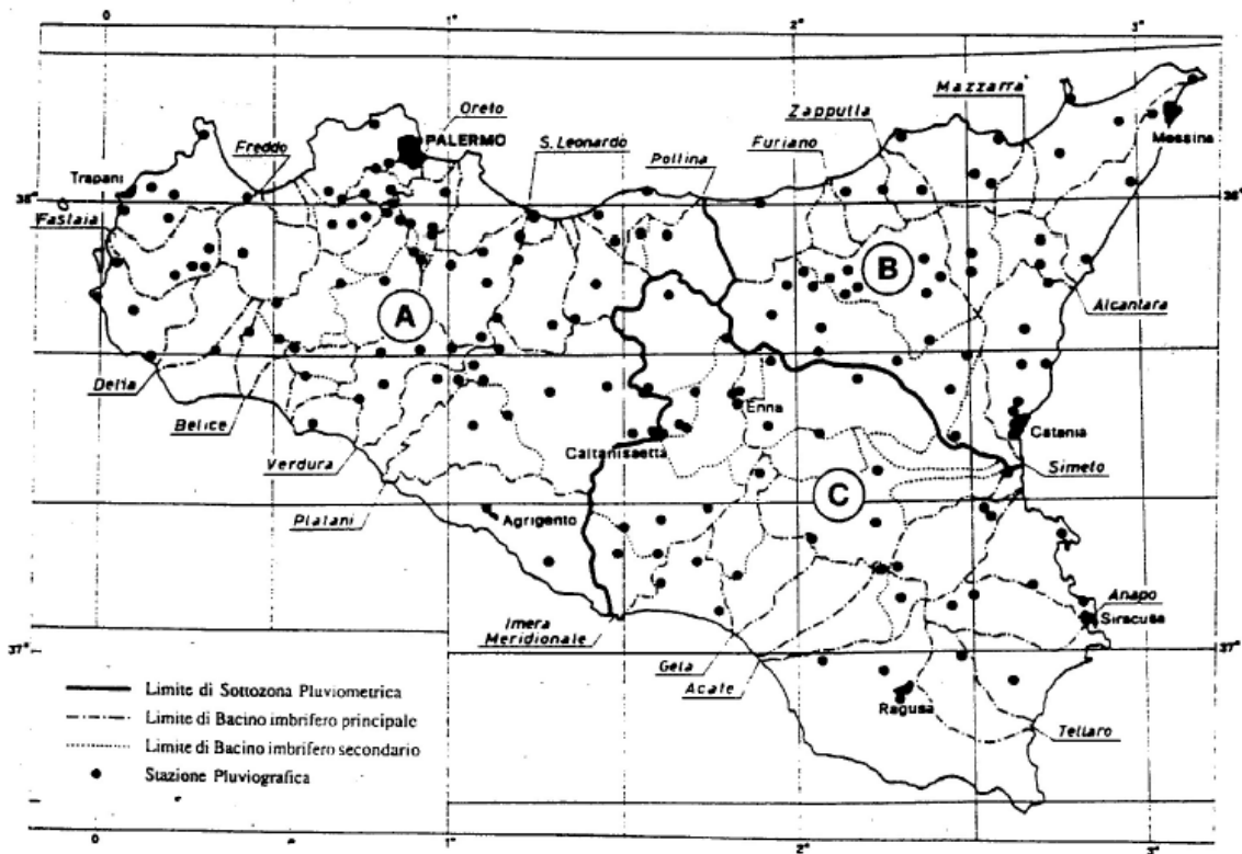
Figura 6.3.1 – Sottozone Omogenee Regione Sicilia
