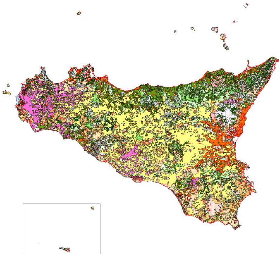
Figura.5.4.1 – Carta Uso Suolo PAI
