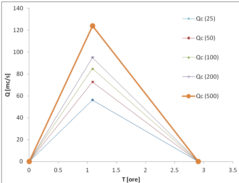
Figura 7.4 Idrogramma di piena Torrente Roccazzelle
