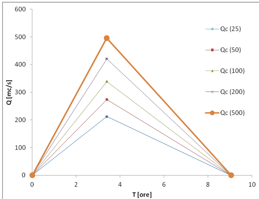
Figura 7.2 Idrogramma di piena Torrente Comunelli
