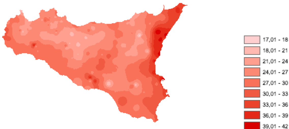
Figura 6.3.2 – Carta dei valori di "a" da PAI
