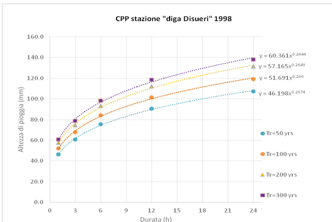
Figura: 5.2.5 – CPP stazione diga Disueri dati fino al 1998
