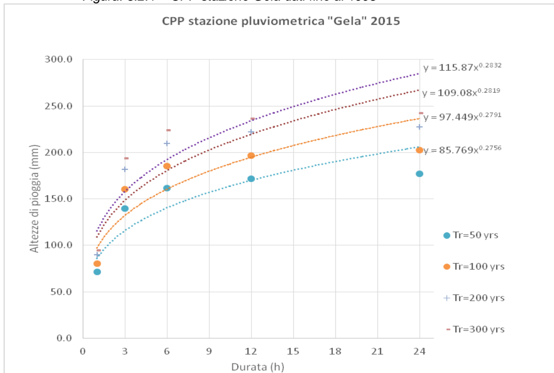
Figura: 5.2.2 – CPP stazione Gela dati aggiornati al 2015
