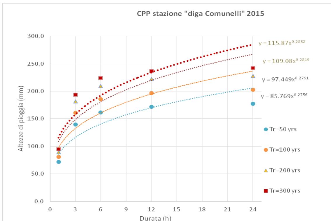
Figura: 5.2.4– CPP stazione diga Comunelli dati fino al 2015
