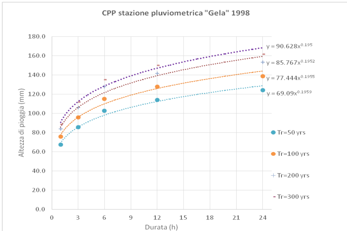
Figura: 5.2.1 – CPP stazione Gela dati fino al 1998
