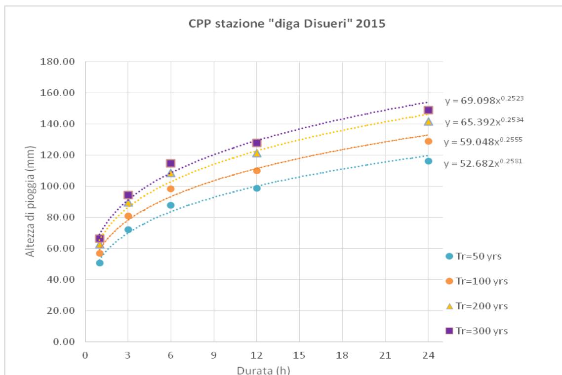
Figura: 5.2.6 – CPP stazione diga Disueri dati fino al 2015
