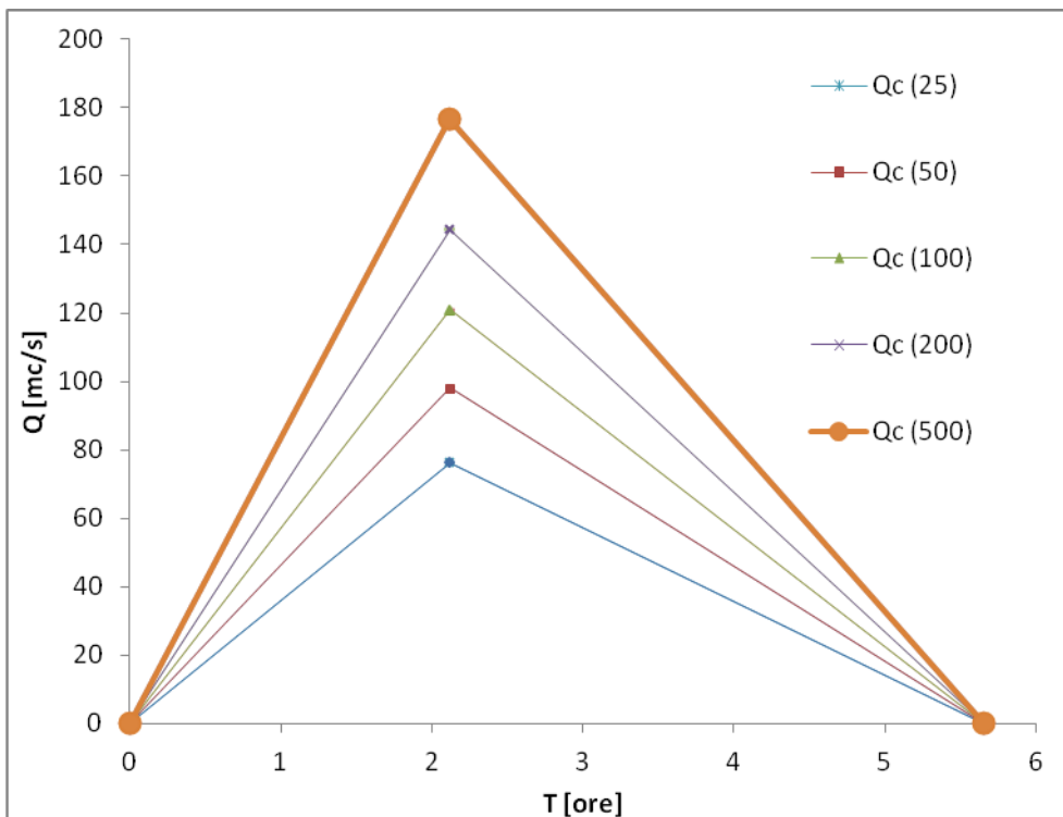
Figura 7.5 Idrogramma di piena Torrente Bruca
