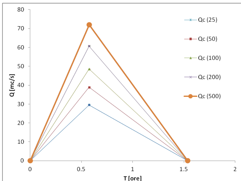
Figura 7.1 Idrogramma di piena Torrente Burgio
