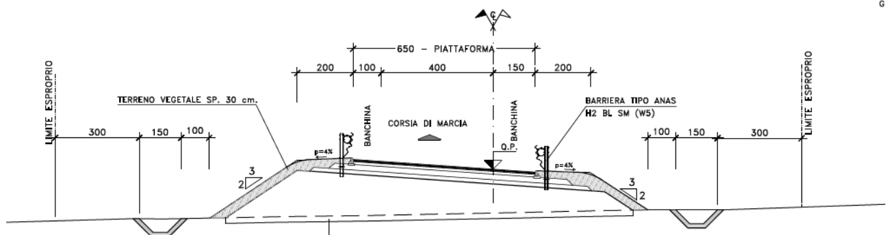
SEZIONE TIPO RAMPA DI SVINCOLO UNIDIREZIONALE TRATTO IN RILEVATO scala 1:100
