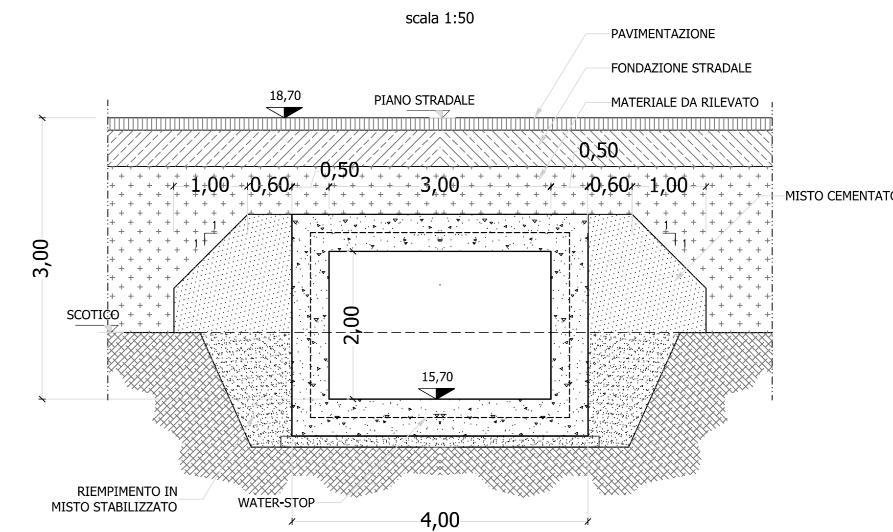
SEZIONE C-C
