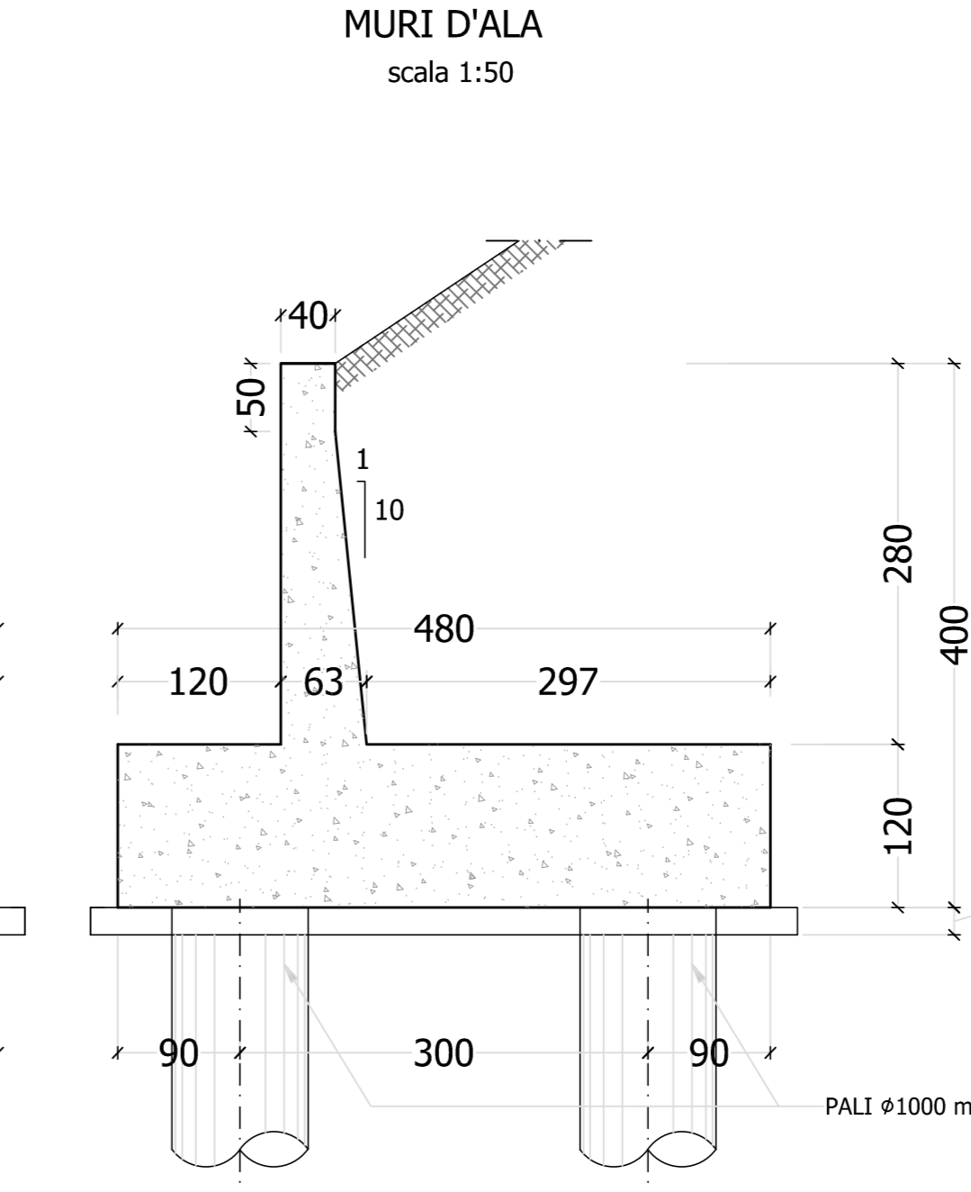
SEZIONE F-F
