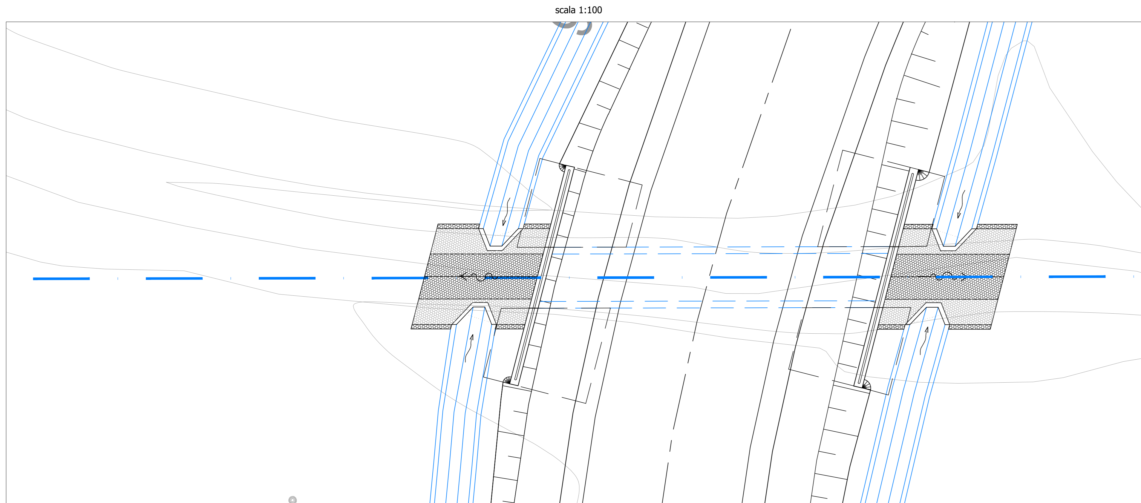
TOMBINO TM_SV02_AB_01 SCATOLARE 3x2 - pk 0+070.00 - PIANTA
