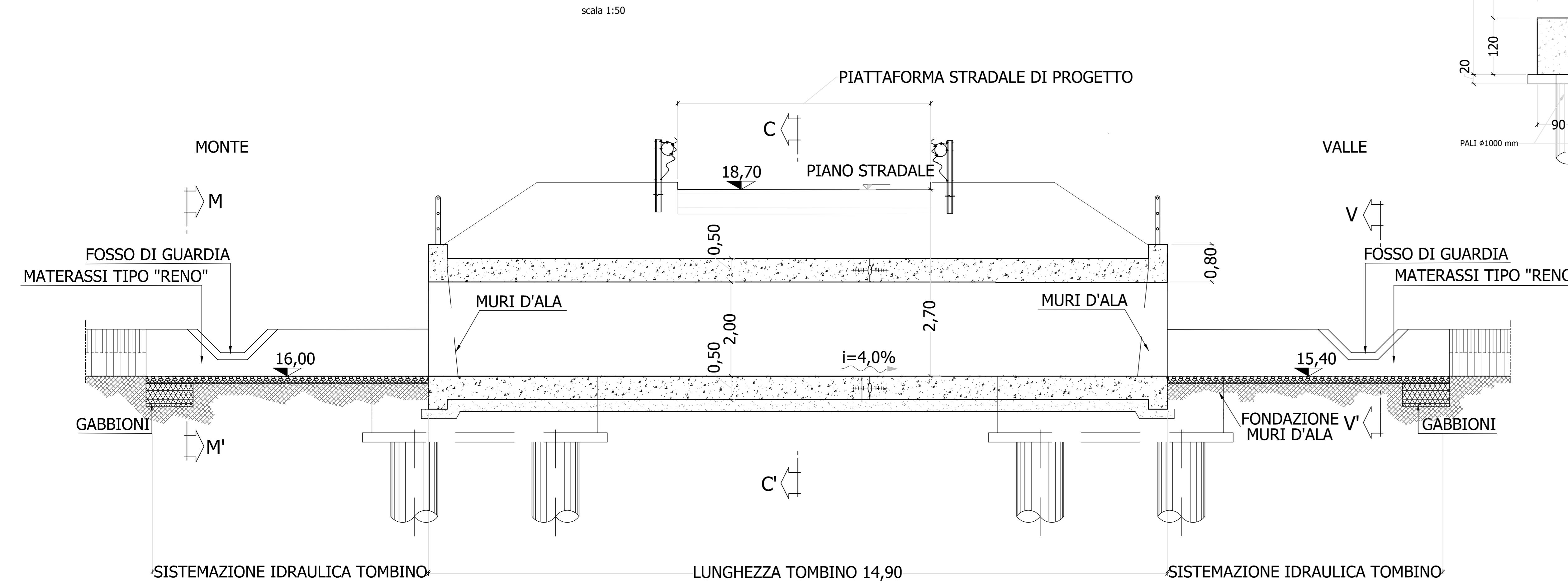
TOMBINO TM_SV02_AB_01 SCATOLARE 3x2 - pk 0+070.00 - SEZIONE LONGITUDINALE
