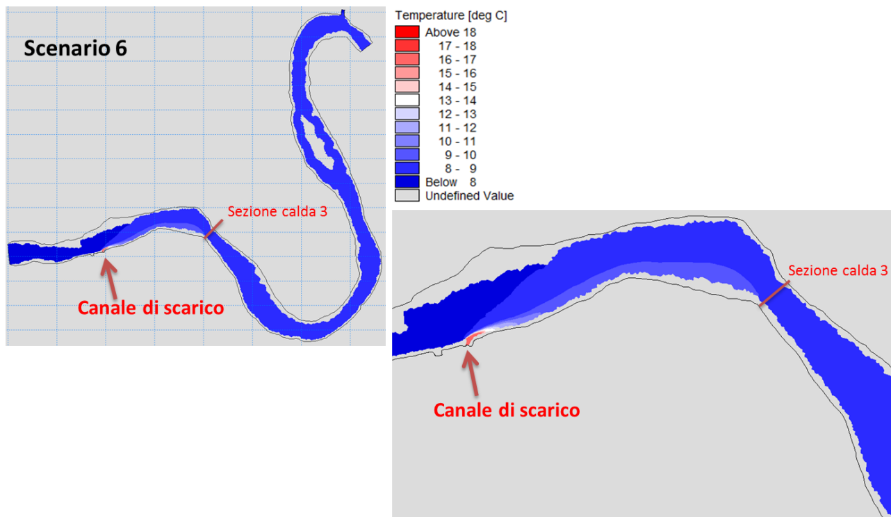
Figura 20 Campo termico calcolato per lo Scenario 6
