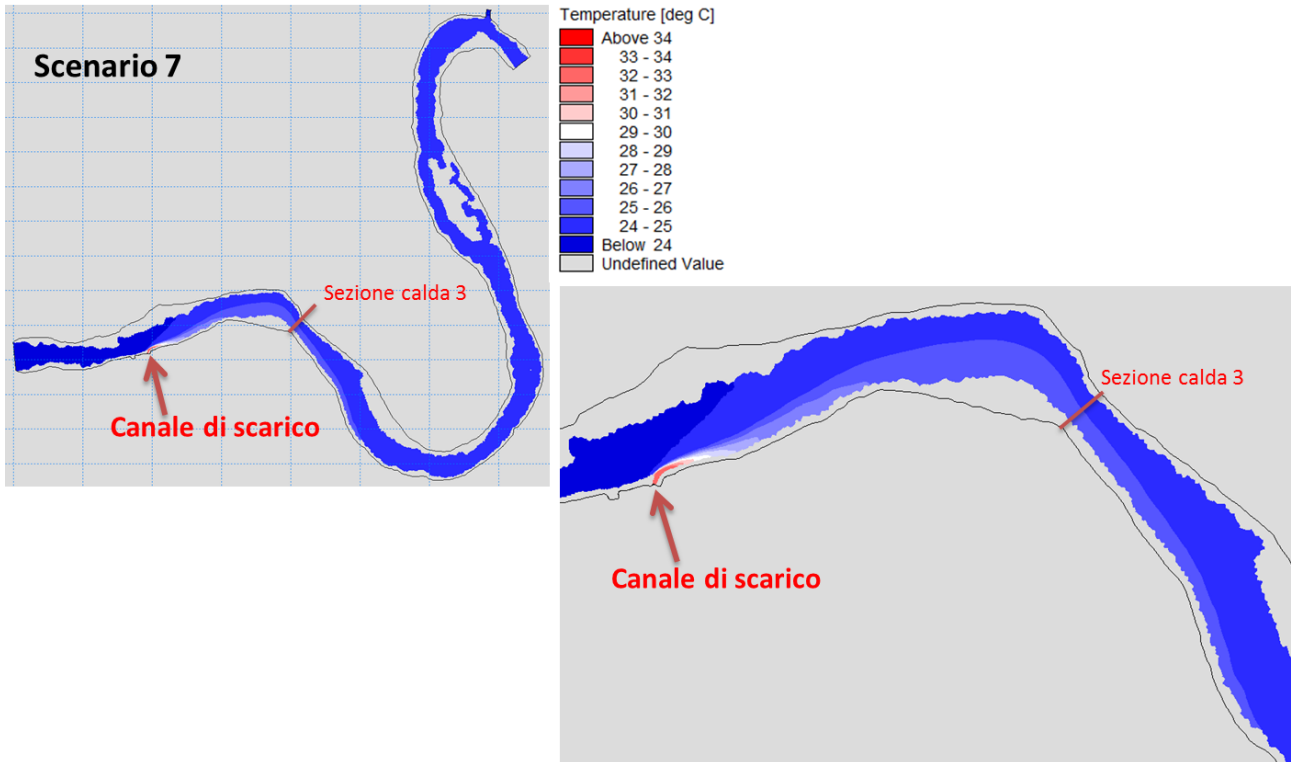
Figura 21 Campo termico calcolato per lo Scenario 7
