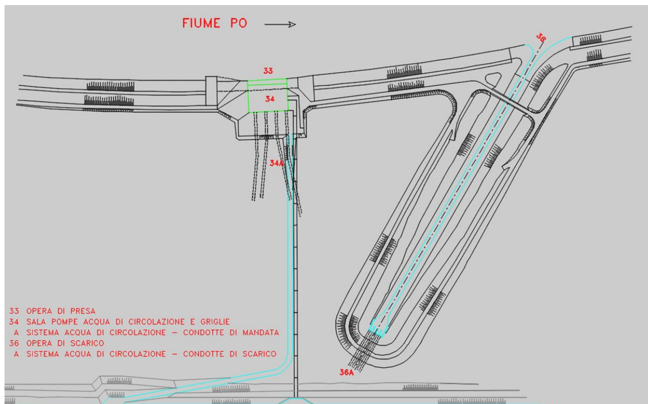
Figura 3 Localizzazione in pianta della presa e del canale di scarico delle acque di circolazione della centrale di La Casella (Rif. 2).
