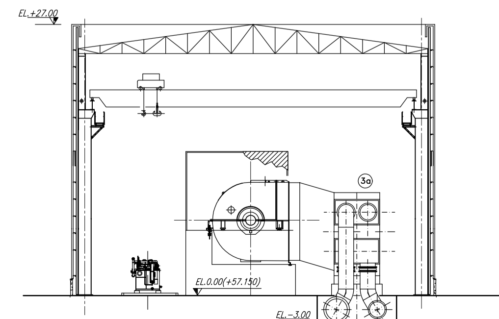
SEZIONE C-C SCALE 1:250
