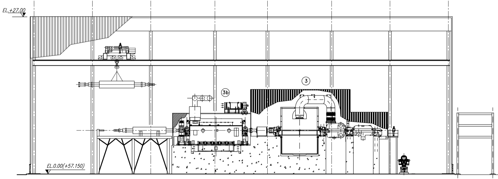
SEZIONE B-B SCALE 1:250
