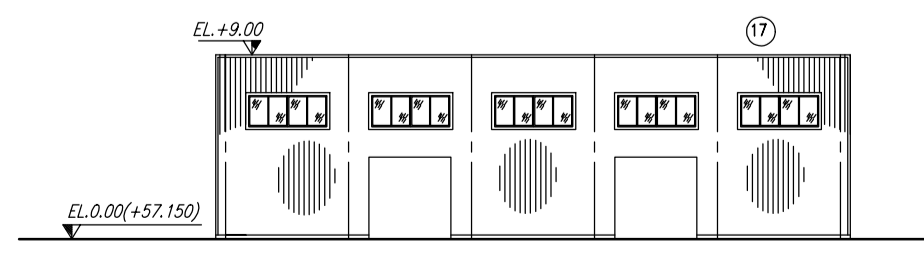
SEZIONE E-E SCALE 1:250
