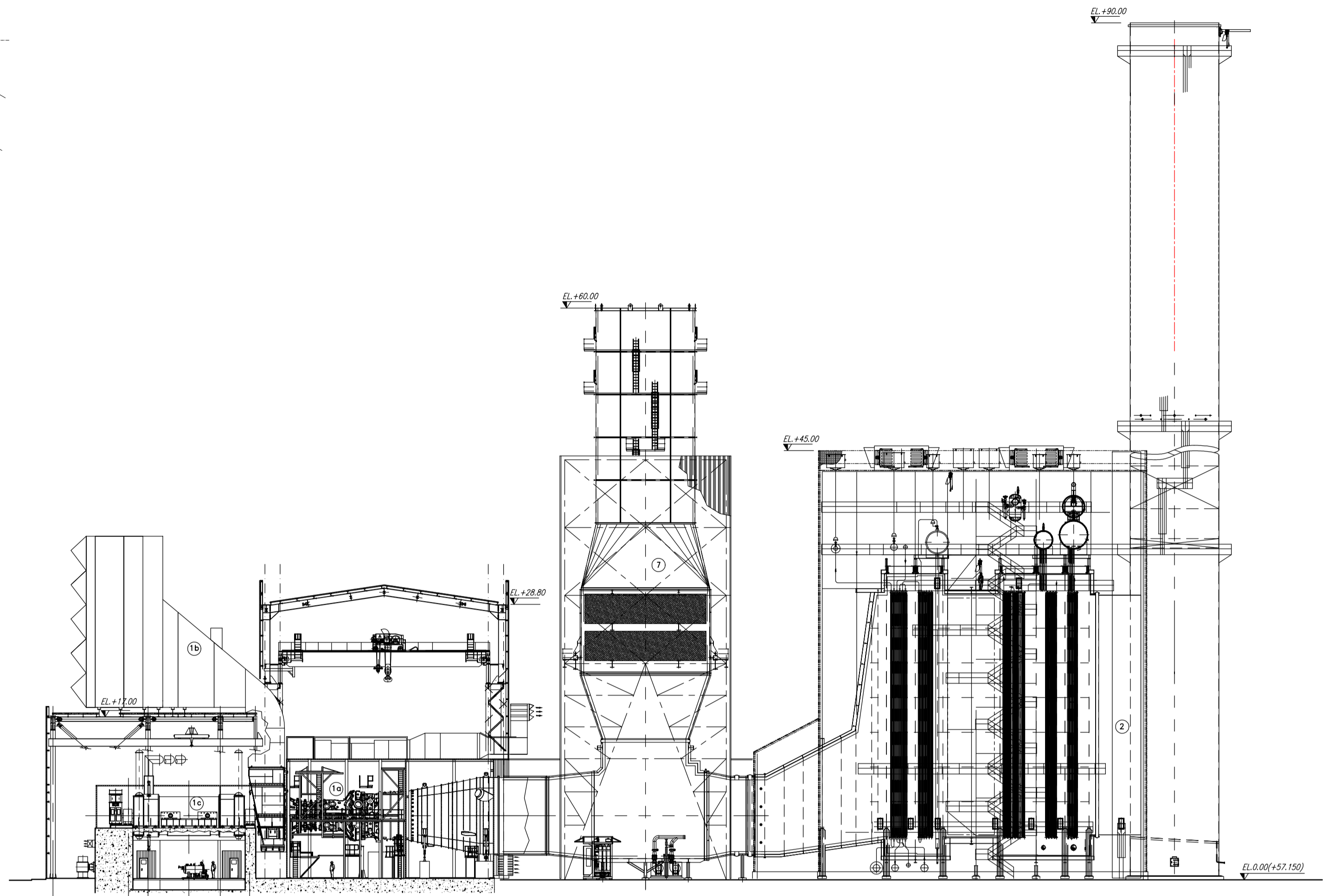
SEZIONE A-A SCALE 1:250
