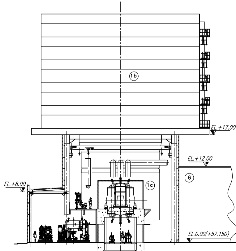
SEZIONE D-D SCALE 1:250
