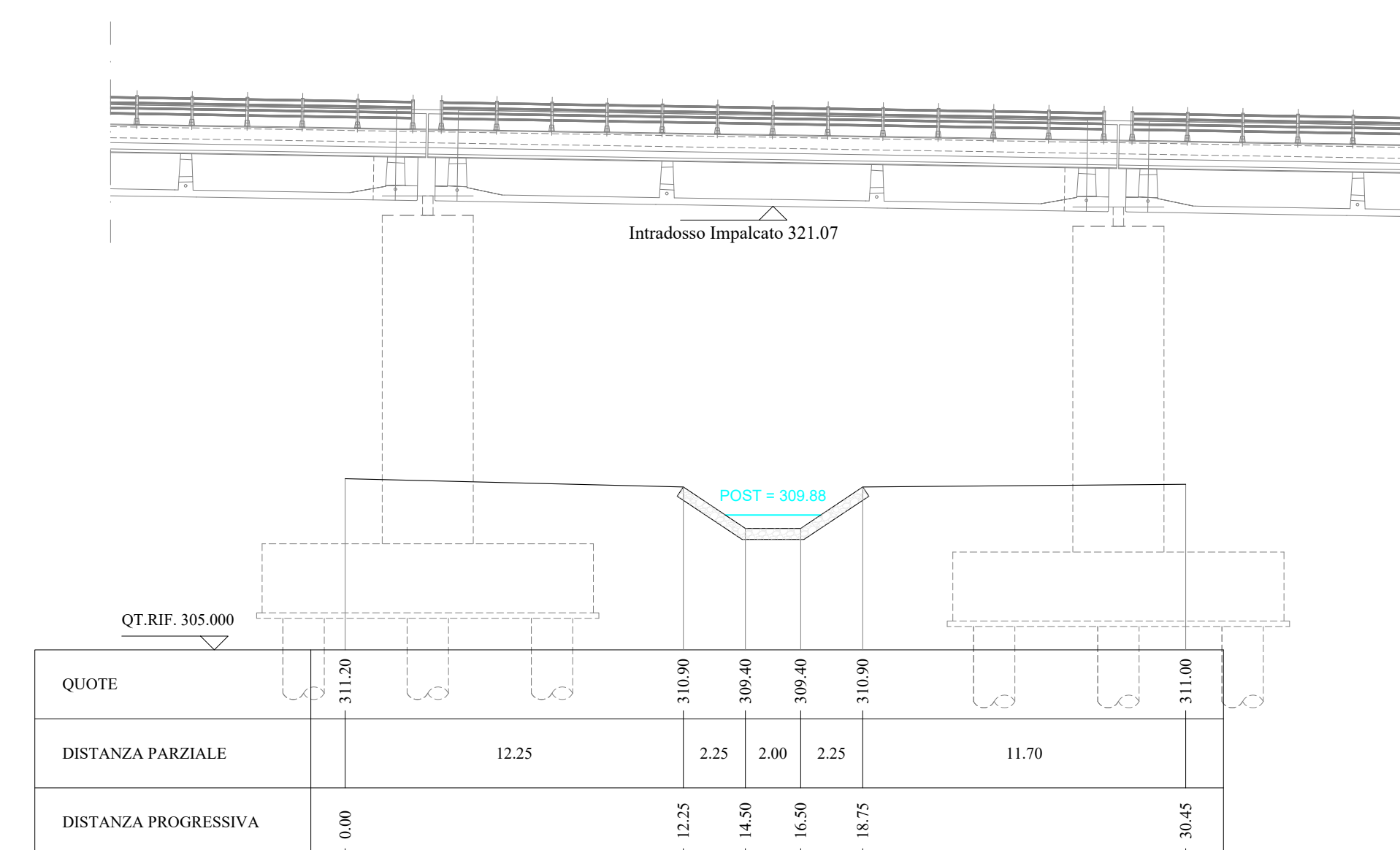
SEZIONE 155.623
