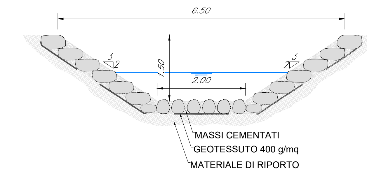
SISTEMAZIONE IDRAULICA SEZIONE TIPO 1
