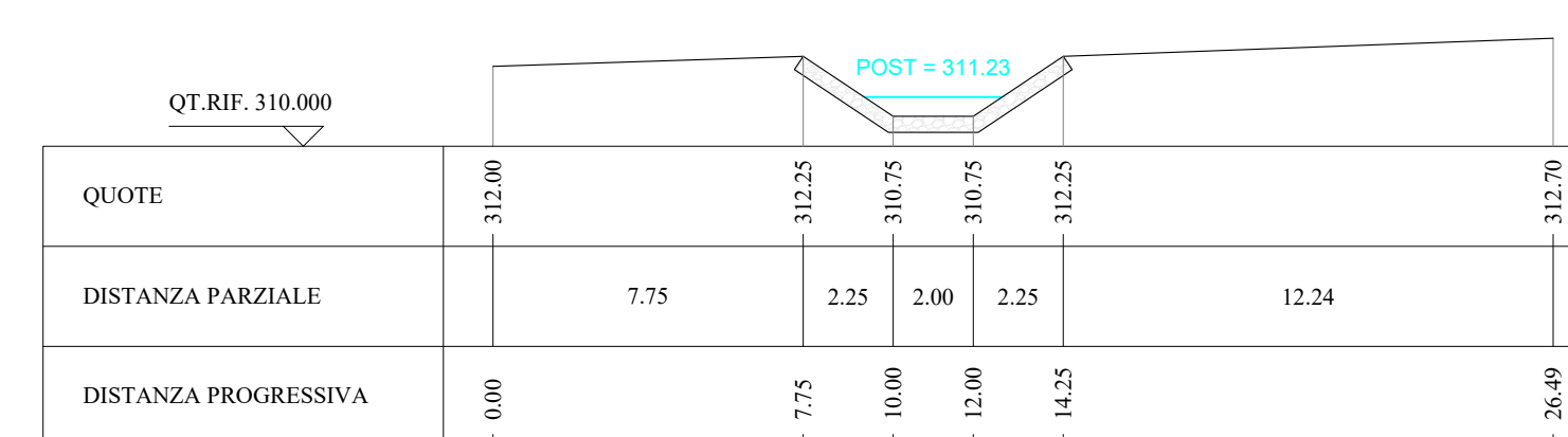
SEZIONE 155.623
