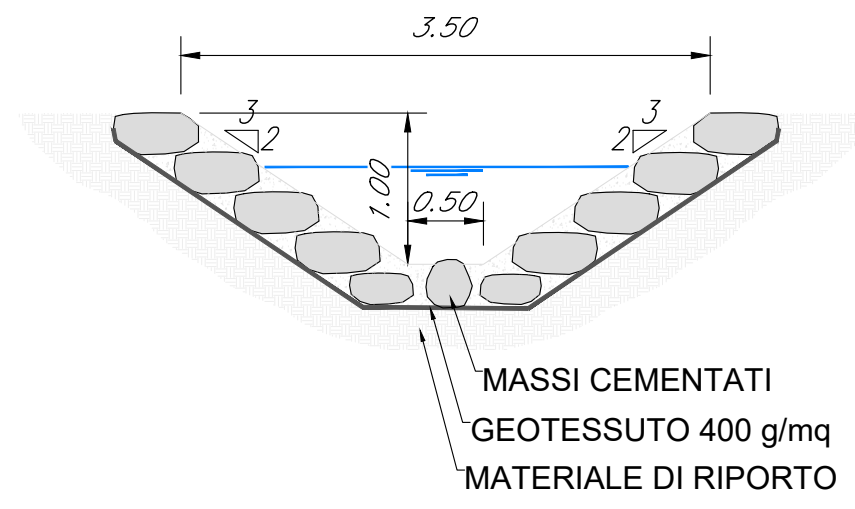
SISTEMAZIONE IDRAULICA SEZIONE TIPO 1 Scala 1:50
