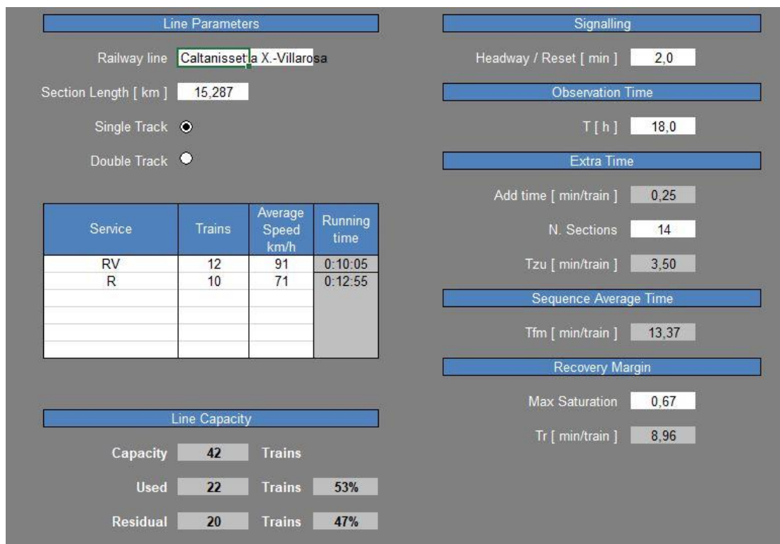
Figura 12: Calcolo capacità tratta a semplice binario tra Fiumetorto e Catenanuova.
