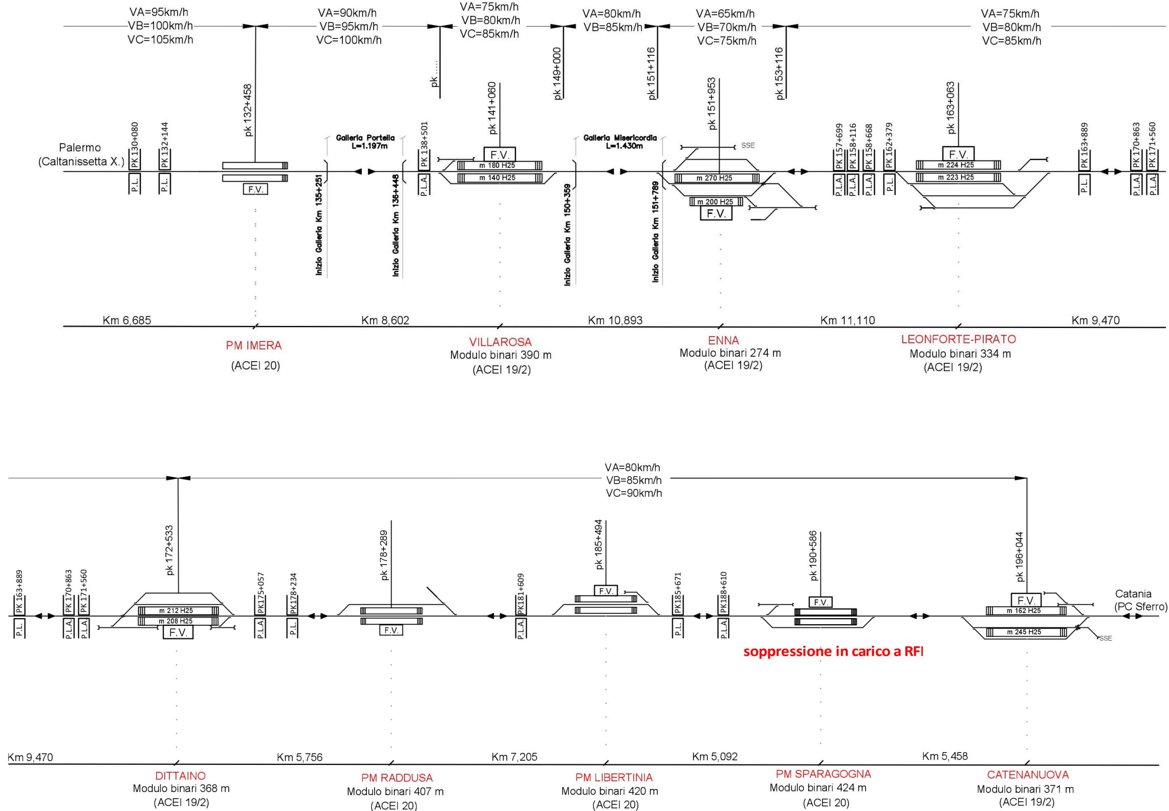
a 6: Layout funzionale della tratta Fiumetorto - Catenanuova. Scenario Attuale (3/3)
