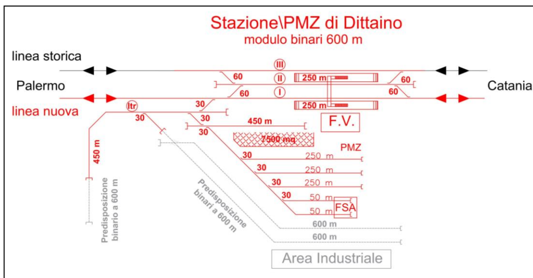
Figura 18: Layout funzionale di progetto – Stazione di Dittaino
