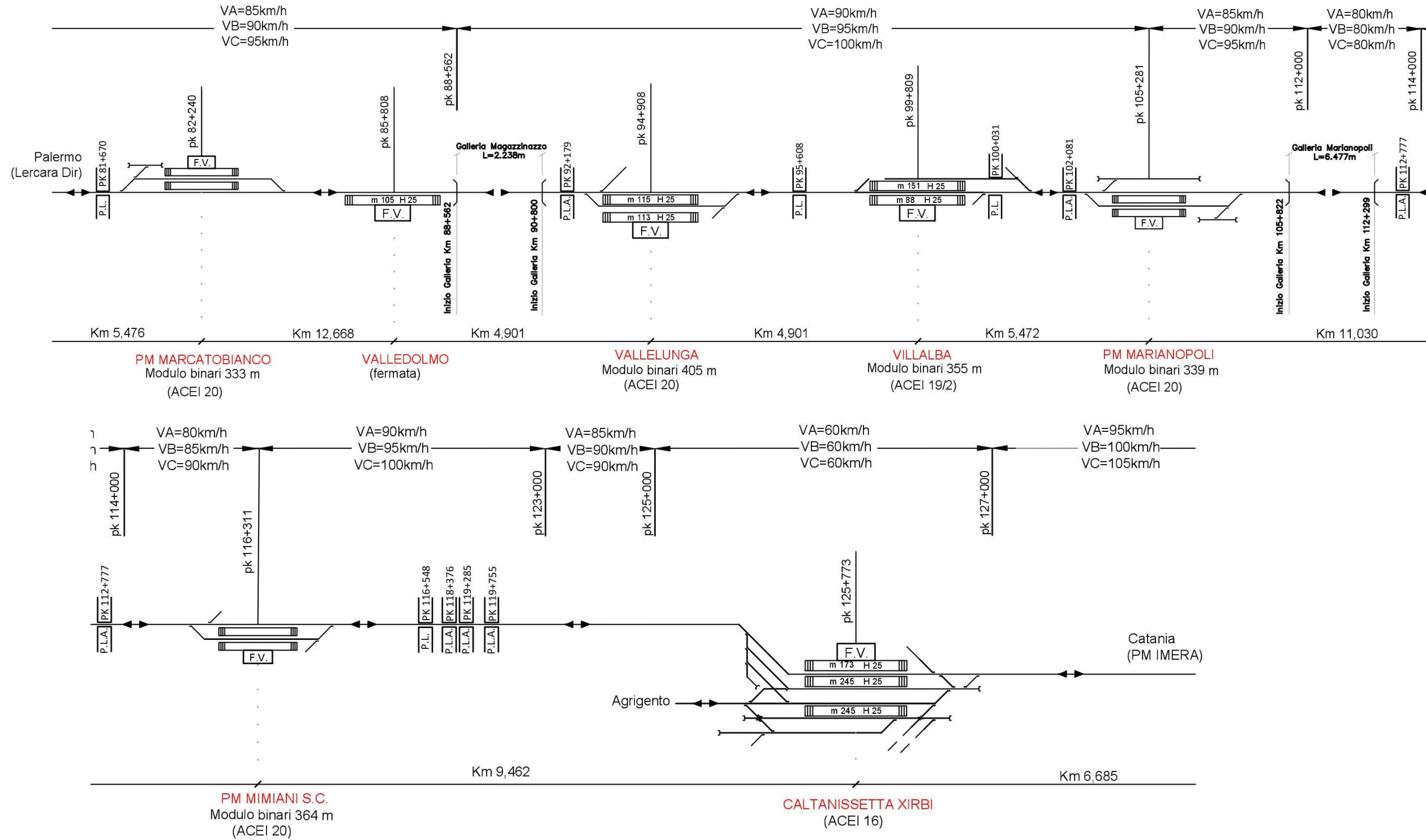
Figura 5: Layout funzionale della tratta Fiumetorto - Catenanuova. Scenario Attuale (2/3)
