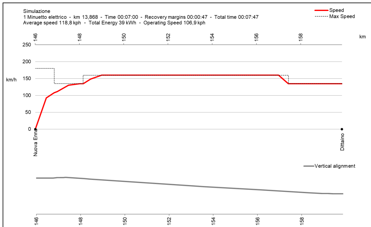
Figura 21: Diagramma di marcia Servizio Regionale Veloce Palermo–Catania della tratta Nuova Enna-Dittaino (Lotto 4B) come da scenario di progetto in Prima Macrofase Funzionale.
