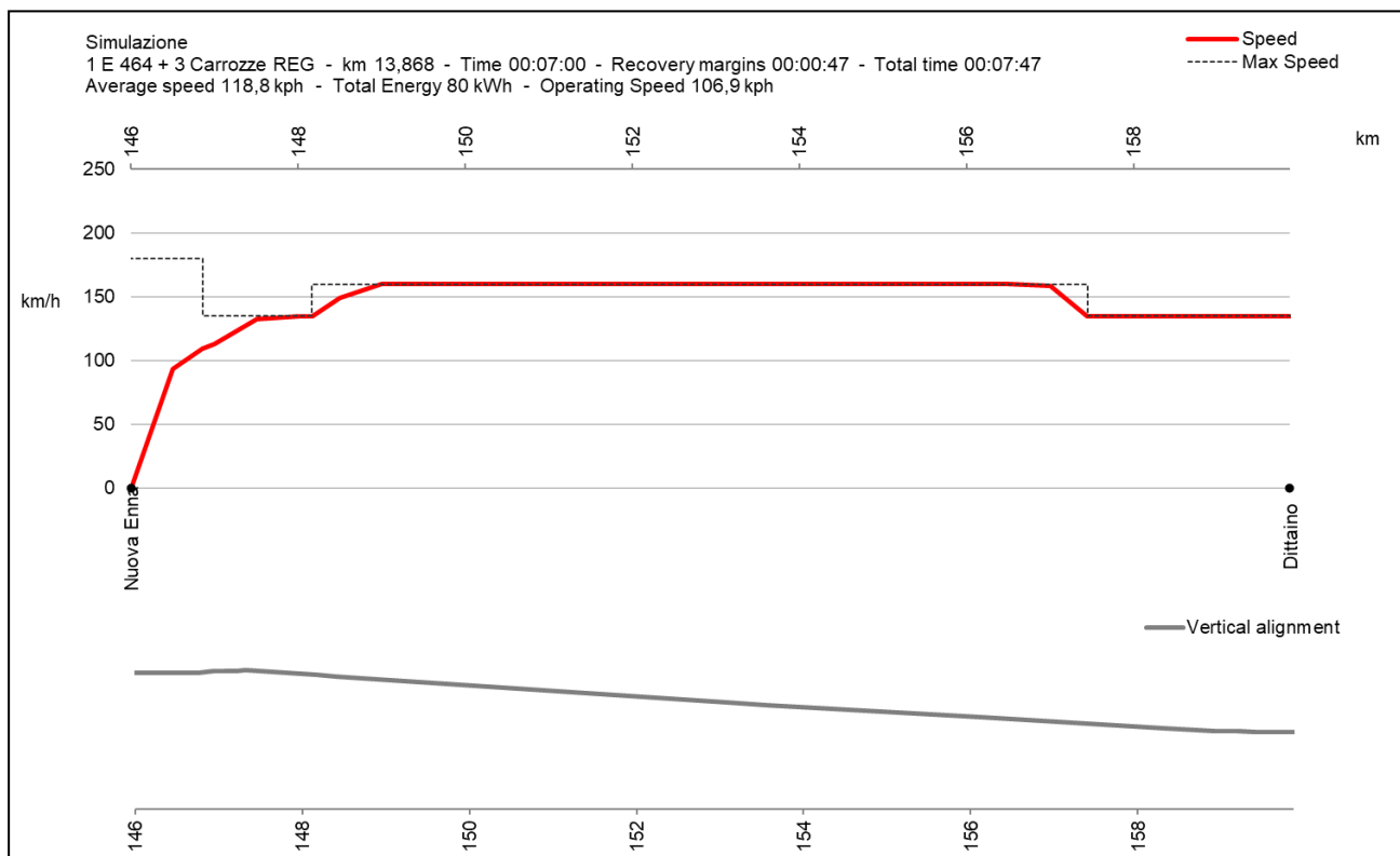
Figura 23: Diagramma di marcia Servizio Regionale Veloce Palermo – Catania della tratta tratta Nuova Enna-Dittaino (Lotto 4B) come da scenario di progetto in Prima Macrofase Funzionale
