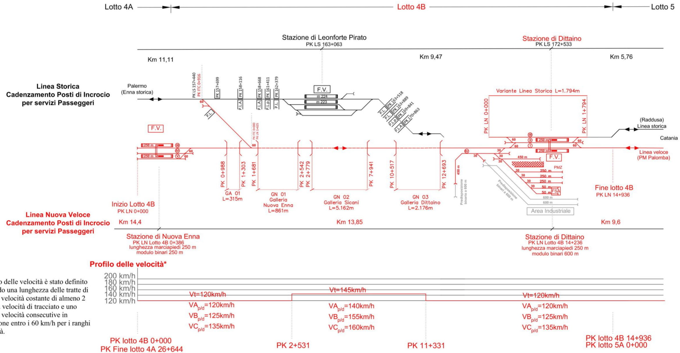
Figura 16: Layout funzionale di progetto del Lotto 4B Nuova Enna (i) – Dittaino (i)
