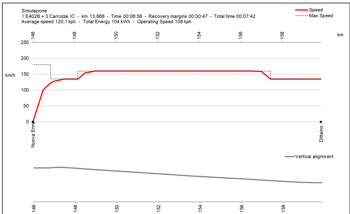
Figura 22: Diagramma di marcia Servizio Intercity Palermo – Catania della tratta Nuova Enna-Dittaino (Lotto 4B) come da scenario di progetto in Prima Macrofase Funzionale.
