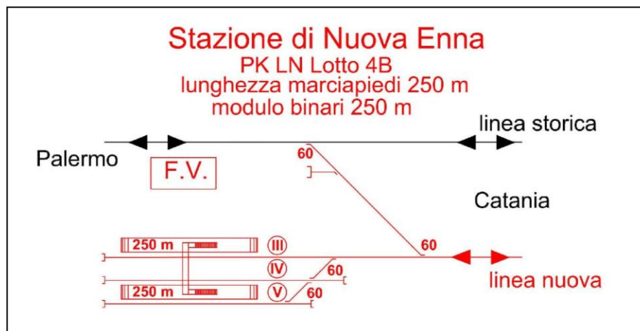
Figura 17: Layout funzionale di progetto – Stazione di Enna Lotto 4B
