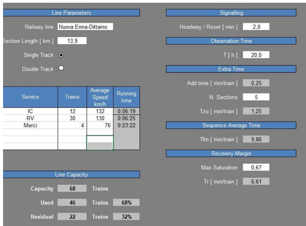
Figura 24: Calcolo capacità tratta a nuovo semplice binario tra Nuova Enna e Dittaino. Prima Macrofase Funzionale
