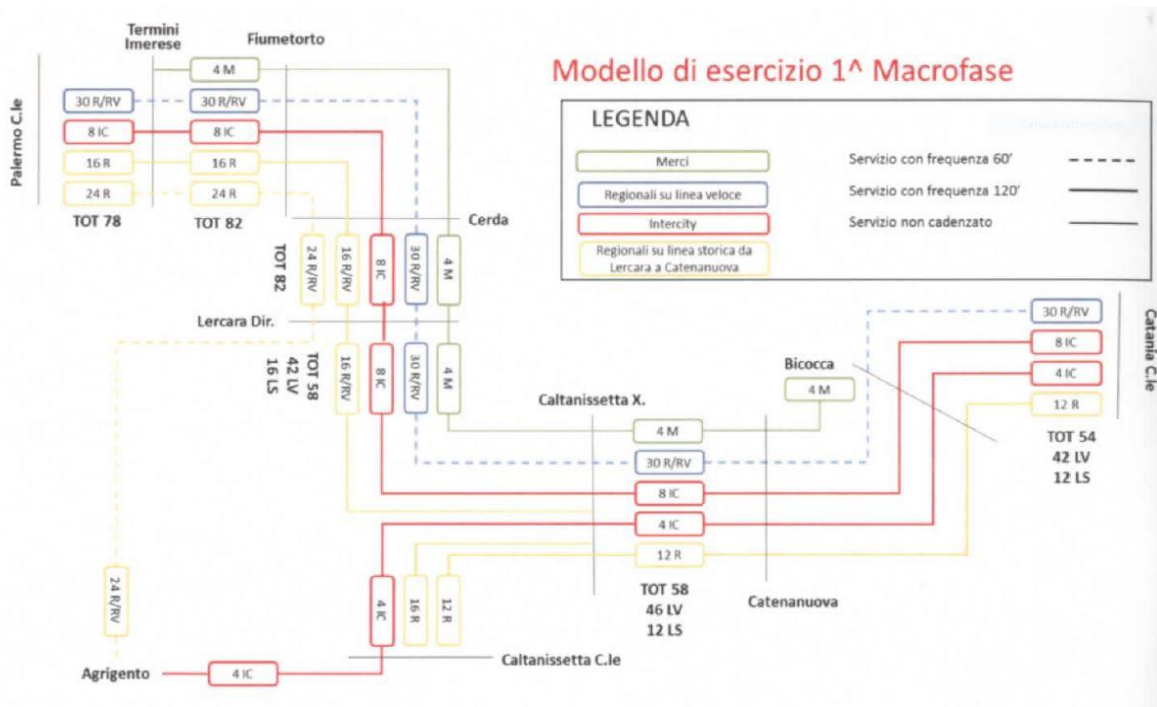
Figura 19: Modello di esercizio di 1° Macrofase. Ripartizione dei servizi tra linea nuova e linea storica
