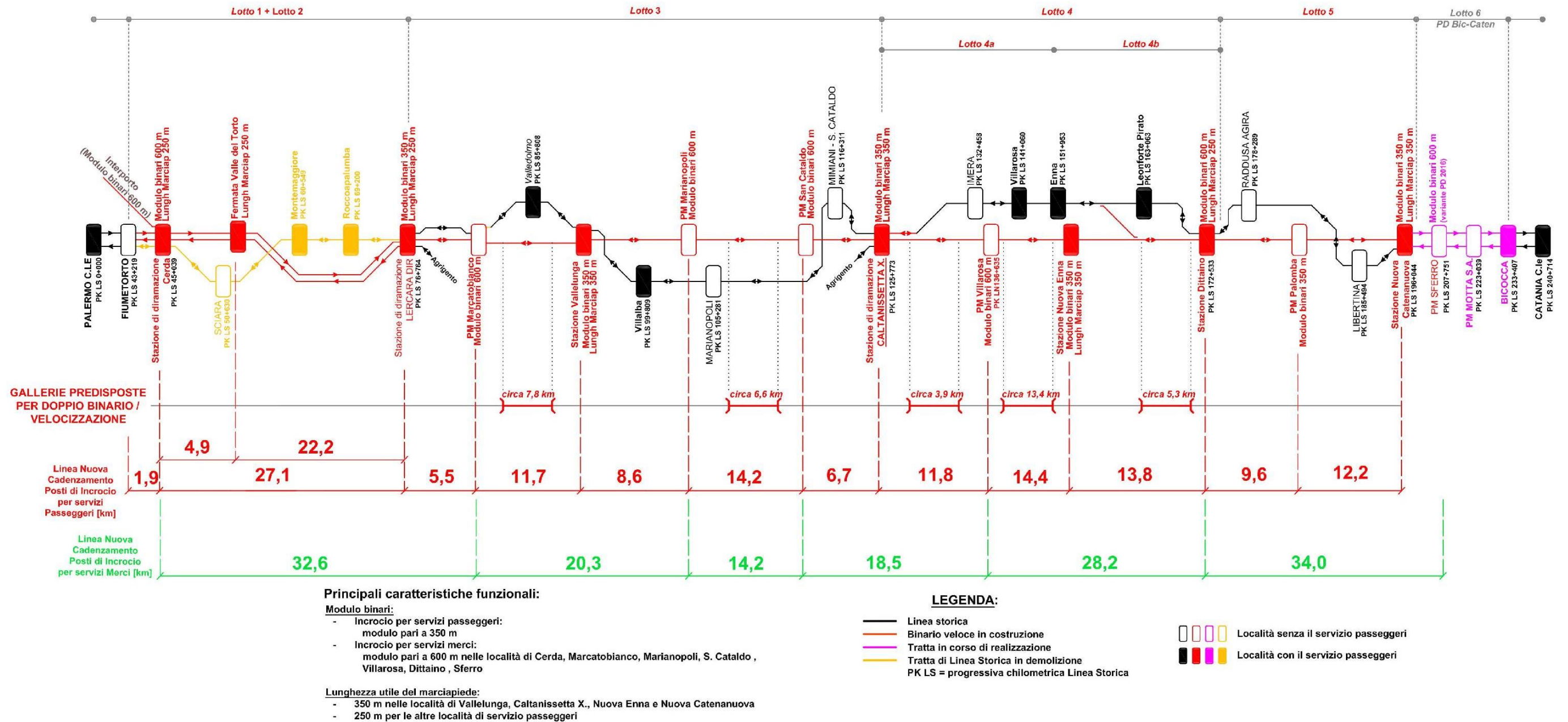
Figura 15 – Schema unifilare Palermo – Catania. 1° Macrofase funzionale.
