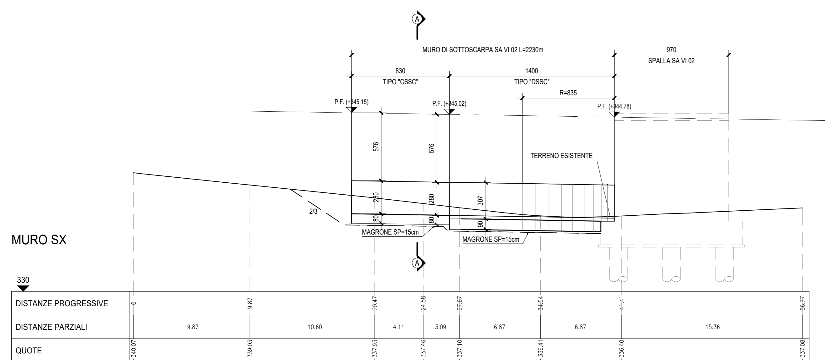
PROFILO LONGITUDINALE MURO SX SPALLA SA VI 02 - Scala 1:200
