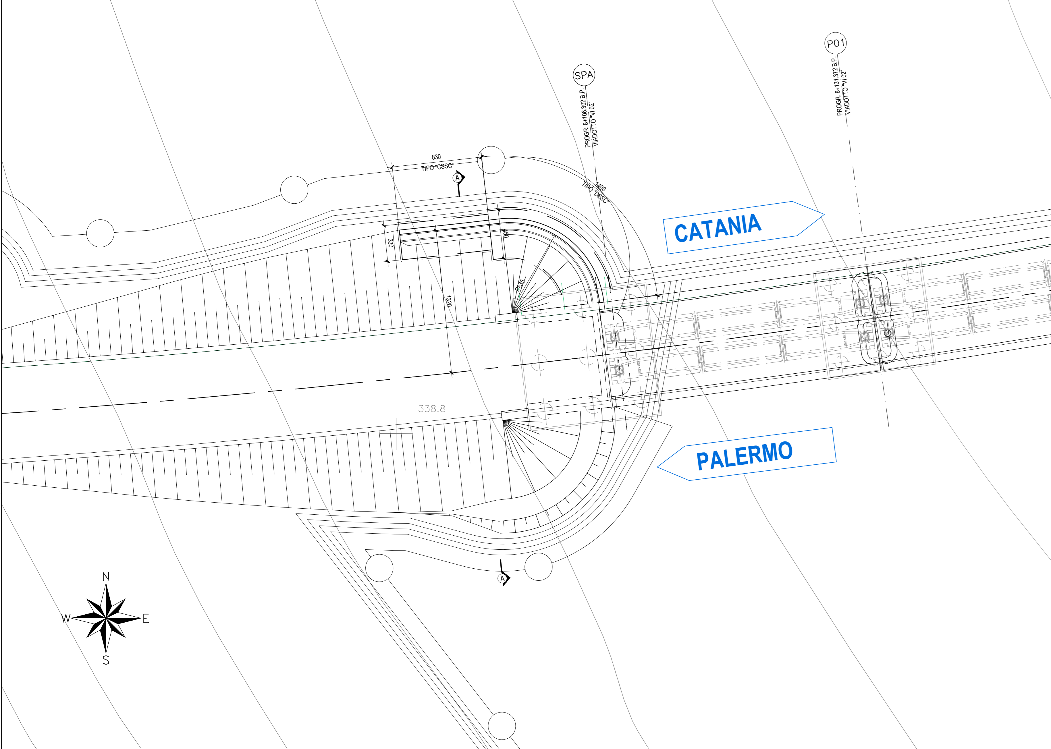
PIANTA MURO SX SPALLA SA VI 02 - Scala 1:200
