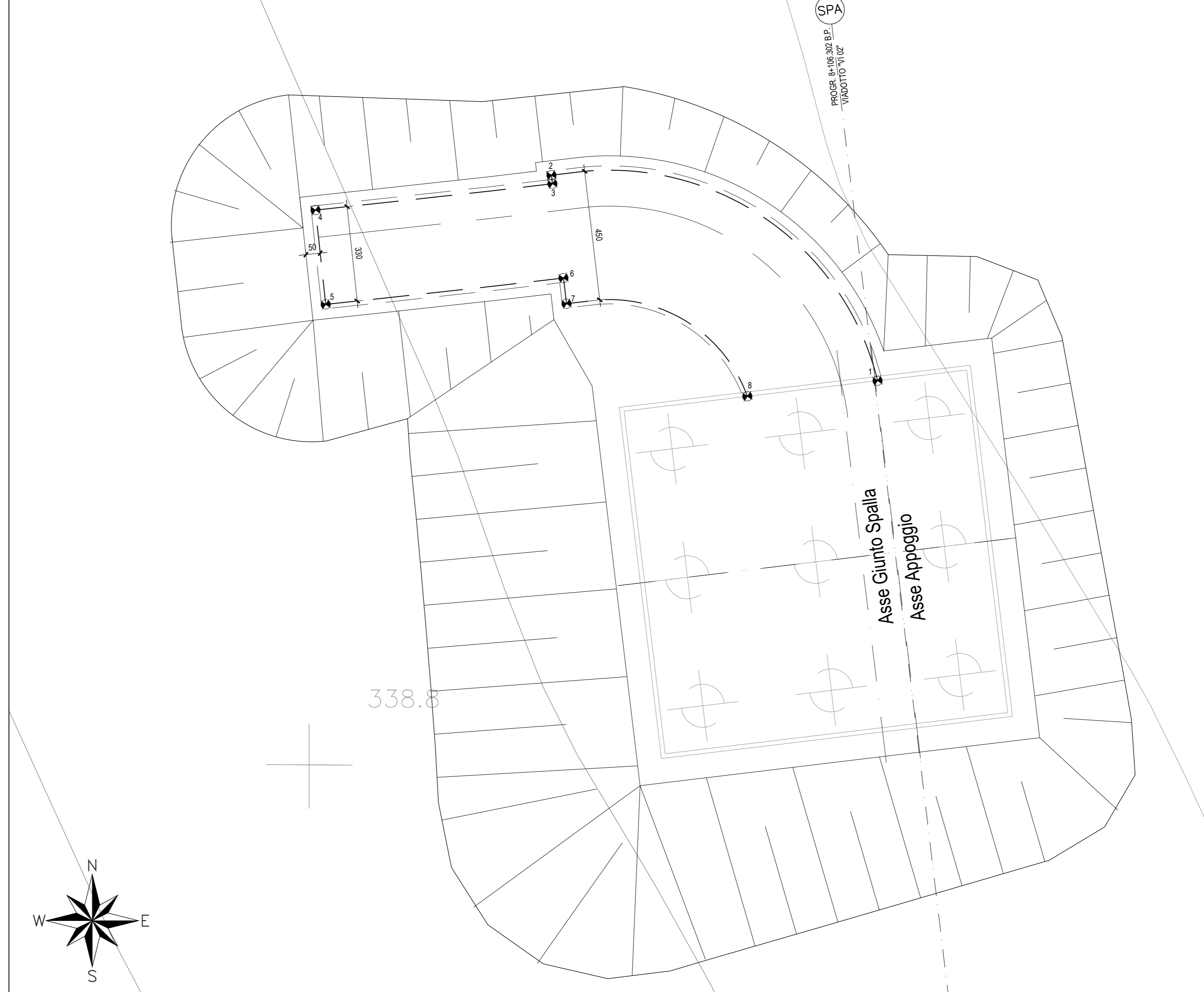
PIANTA SCAVI - Scala 1:100
