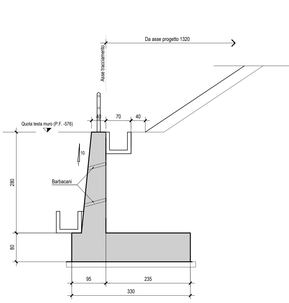
Tipo "Cssc"- 2.00 < H < 3.00
