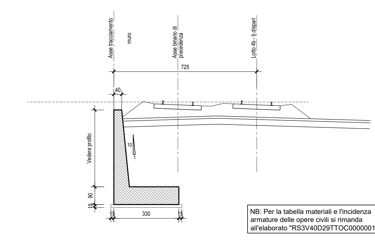
SEZIONE TIPO-Scala 1:100
