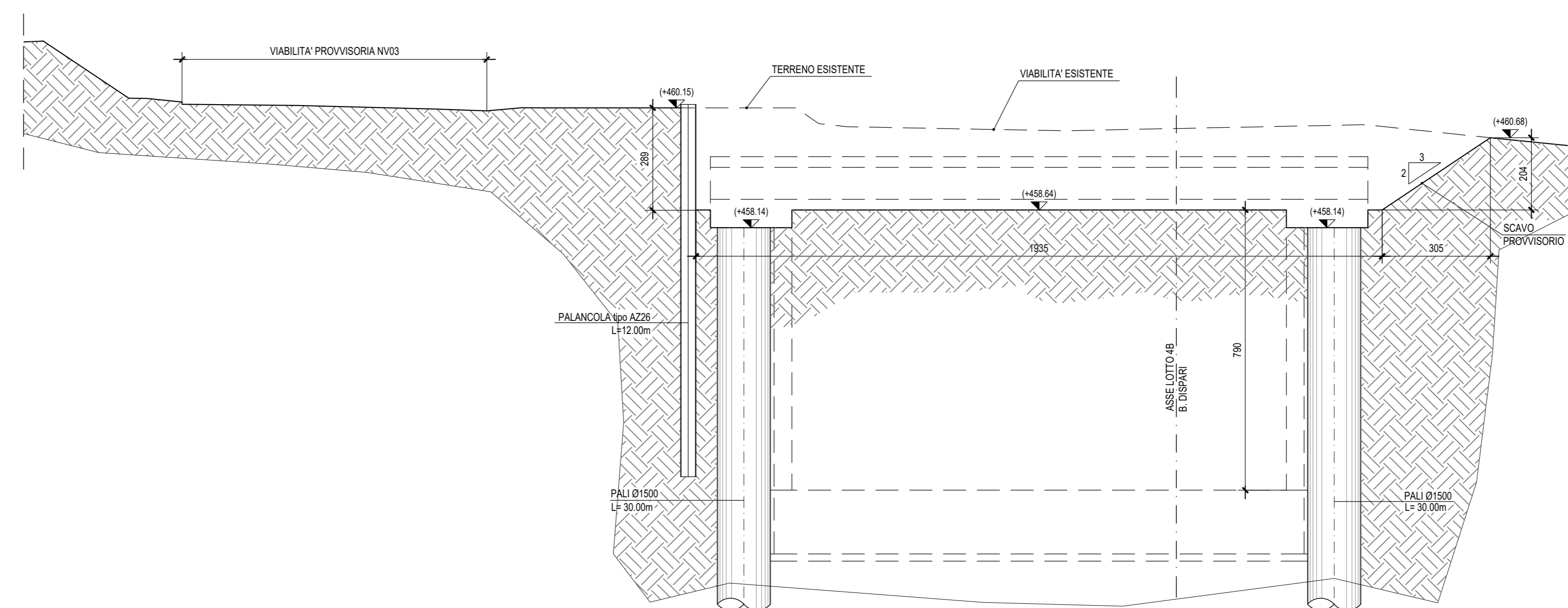
SEZIONE D-D - Scala 1:100
