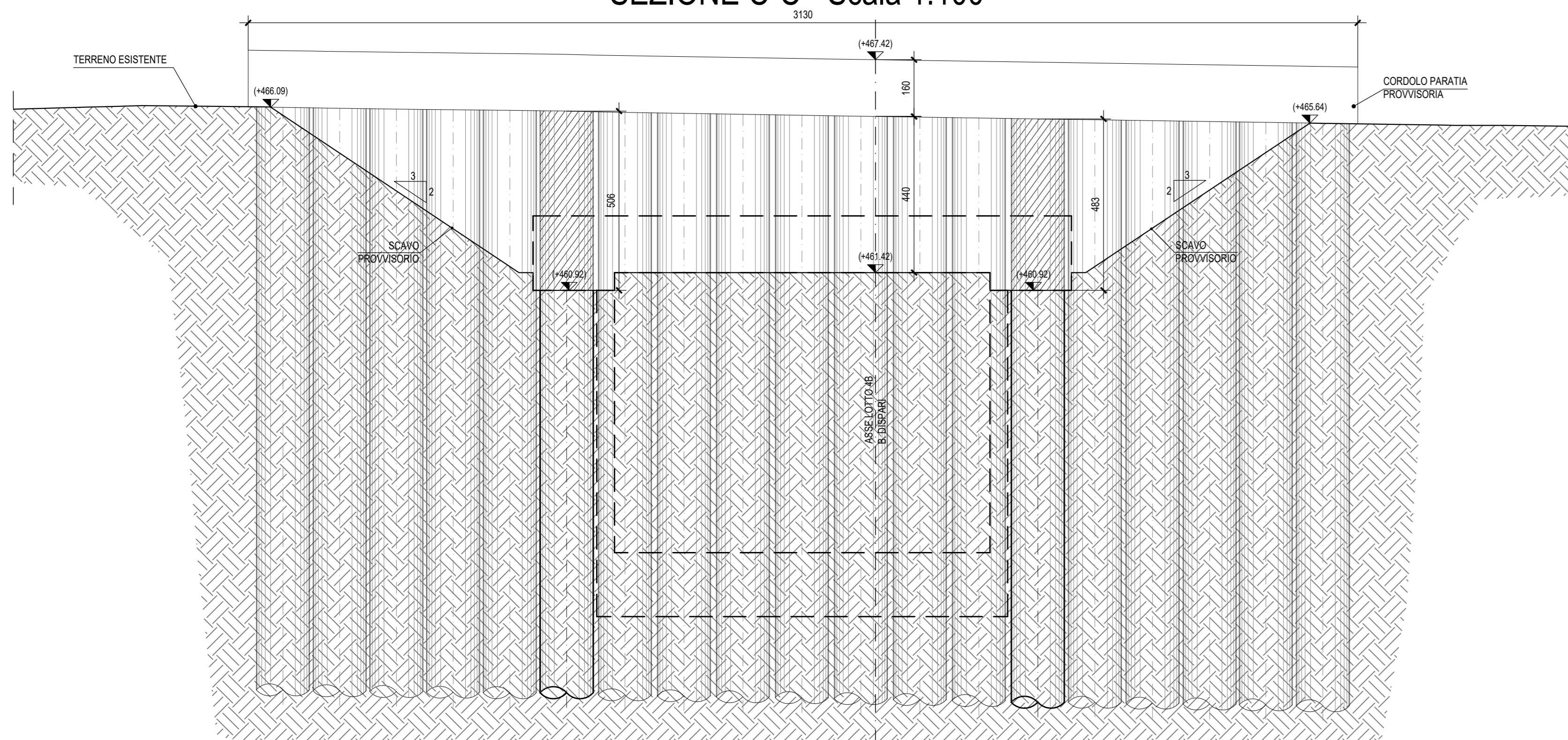
SEZIONE C-C - Scala 1:100
