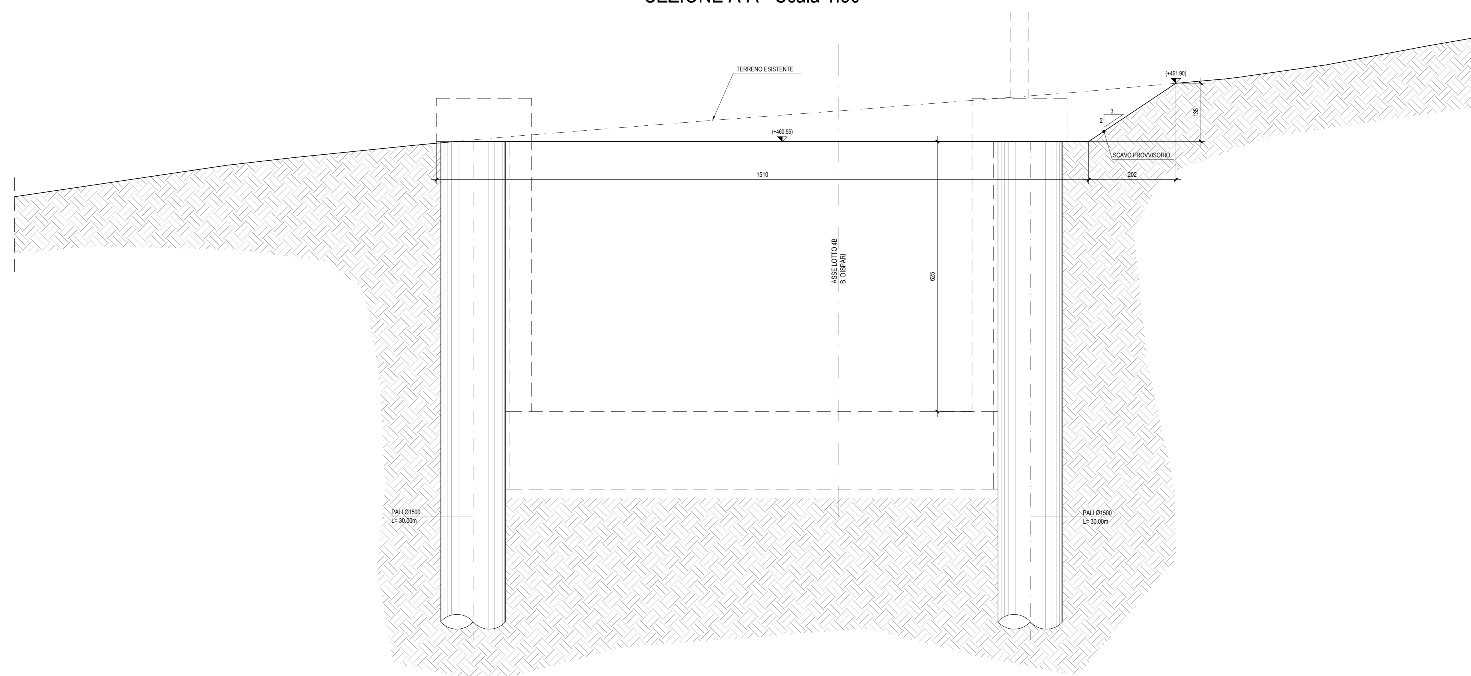
SEZIONE A-A - Scala 1:50
