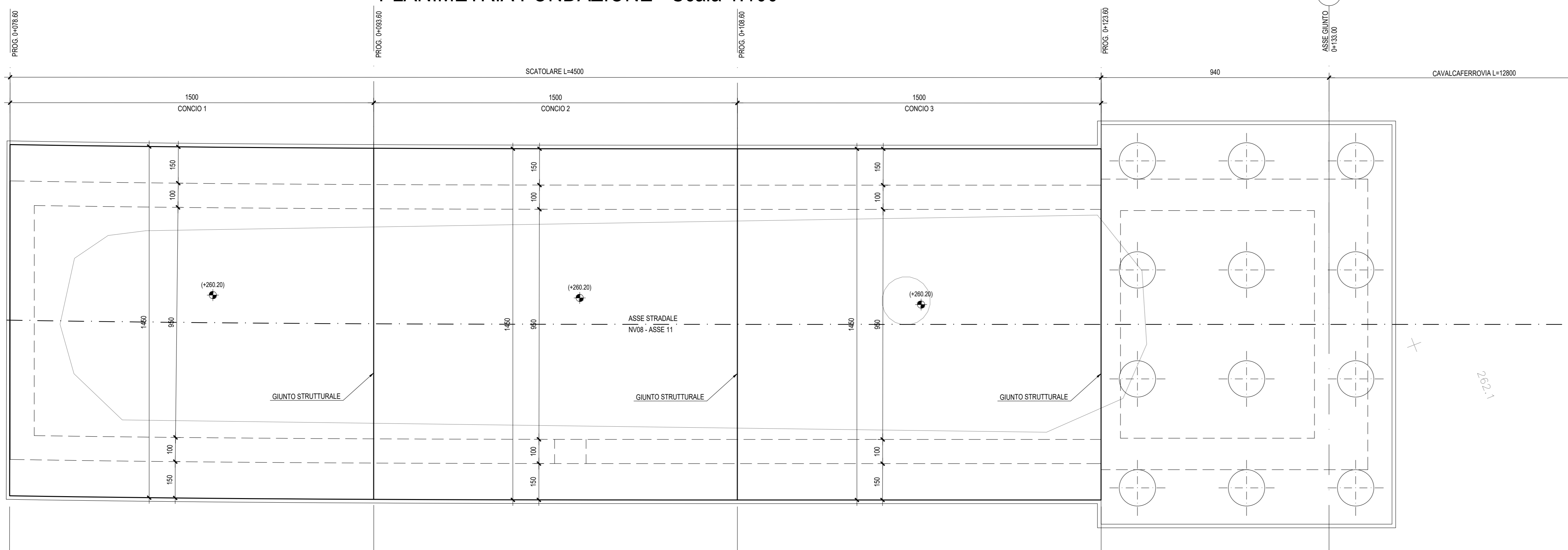
PLANIMETRIA SCAVO - Scala 1:100
