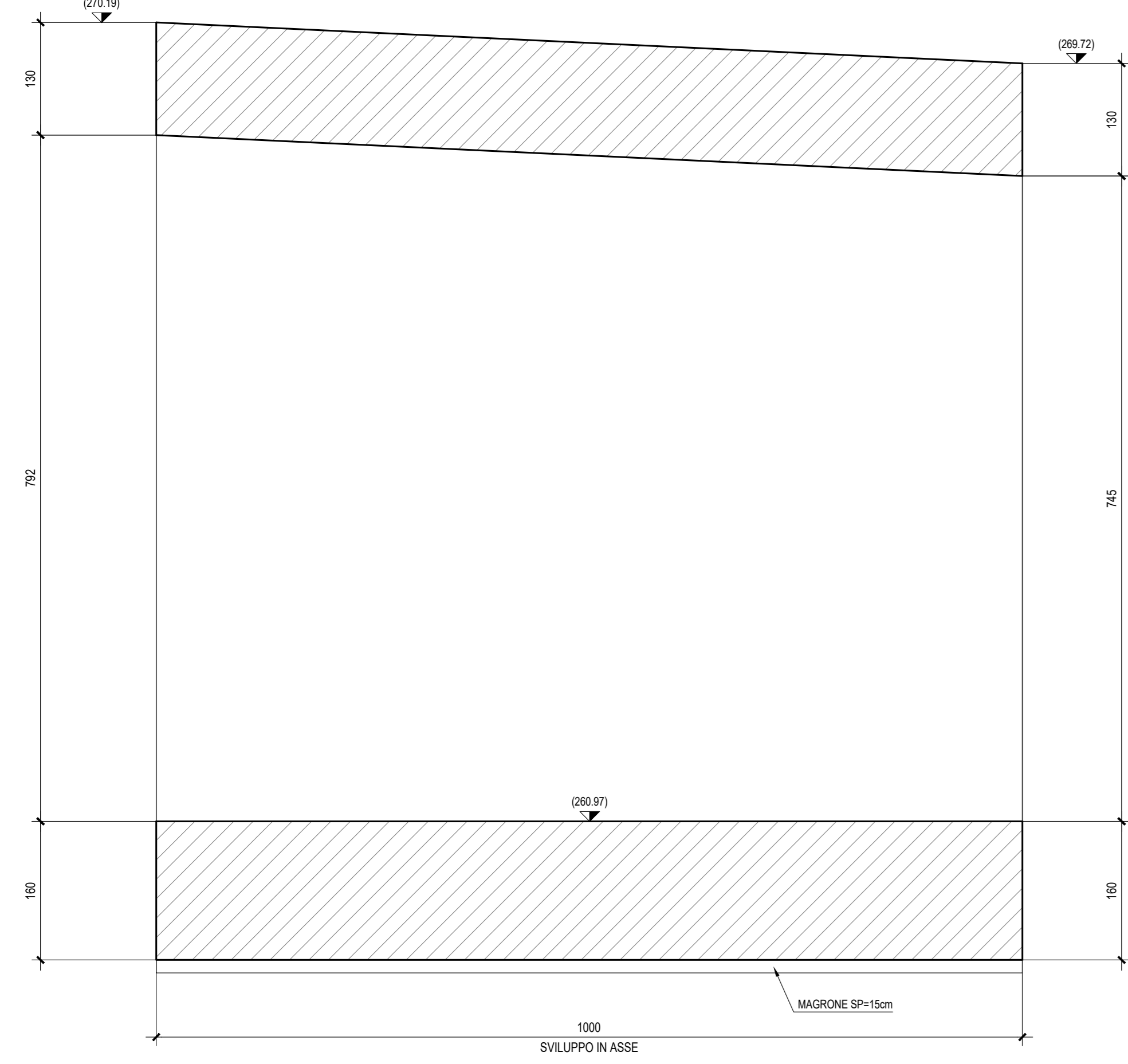
SEZIONE LONGITUDINALE - Scala 1:50
