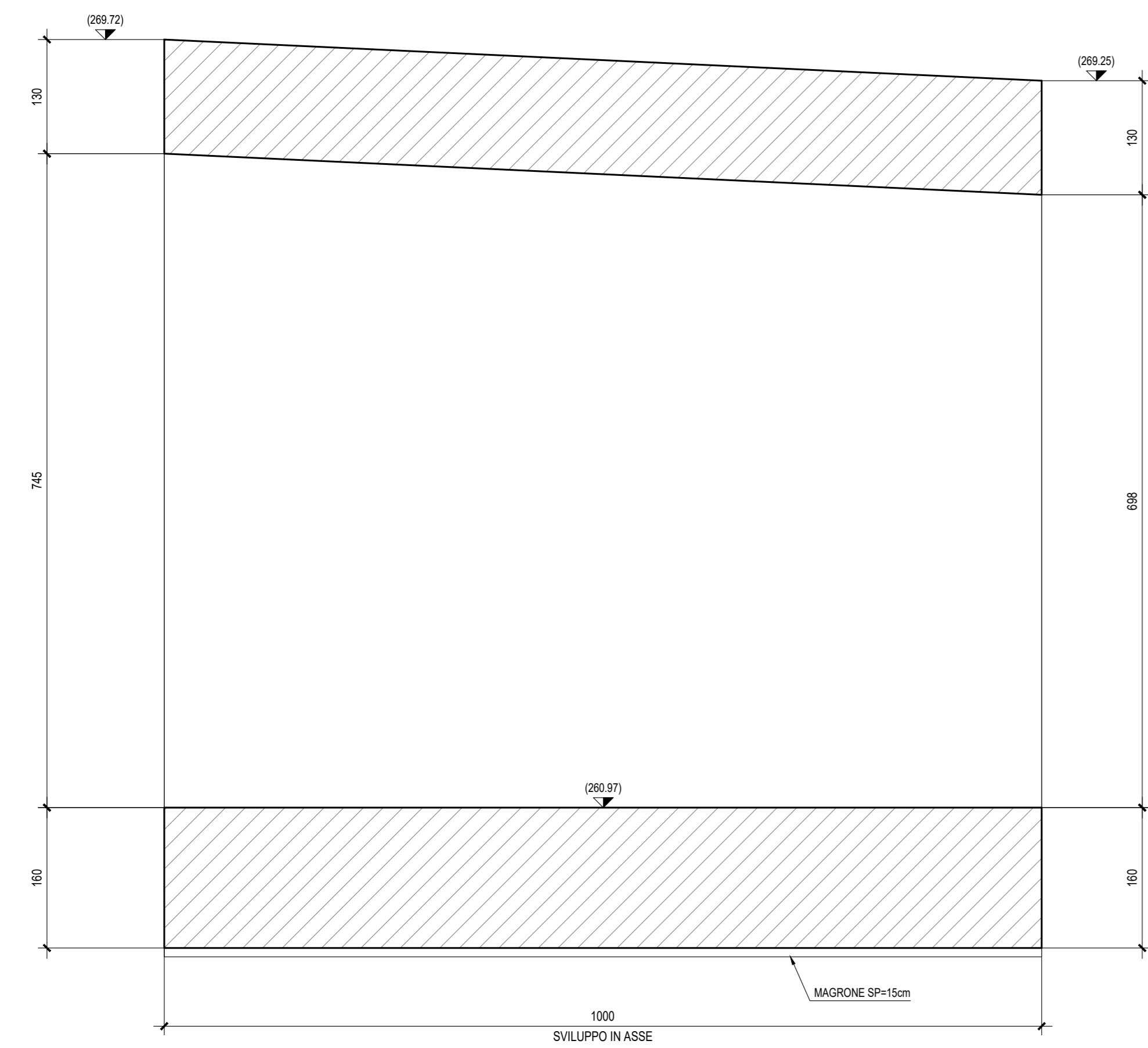
SEZIONE LONGITUDINALE - Scala 1:50
