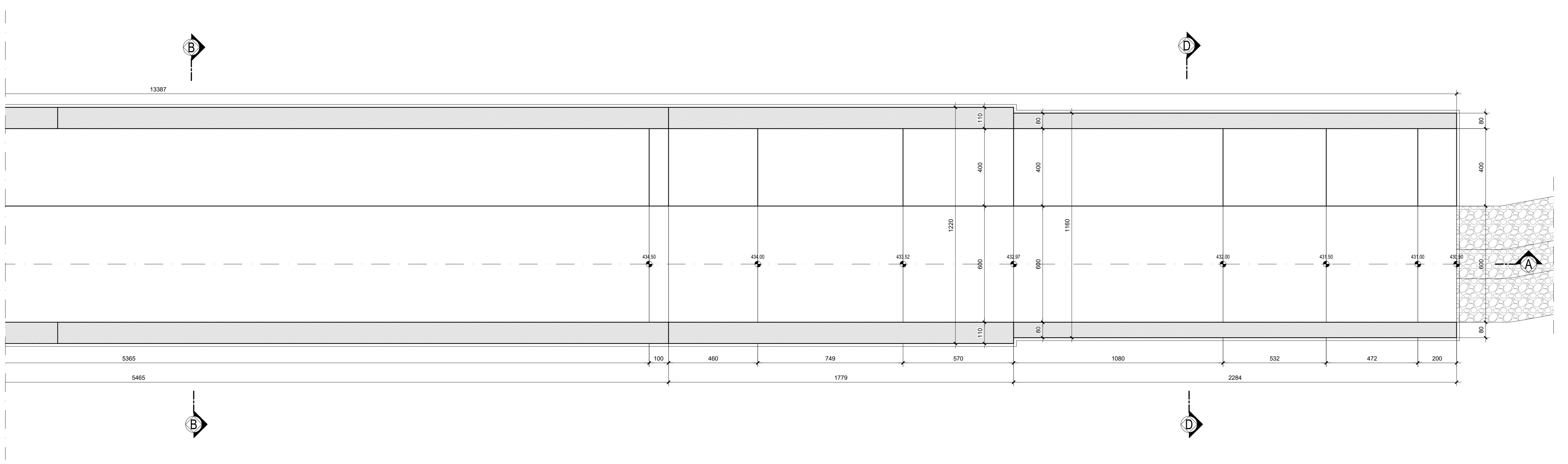
PIANTA SPICCATO - SCALA 1:100
