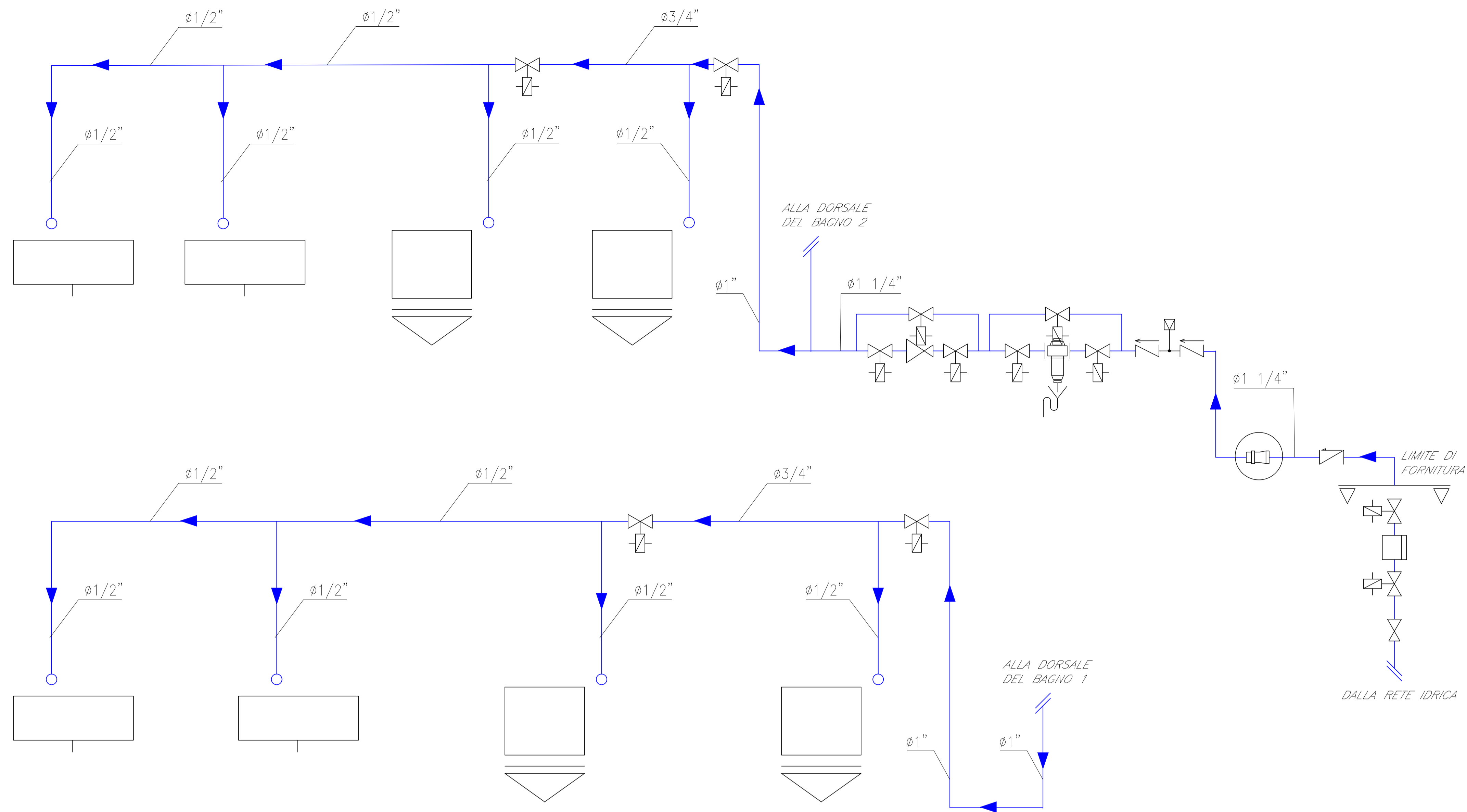
SCHEMA FUNZIONALE IMPIANTO IDRICO SANITARIO – SERVIZIO IGIENICO FV
