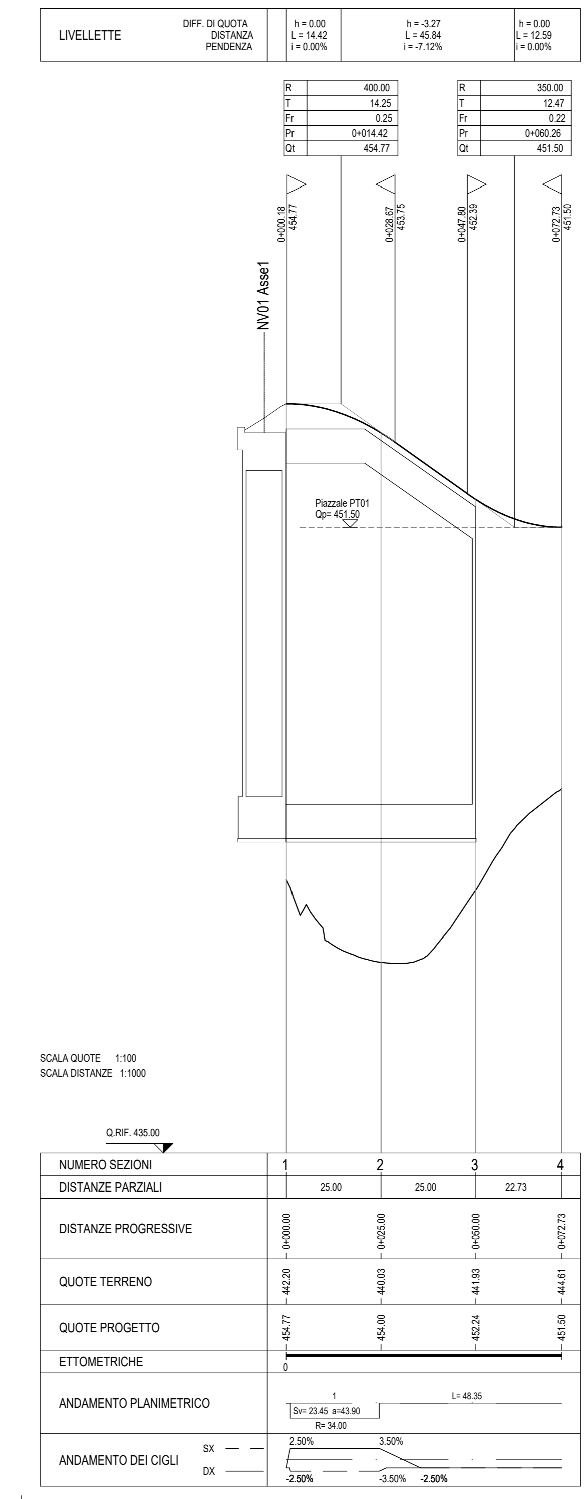
Profilo longitudinale Asse2
