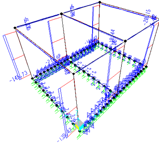
Sforzo Normale N - Involuppo SLU
