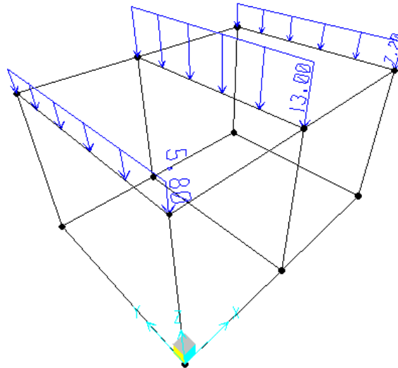
G1 – Peso solaio
