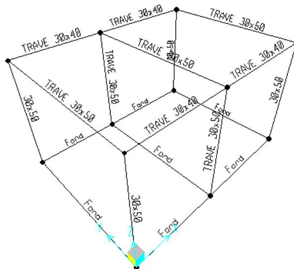
Figura 7: tipologia aste
