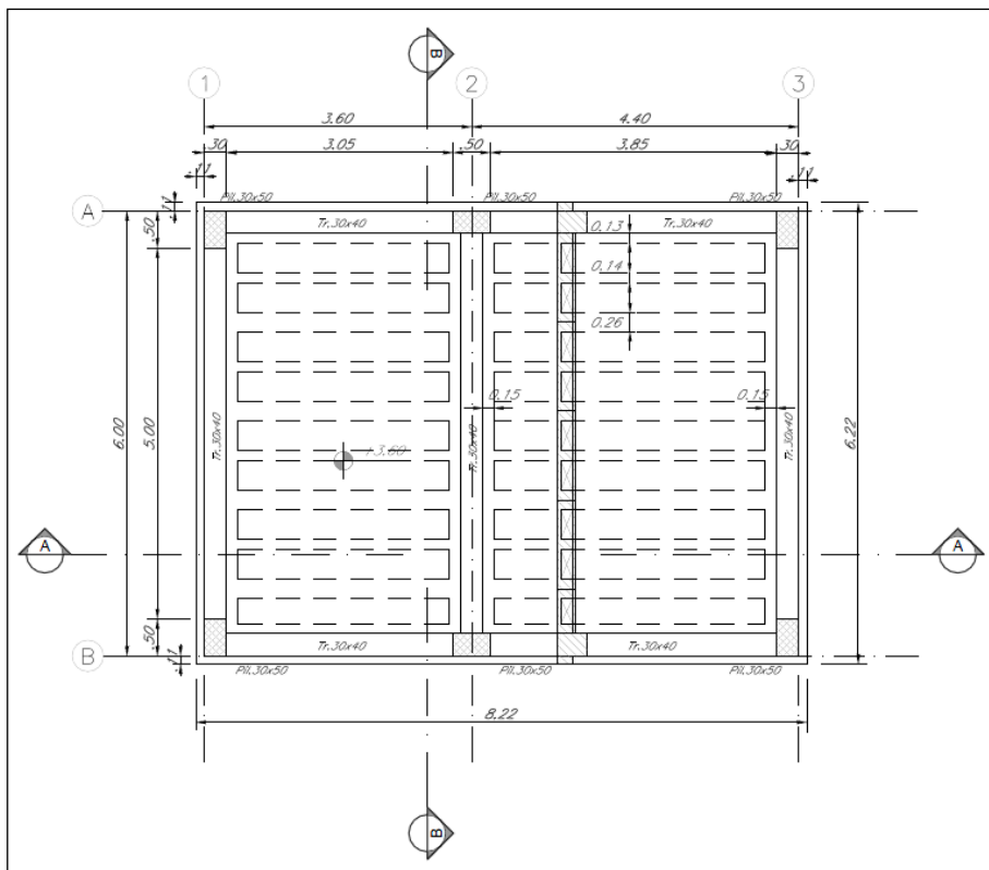
Figura 1-2. Carpenteria copertura.
