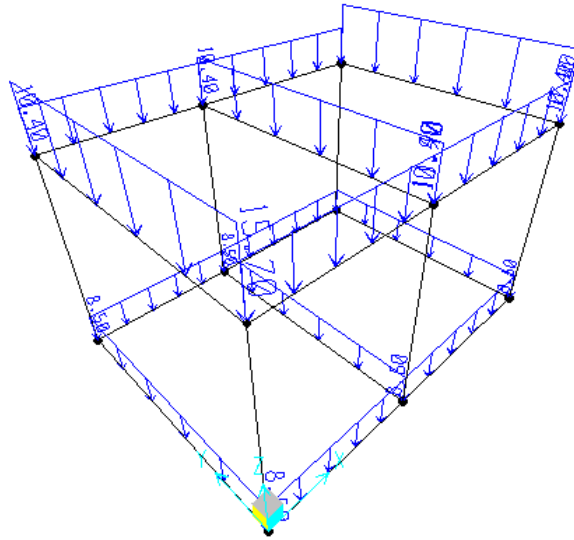
G2 – Permanenti non strutturali
