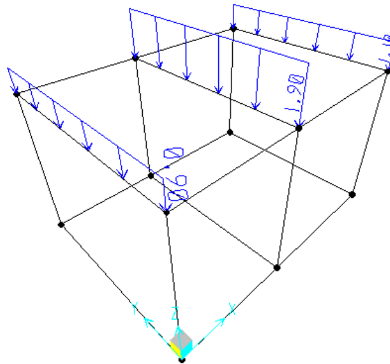
QH1 – Accidentali (Manutenzione)
