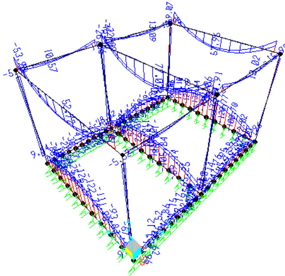
Momento M3 - Involuppo SLER
