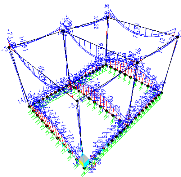
Momento M3 - Involuppo SLU
