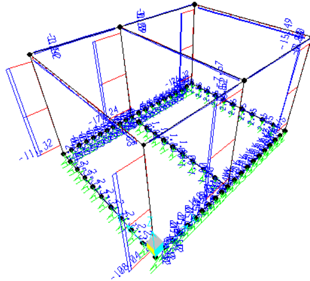
Sforzo Normale N - Involuppo SLER
