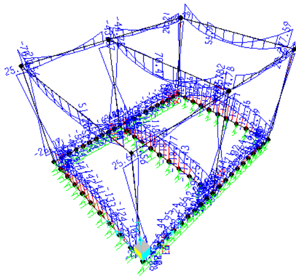
Momento M3 - Involuppo SLV
