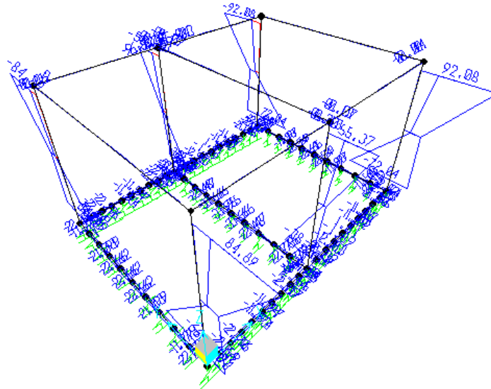
Momento M2 - Inviluppo SLV
