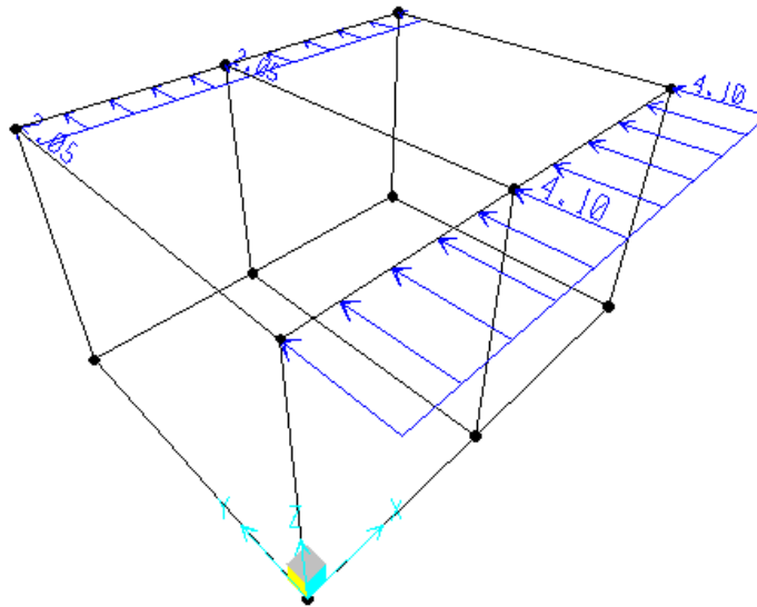
Vy+ – Vento Y+
