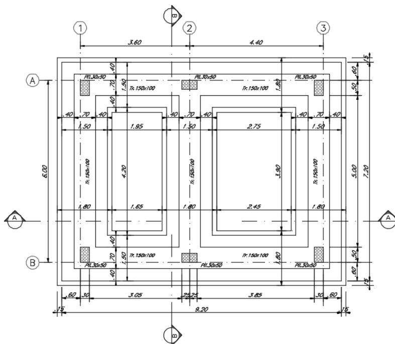
Figura 1-1. Carpenteria fondazioni.
