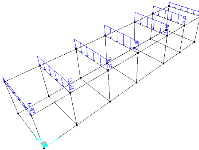
G1 – Peso solaio
