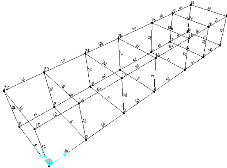
Figura 8: numerazione aste e nodi
