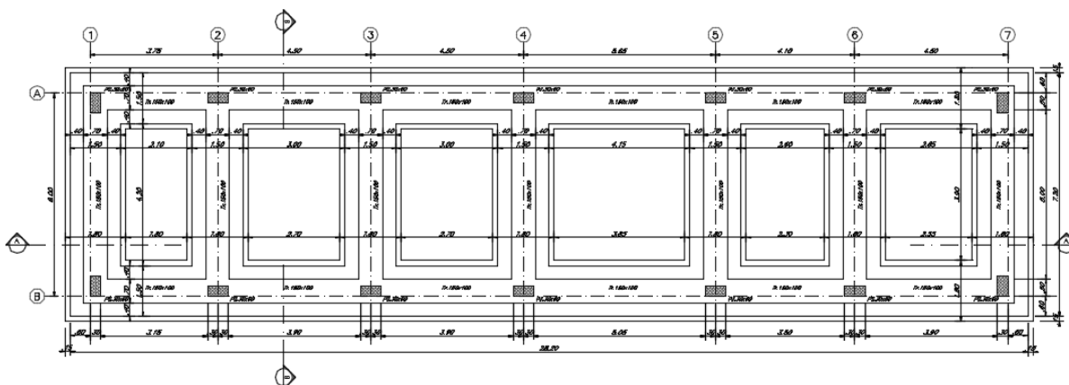
Figura 1-1. Carpenteria fondazioni.
