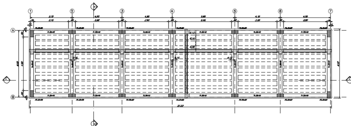
Figura 1-2. Carpenteria copertura.
