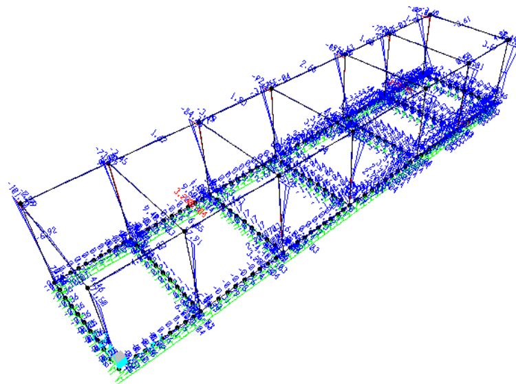
Momento M2 - Inviluppo SLU
