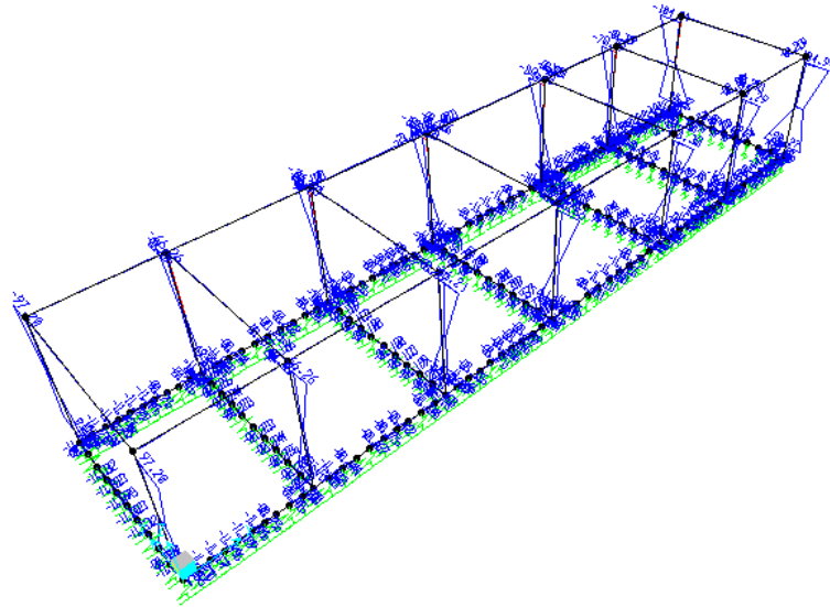
Momento M2 - Involuppo SLV
