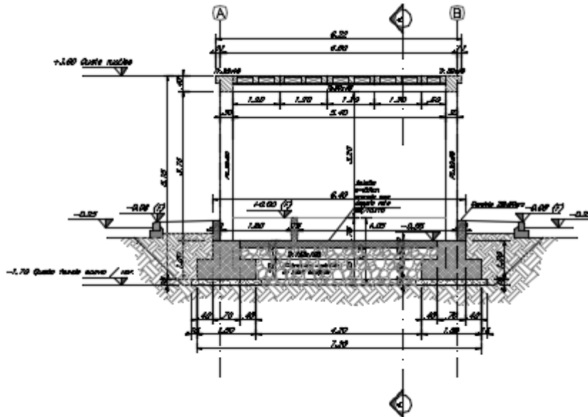
Figura 1-4. Sezione B
