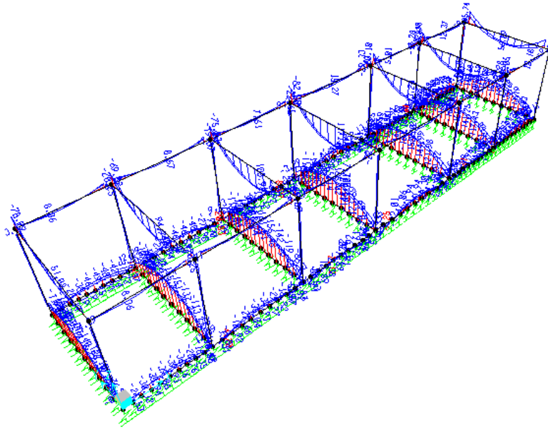
Momento M3 - Inviluppo SLU
