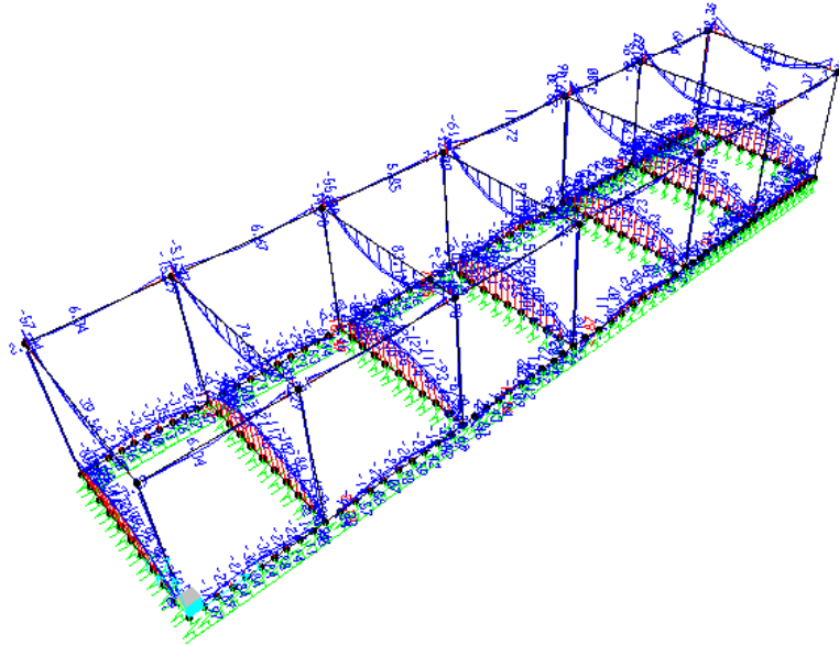
Momento M3 - Involuppo SLER
