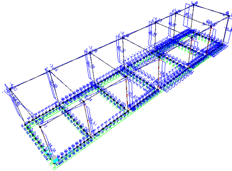
Taglio V3 - Involuppo SLU
