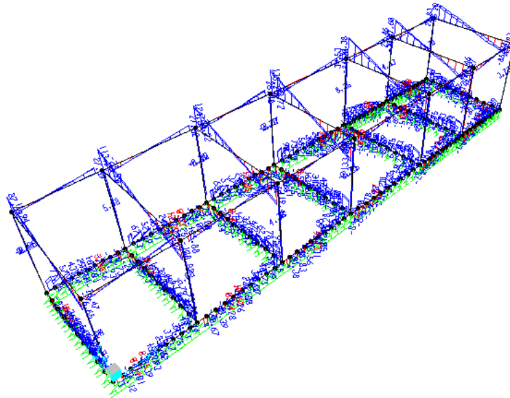
Taglio V2 - Involuppo SLU
