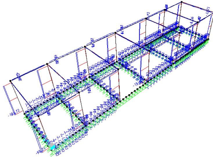
Sforzo Normale N - Involuppo SLER
