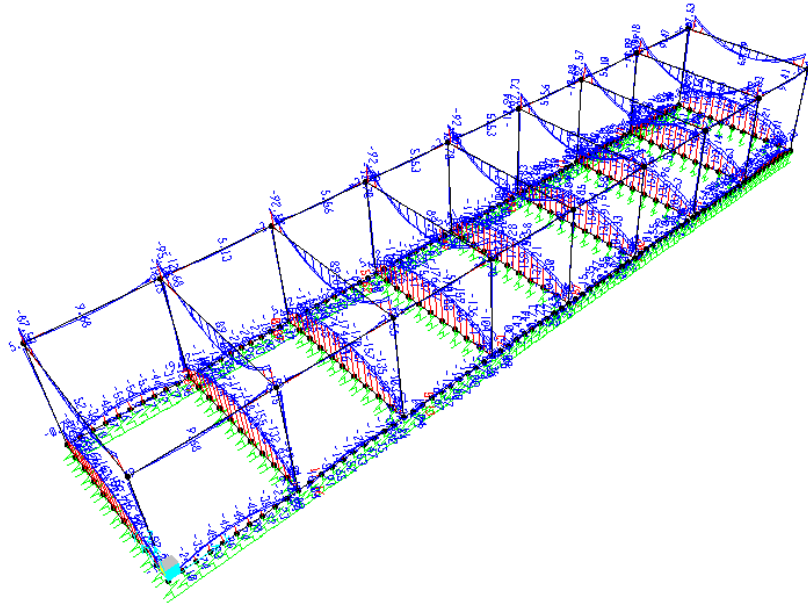
Momento M3 - Involuppo SLER
