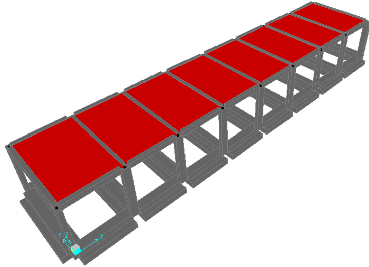
Figura 1-5. Vista estrusa modello FEM
