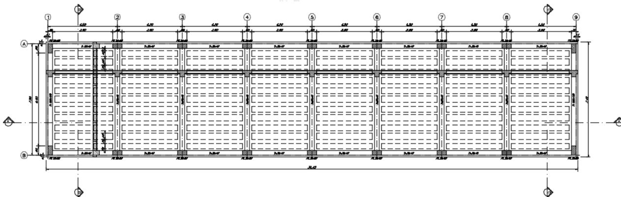
Figura 1-2. Carpenteria copertura.
