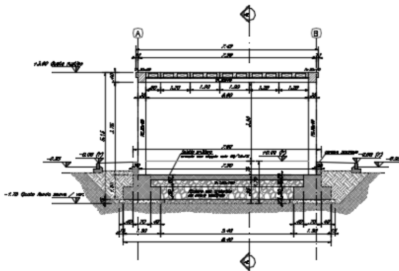
Figura 1-3. Sezione A
