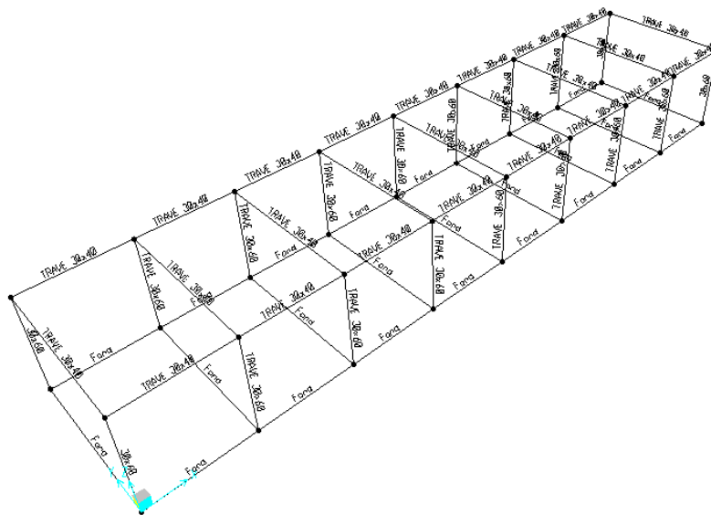
Figura 7: tipologia aste
