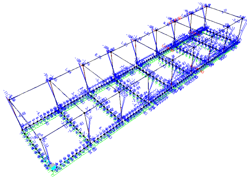
Momento M2 - Involuppo SLER
