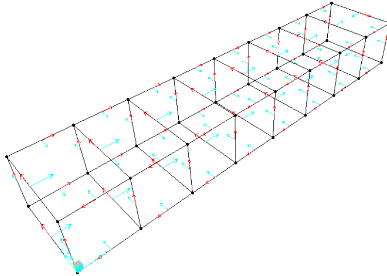
Figura 6: assi locali
