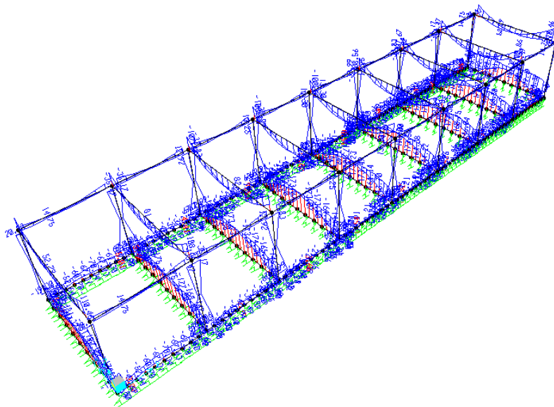
Momento M3 - Involuppo SLV
