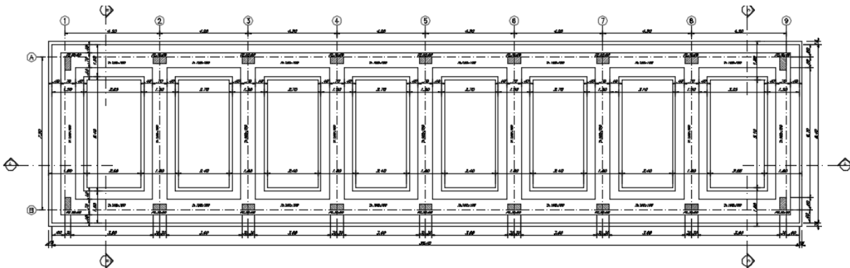
Figura 1-1. Carpenteria fondazioni.
