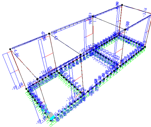
Sforzo Normale N - Involuppo SLV
