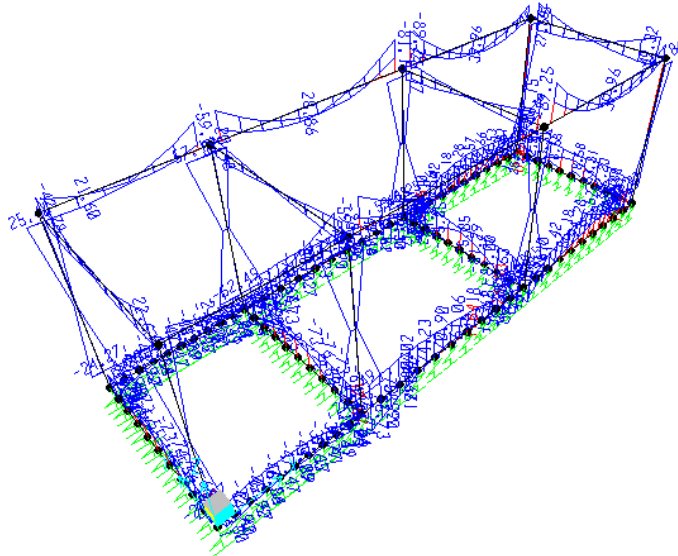
Momento M3 - Inviluppo SLV
