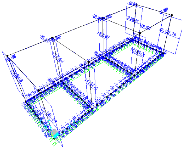
Taglio V3 - Inviluppo SLV
