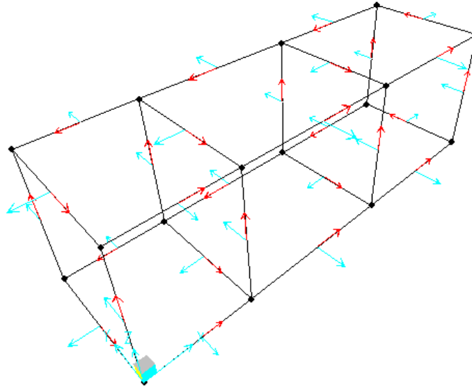
Figura 6: assi locali
