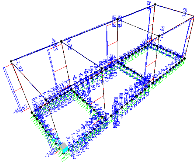
Sforzo Normale N - Involuppo SLER
