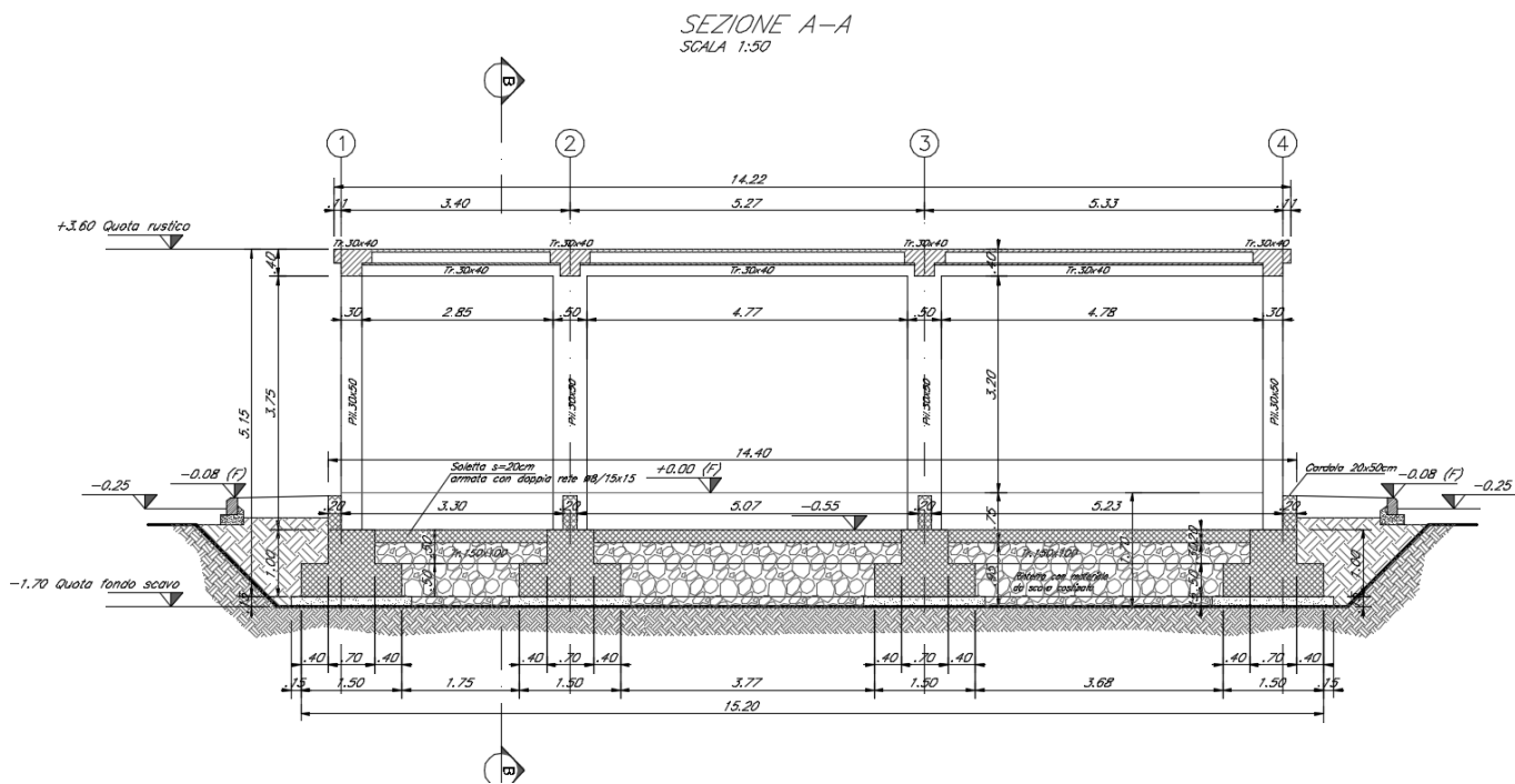
Figura 1-3. Sezione A
