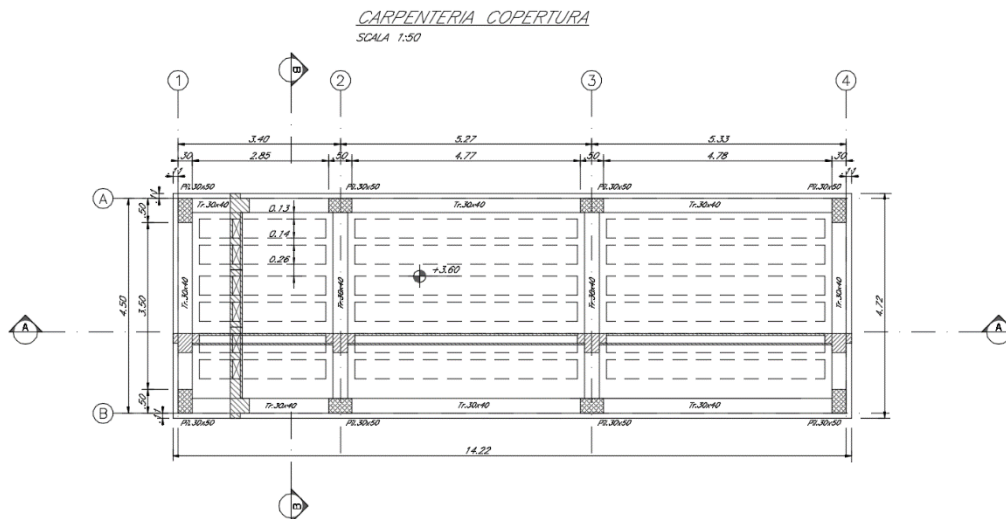
Figura 1-2. Carpenteria copertura.
