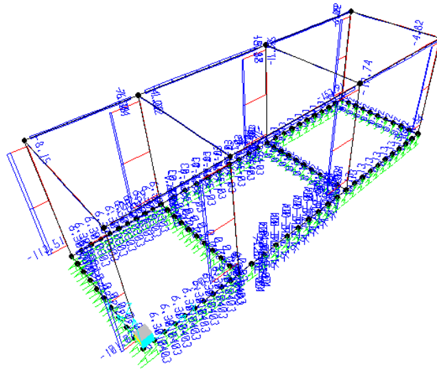
Sforzo Normale N - Inviluppo SLU
