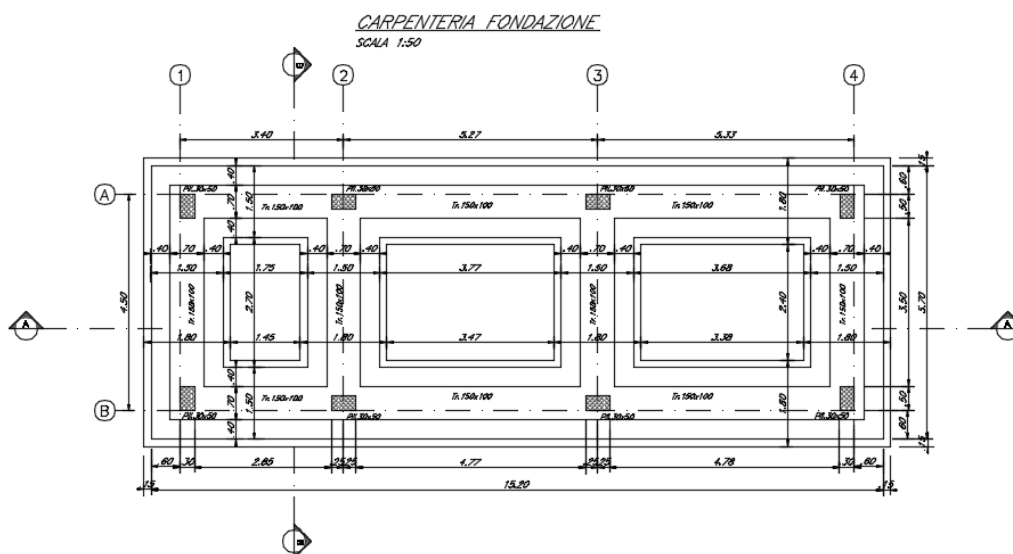
Figura 1-1. Carpenteria fondazioni.
