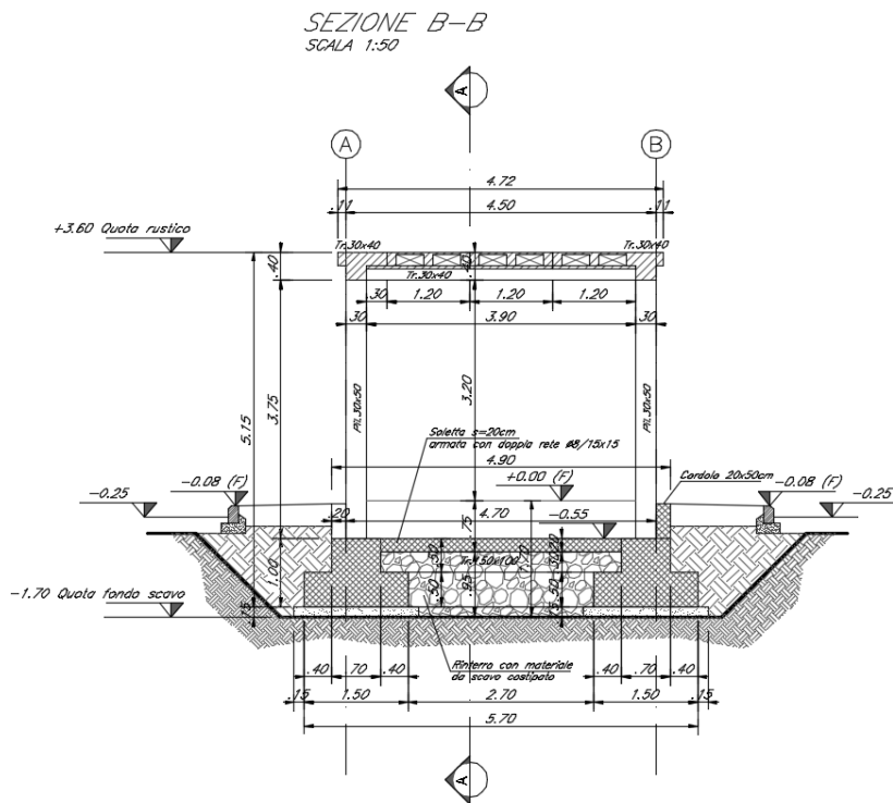
Figura 1-4. Sezione B
