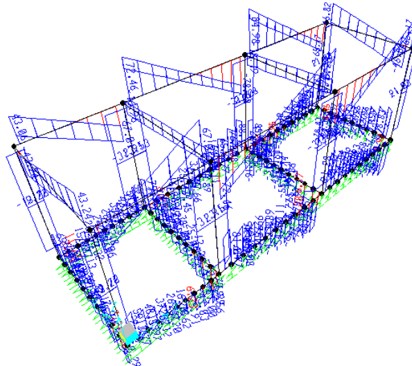
Taglio V2 - Involuppo SLV
