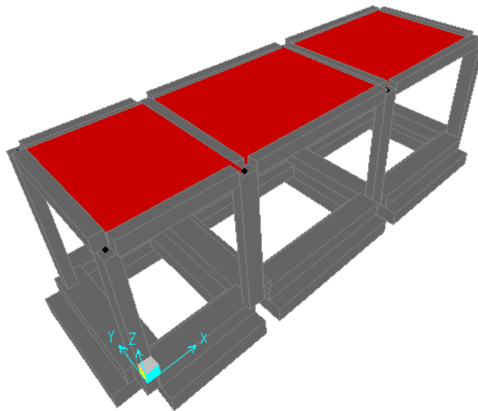
Figura 1-5. Vista estrusa modello FEM
