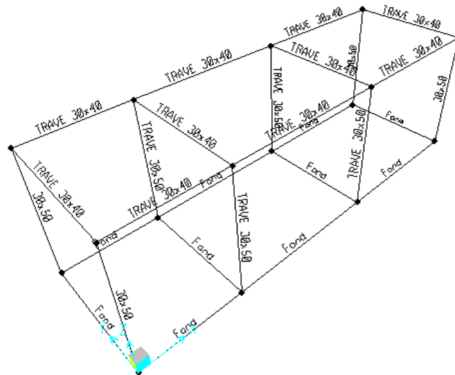
Figura 7: tipologia aste
