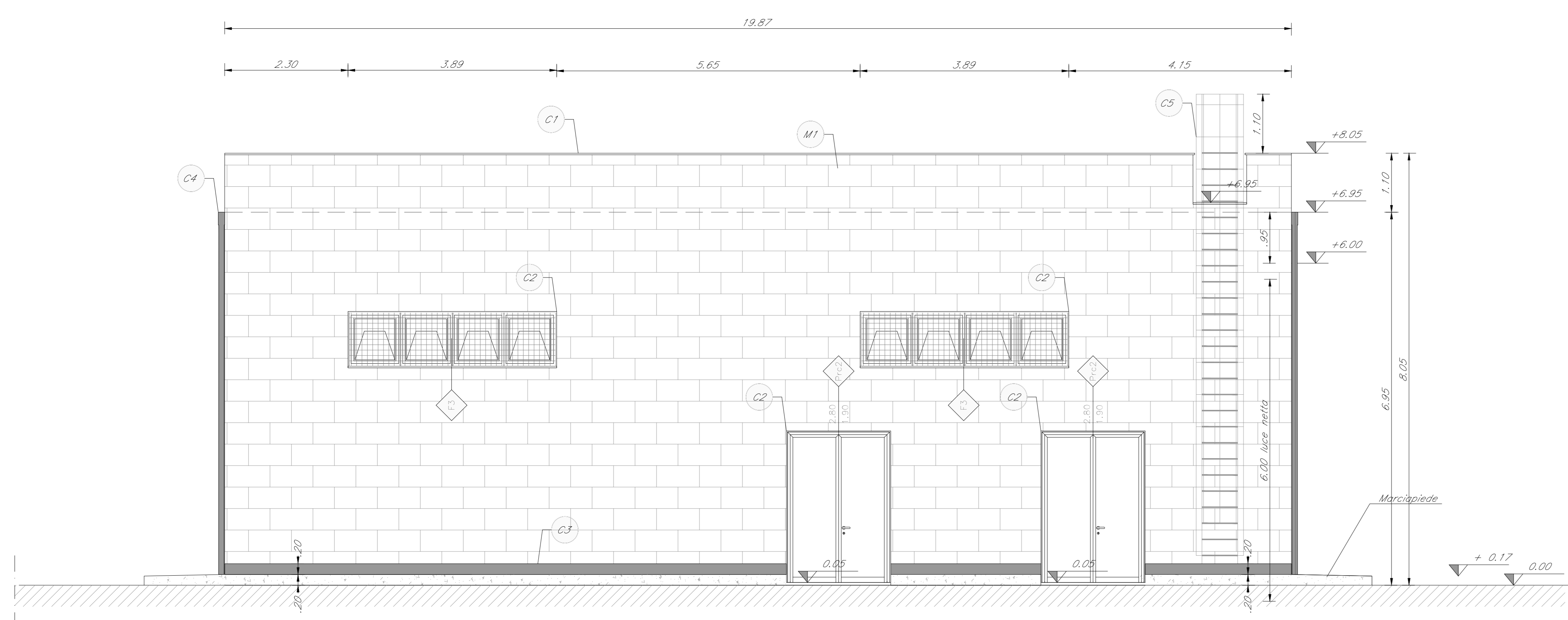
PROSPETTO P2 SCALA 1:50
