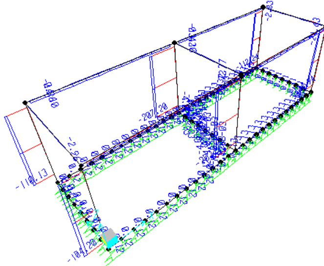
Sforzo Normale N - Involuppo SLER
