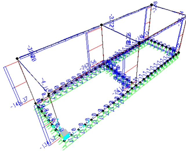
Sforzo Normale N - Inviluppo SLU
