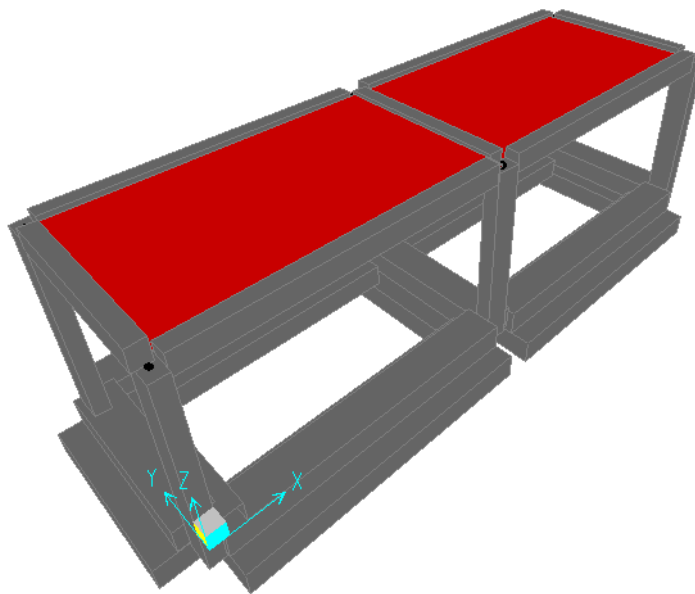
Figura 1-5. Vista estrusa modello FEM
