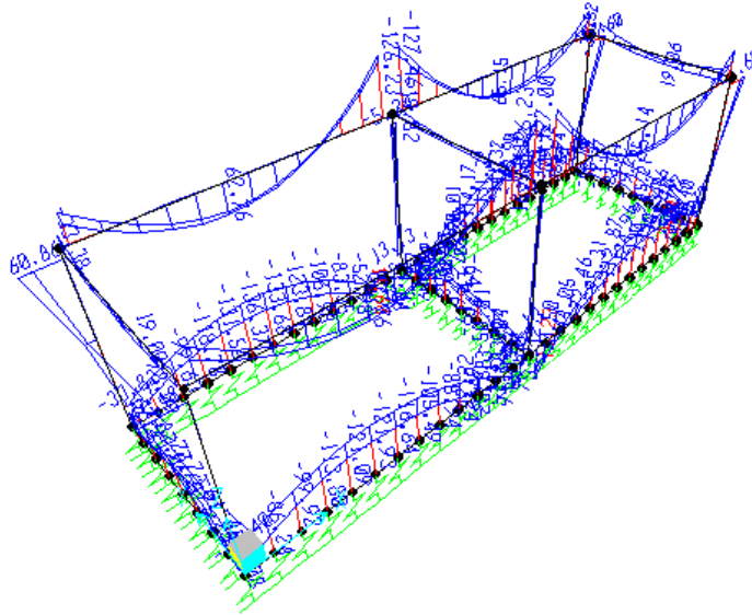
Momento M3 - Involuppo SLU
