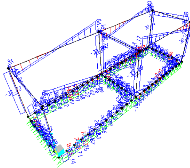
Taglio V2 - Inviluppo SLV
