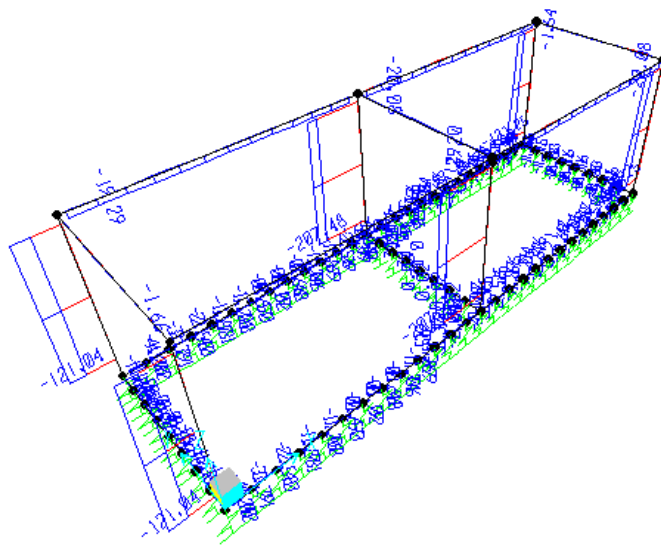
Sforzo Normale N - Inviluppo SLV
