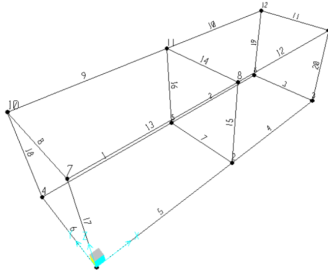
Figura 8: numerazione aste e nodi
