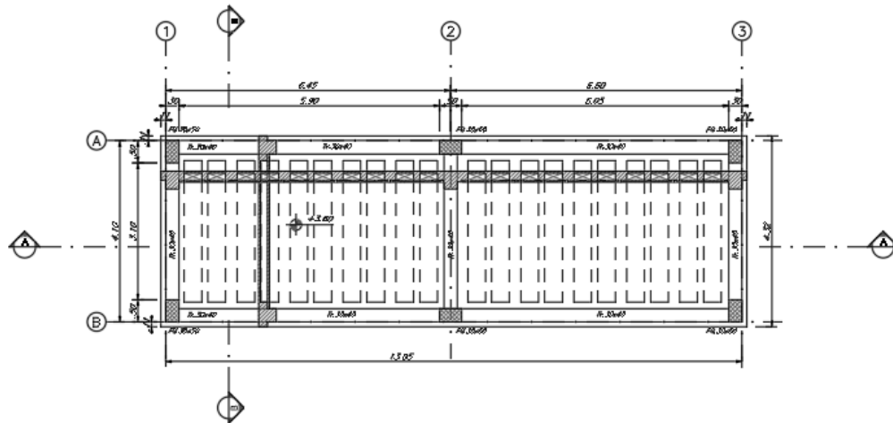
Figura 1-2. Carpenteria copertura.
