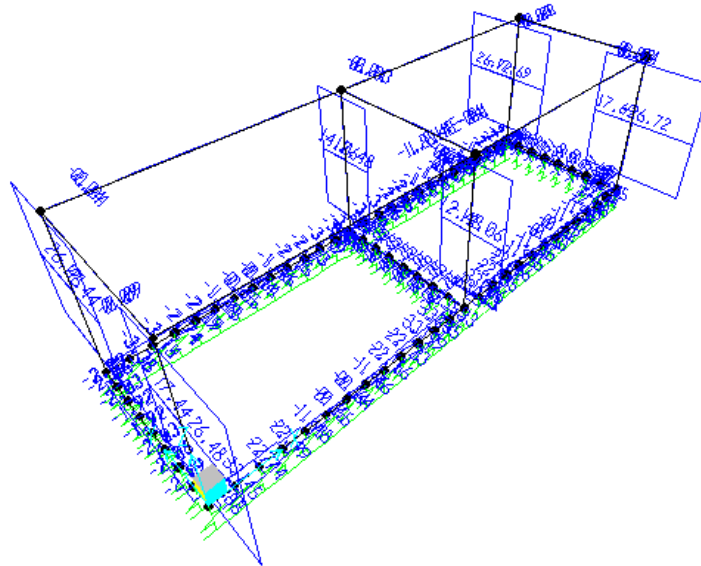
Taglio V3 - Involuppo SLV
