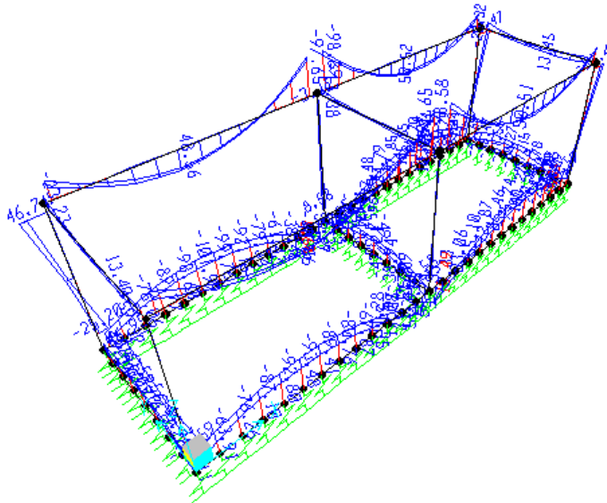
Momento M3 - Involuppo SLER
