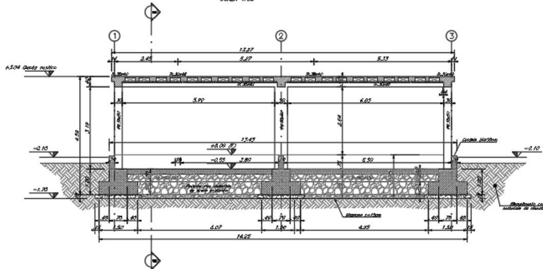
Figura 1-3. Sezione A
