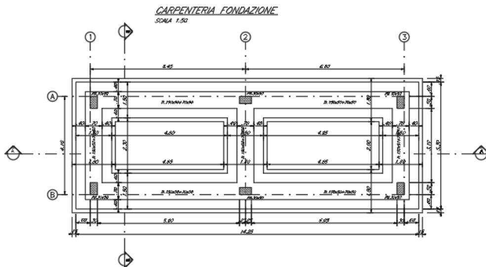
Figura 1-1. Carpenteria fondazioni.
