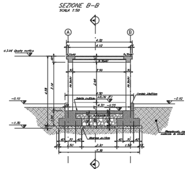
Figura 1-4. Sezione B
