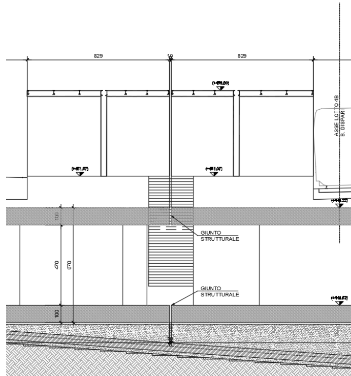
Figura 1-2. Sezione
