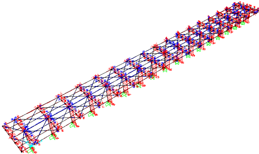
Sforzo Normale N - Involuppo SLU
