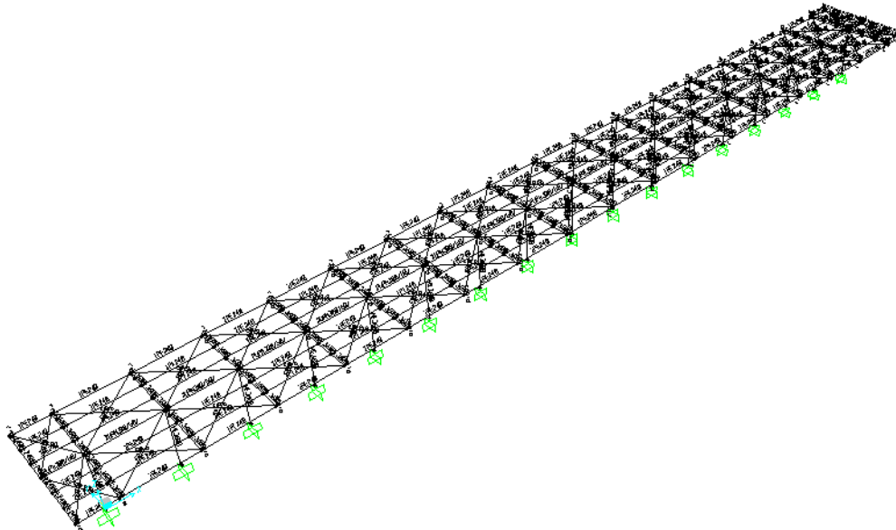
Figura 5: tipologia aste
