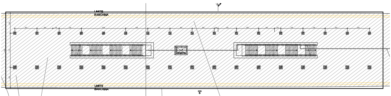
Figura 1-1. Carpenteria fondazioni.
