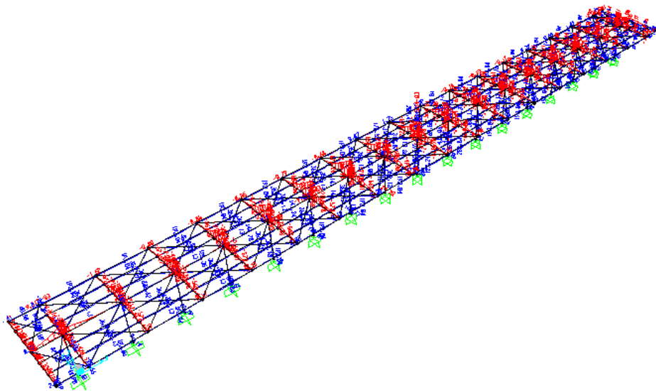
Momento M3 - Involuppo SLU
