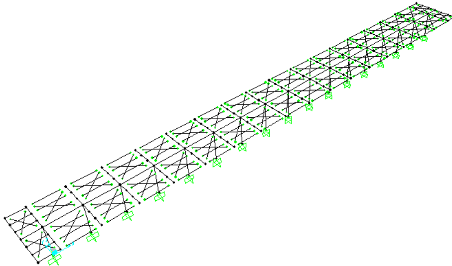
Figura 7: aste rilasciate
