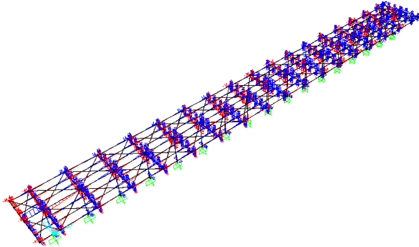
Taglio V2 - Involuppo SLU
