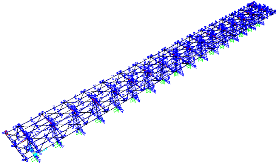
Momento M3 - Inviluppo SLV
