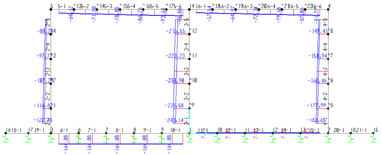
Fig. 9 – Involuppo azioni assiali SLV
