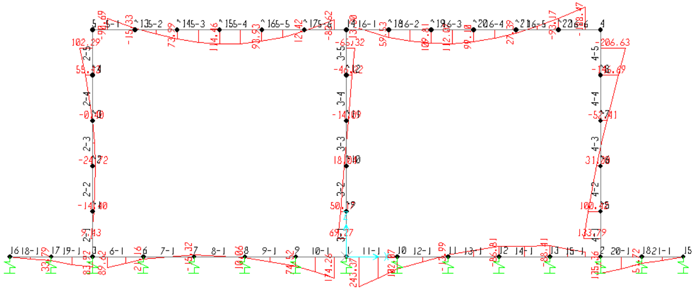
Fig. 10 – Involuppo momenti flettenti SLE rara
