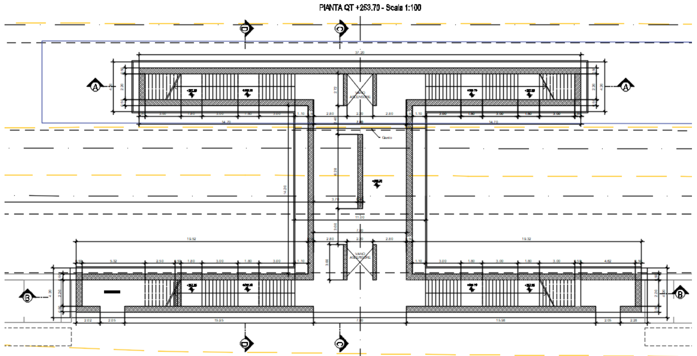
Fig. 2 - Pianta quota sottopasso
