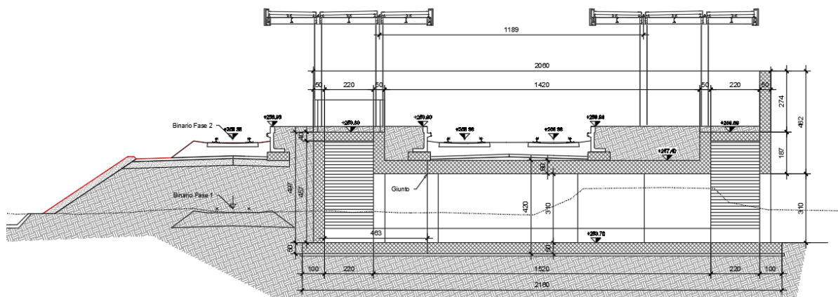
Fig. 1 –Sezione longitudinale
