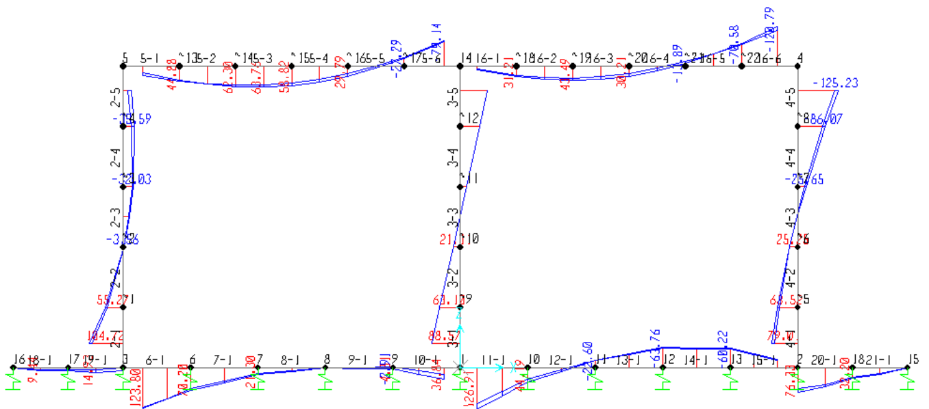
Fig. 7 – Involuppo momenti flettenti SLV
