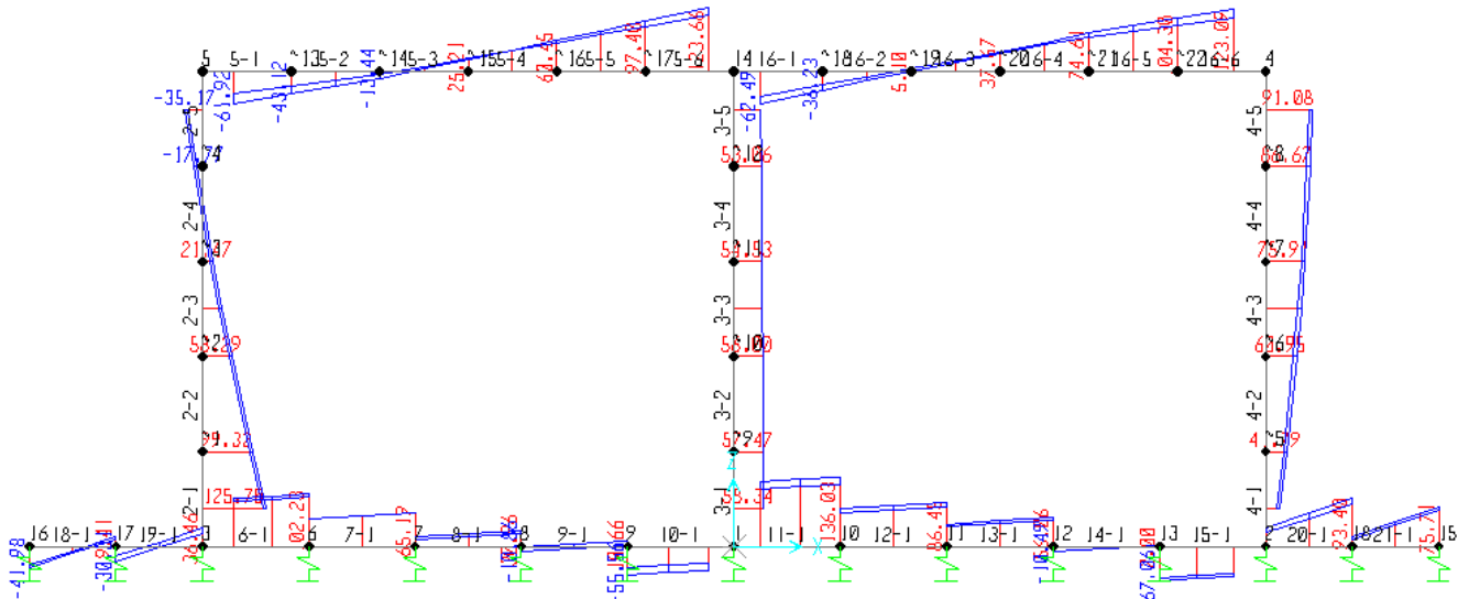
Fig. 8 – Involuppo sforzi taglianti SLV
