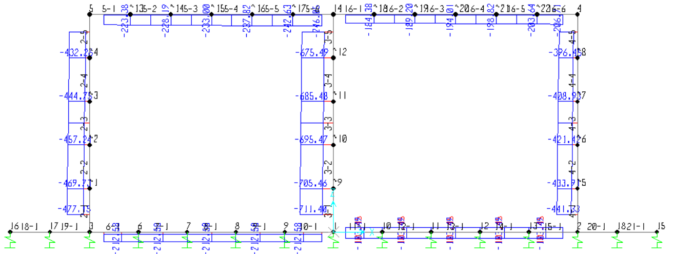
Fig. 6 – Involuppo azioni assiali SLU
