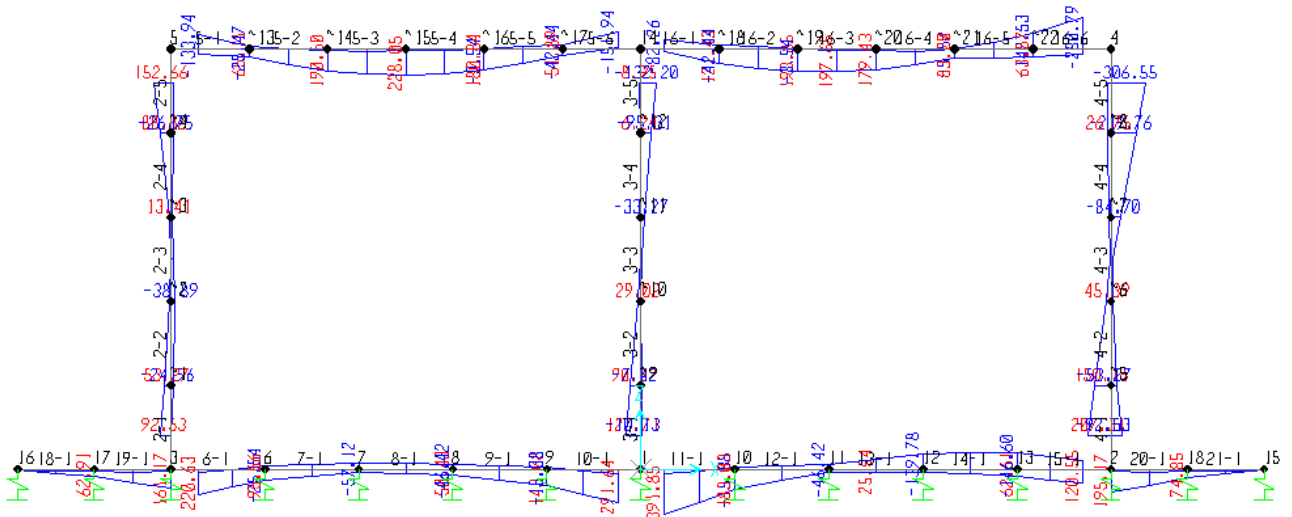
Fig. 4 – Involuppo momenti flettenti SLU
