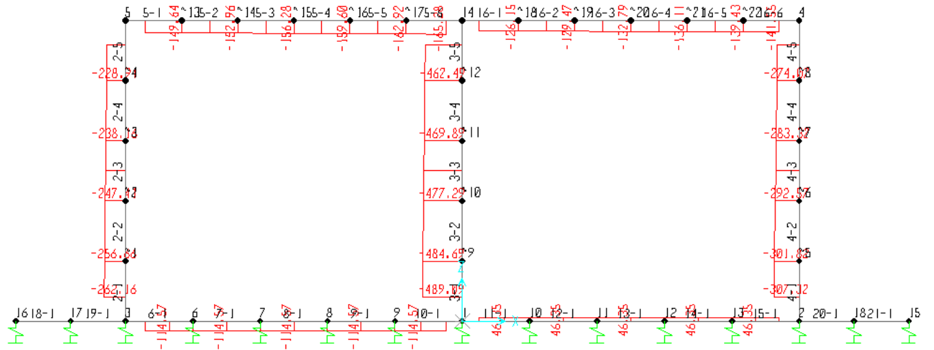
Fig. 11 – Involuppo azioni assiali SLE rara
