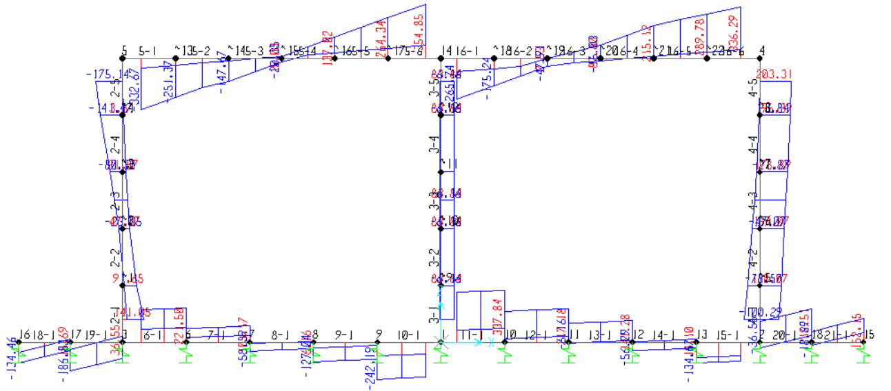
Fig. 5 – Involuppo sforzi taglienti SLU
