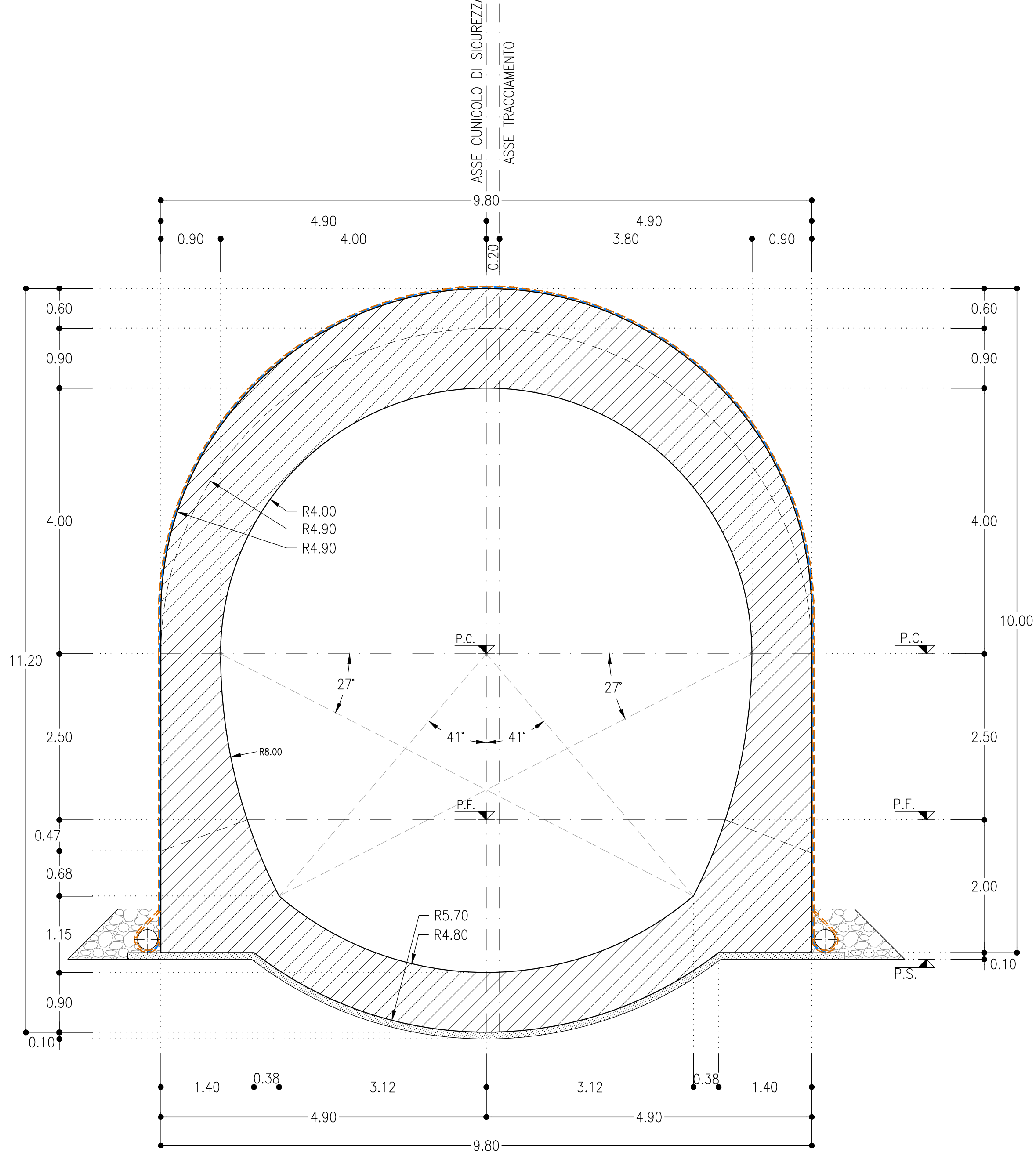
SEZIONE B-B SCALA 1:50 CARPENTERIA
