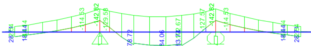
Soll. Flettenti SLE Combinazione rara
