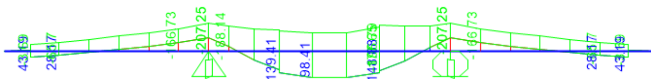
Involuppo sollecitazioni flettenti (S.L.U.)
