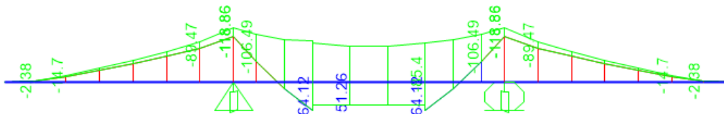
Soll. Flettenti SLE Combinazione frequente
