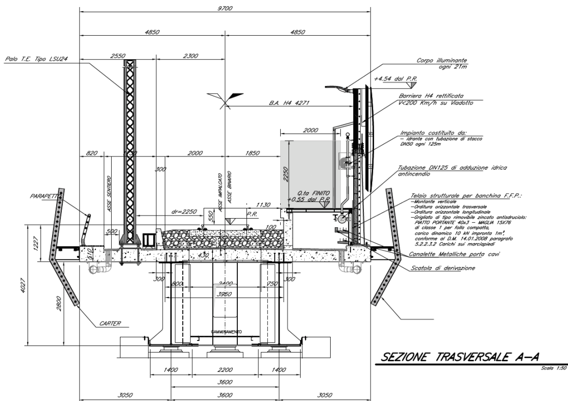
Figura 2_ Sezione in asse appoggi
