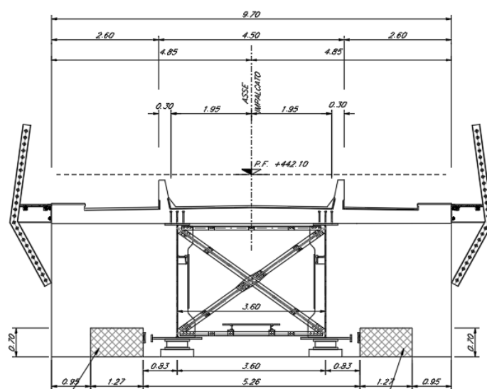
Figura 1 - Sezione trasversale
