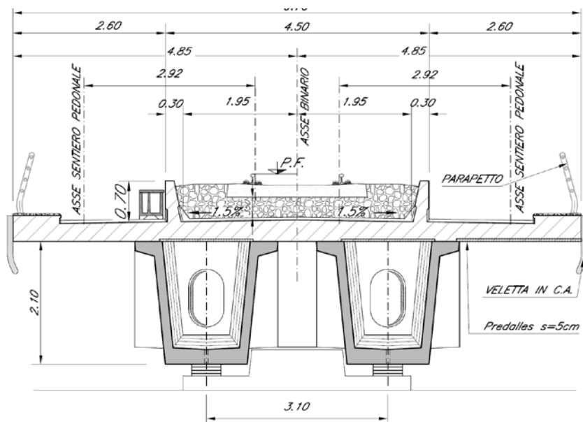
Figura 1 - Sezione trasversale campate in c.a.p. L=25 m
