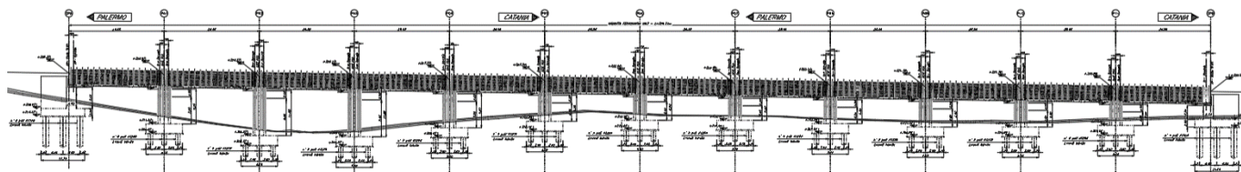
Figura 2 – Prospetto viadotto VI03
