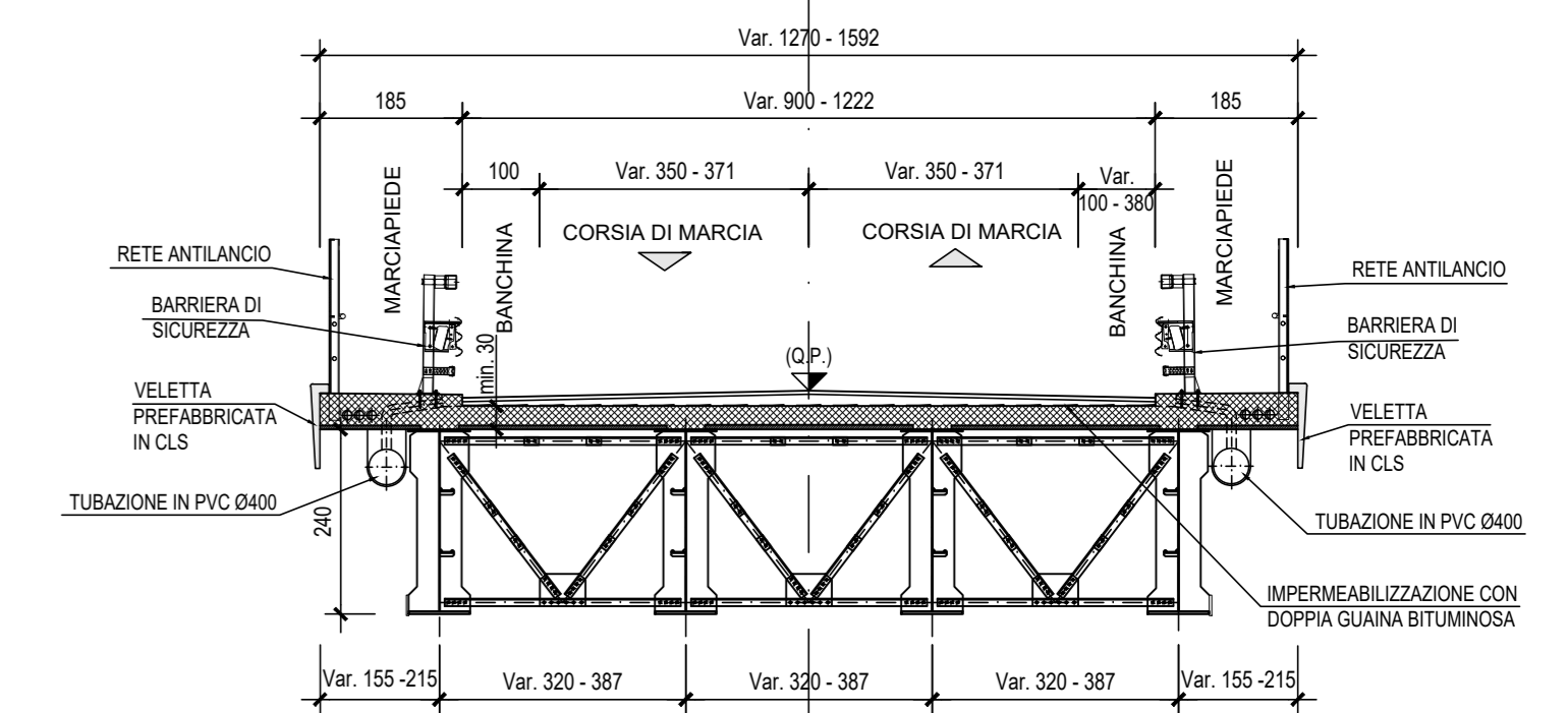
SEZIONE TIPO TRAVI (H=240) - Scala 1:100
