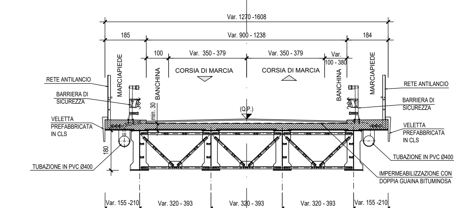
SEZIONE TIPO TRAVI (H=180) - Scala 1:100
