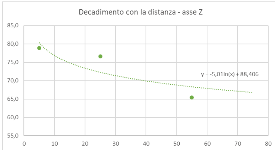
Figura 4-3 Curva di attenuazione del Leq,te in funzione della distanza dal binario, ricavata dai rilievi lungo l'asse Z, in corrispondenza della Terna 1 (5 metri), della Terna 2 (25 metri) e della Terna 3 (55 metri) e relativa al totale dei transiti ferroviari rilevati durante il periodo di osservazione.
