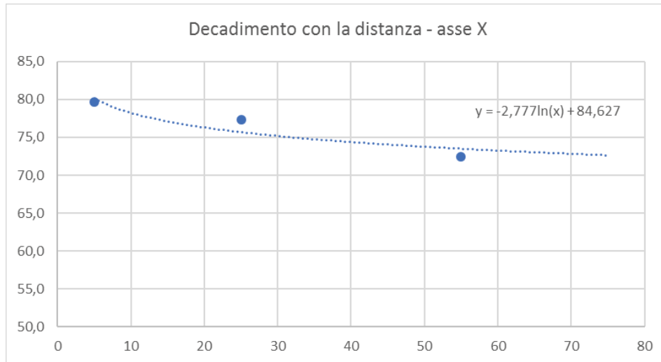
Figura 4-1 Curva di attenuazione del Leq,te in funzione della distanza dal binario, ricavata dai rilievi lungo l'asse X, in corrispondenza della Terna 1 (5 metri), della Terna 2 (25 metri) e della Terna 3 (55 metri) e relativa al totale dei transiti ferroviari rilevati durante il periodo di osservazione.
