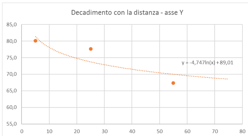
Figura 4-2 Curva di attenuazione del Leq,te in funzione della distanza dal binario, ricavata dai rilievi lungo l'asse Y, in corrispondenza della Terna 1 (5 metri), della Terna 2 (25 metri) e della Terna 3 (55 metri) e relativa al totale dei transiti ferroviari rilevati durante il periodo di osservazione.
