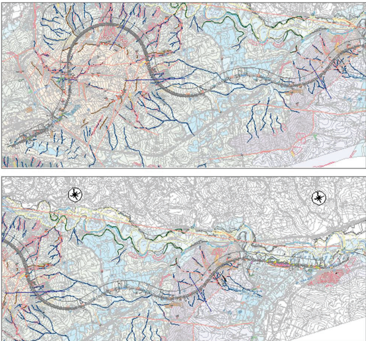
Figura 2-2 Stralcio della carta geologica con elementi di geomorfologia – inquadramento della linea di progetto
