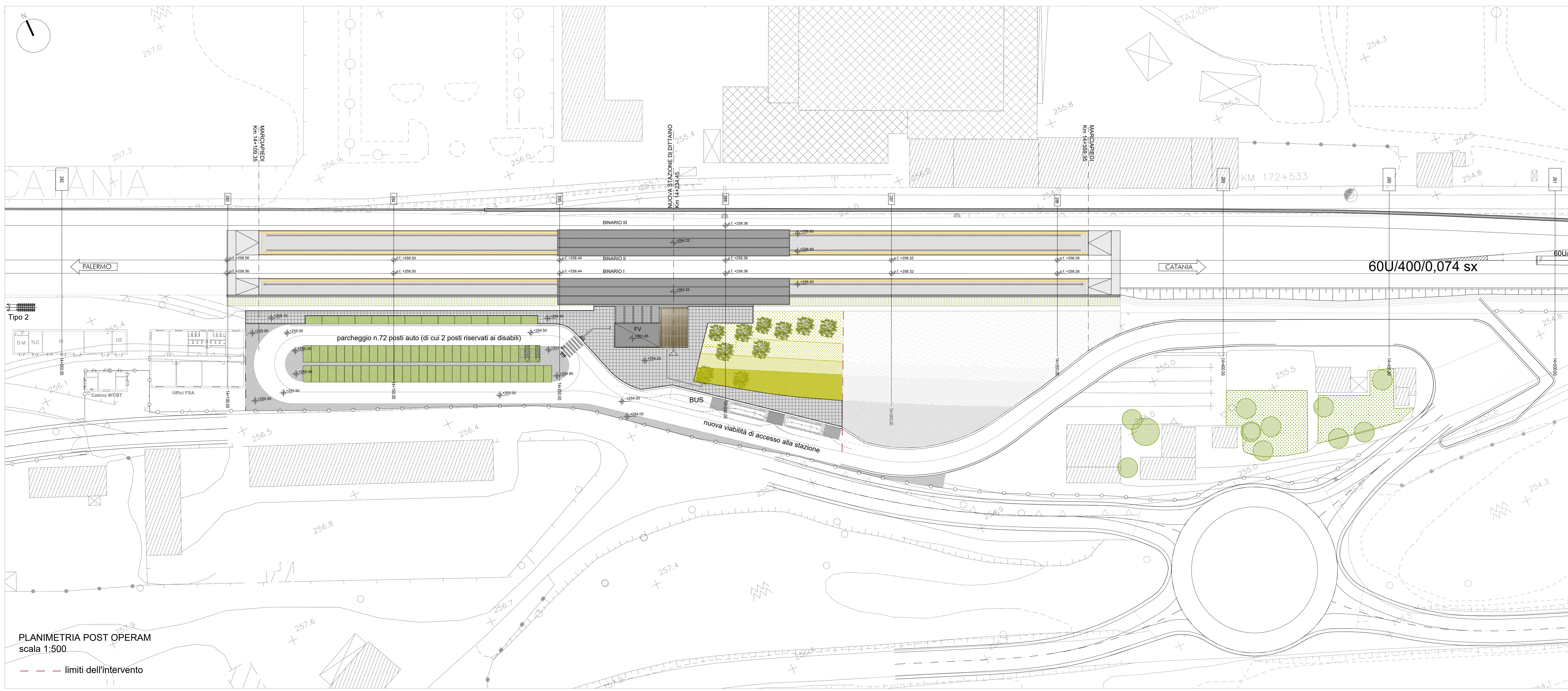
PLANIMETRIA ANTE OPERAM scala 1:500
