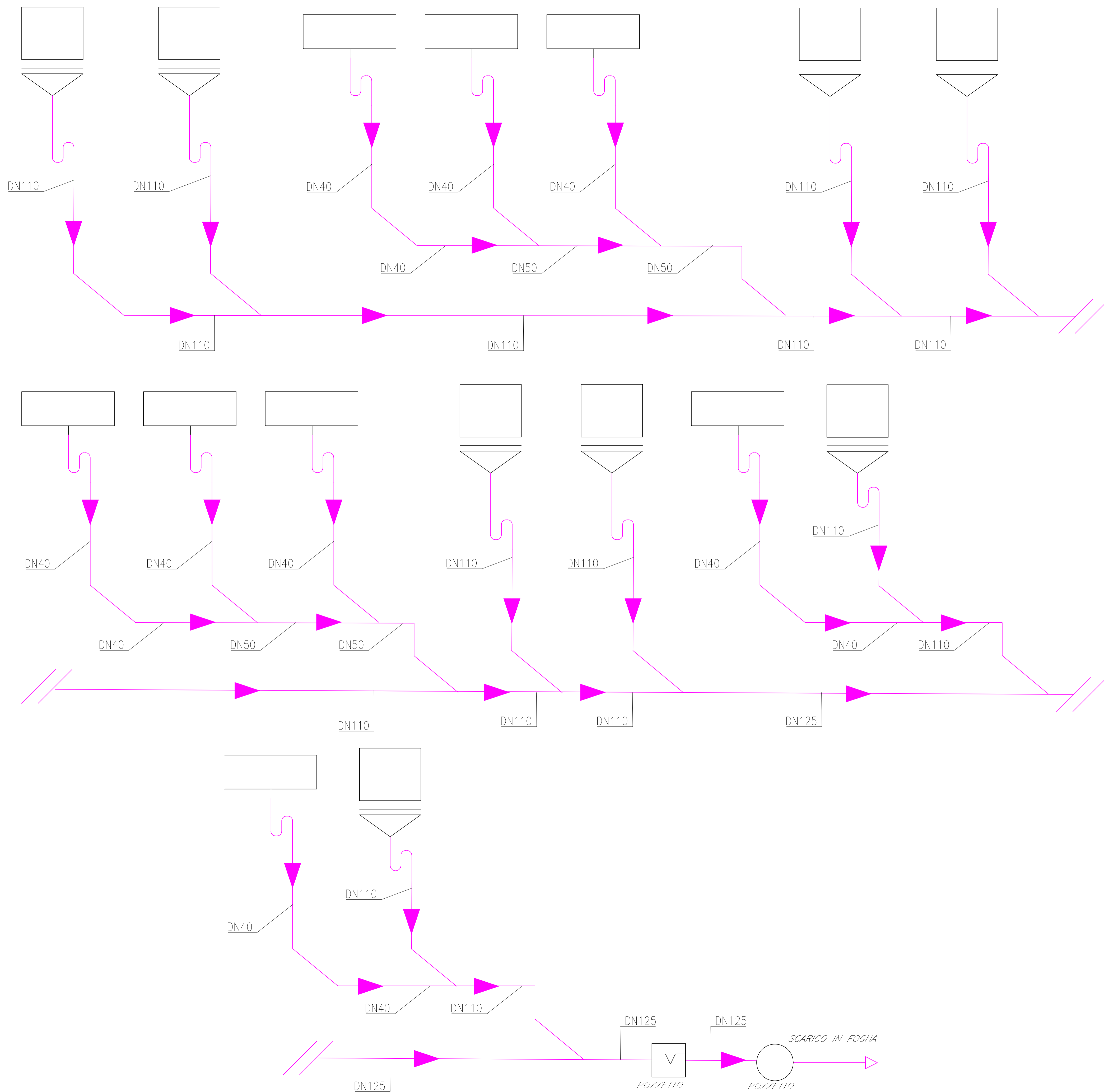
SCHEMA FUNZIONALE 1 IMPIANTO SCARICO ACQUE NERE - STAZIONE ENNA
