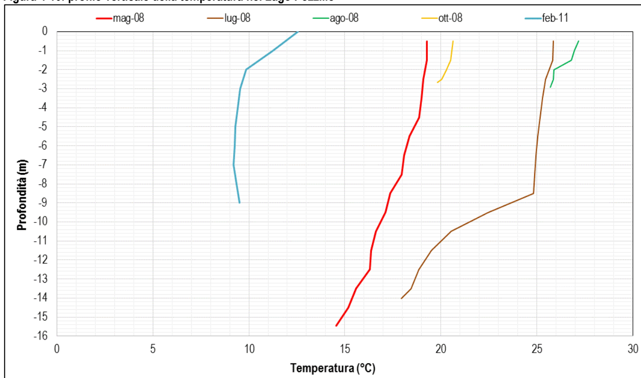
Figura 4-10: profilo verticale della temperatura nel Lago Pozzillo
