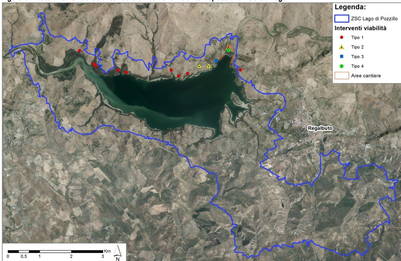
Figura 5-1: localizzazione aree di cantiere e interventi viabilità rispetto alla ZSC e al lago
