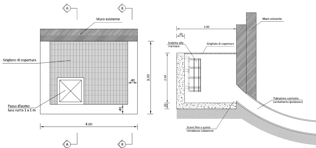
Figura 3-24: planimetria e sezione del nuovo pozzetto di progetto estratti dall'elaborato "Opere di regimentazione idraulica_Carpenterie e armature pozzetto"
