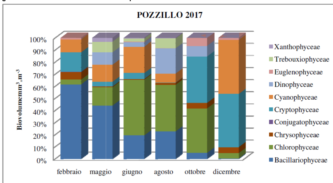
Figura 4-9: andamento delle abbondanze fitoplanctoniche
