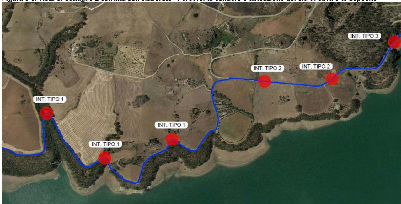
Figura 3-8: vista di dettaglio 2 estratta dall'elaborato "Percorsi di cantiere e ubicazione dei siti di cava e di deposito"
