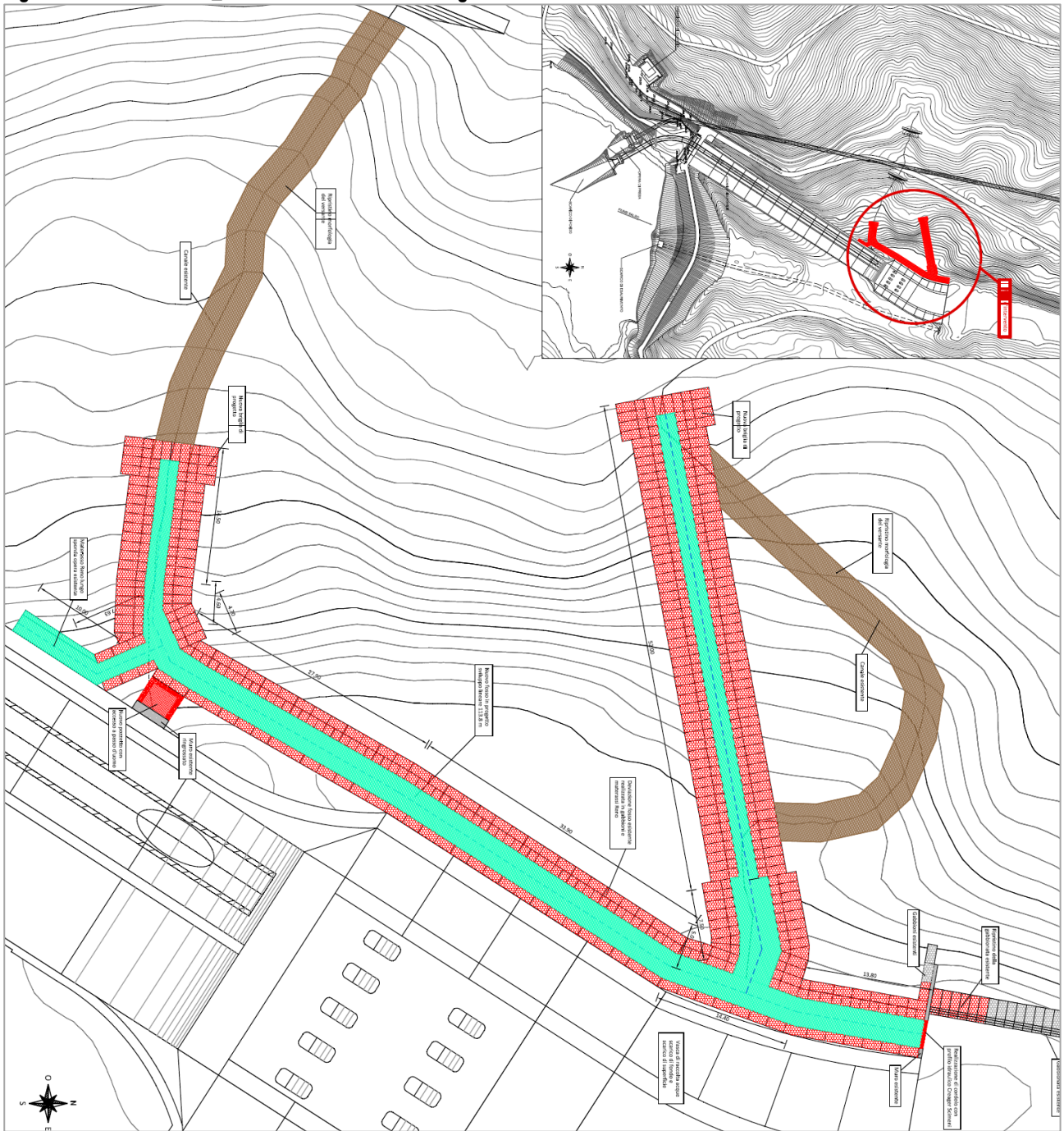
Figura 3-21: planimetria generale degli interventi in corrispondenza dell'area del dissesto estratta dall'elaborato "Opere di regimentazione idraulica_Planimetria e ubicazione degli interventi"
