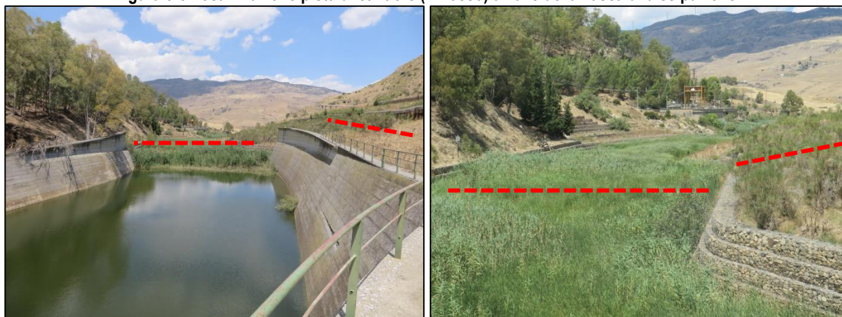
Figura 5-8: localizzazione pista di cantiere (in rosso) a valle della vasca di dissipazione
