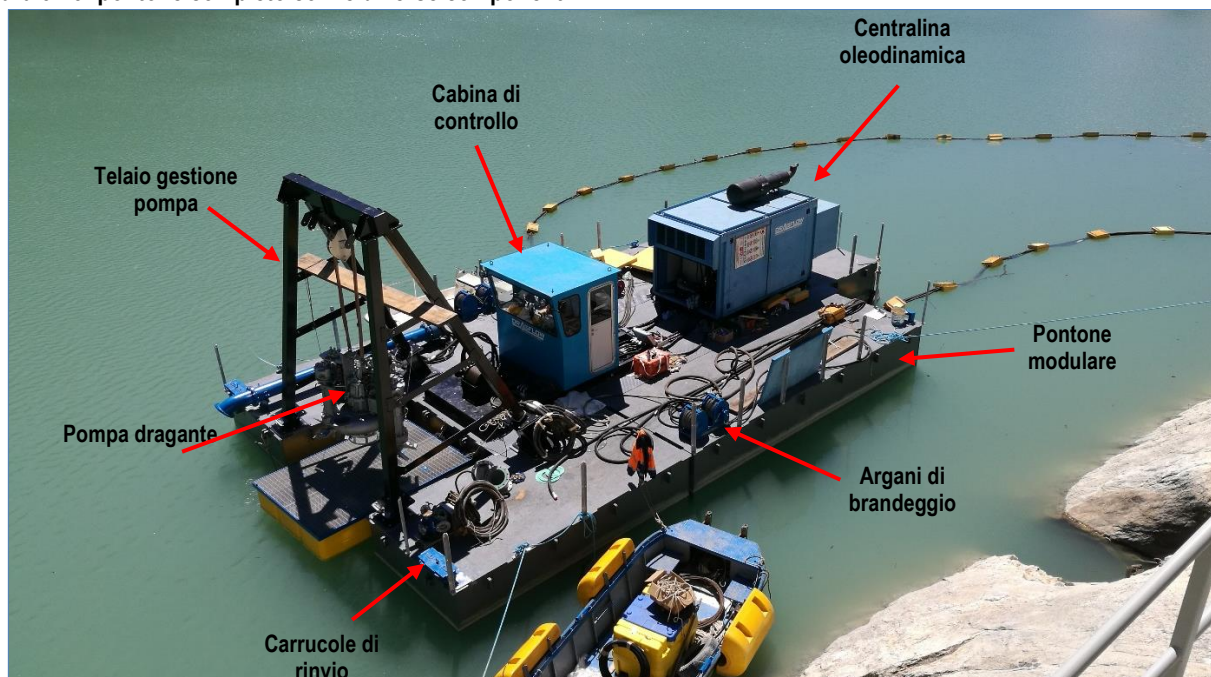
Figura 3-13: pontone completo con le diverse componenti
