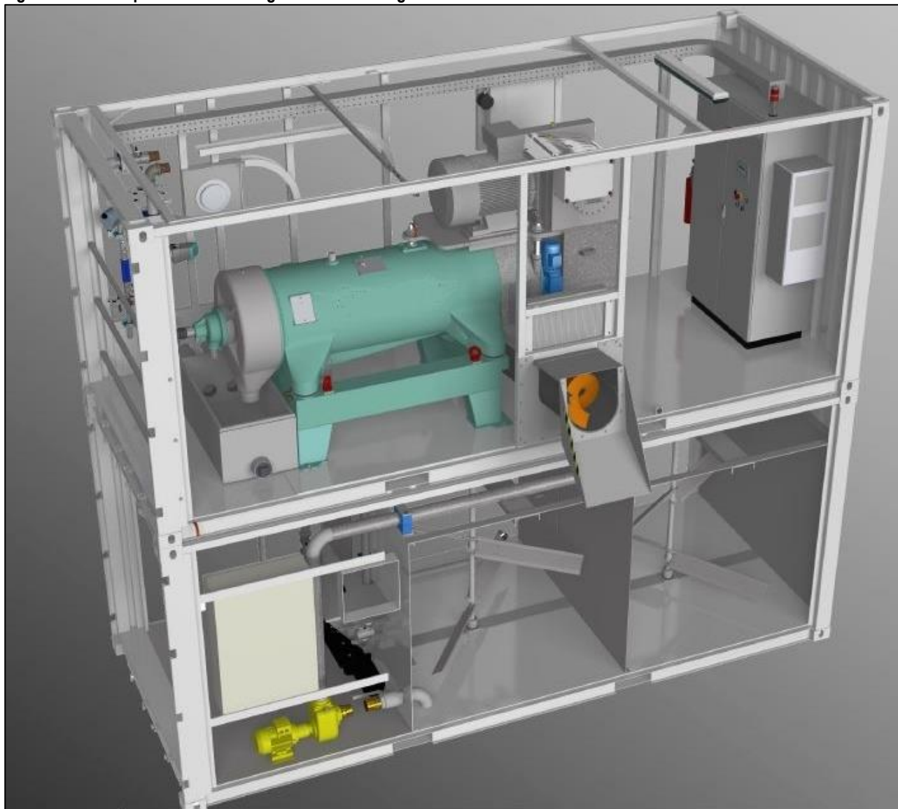
Figura 3-19: esempio di sistema integrato con centrifuga
