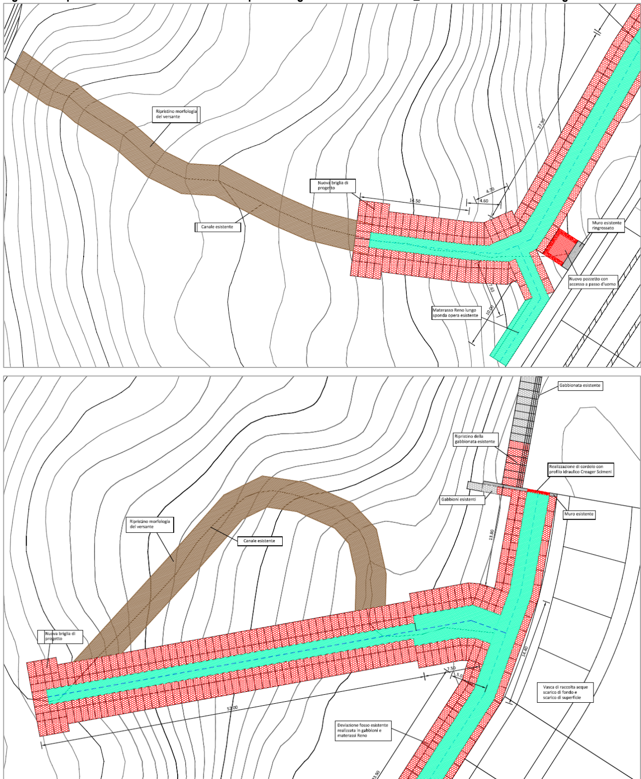
Figura 3-22: particolari estratti dall'elaborato "Opere di regimentazione idraulica_Planimetria e ubicazione degli interventi"
