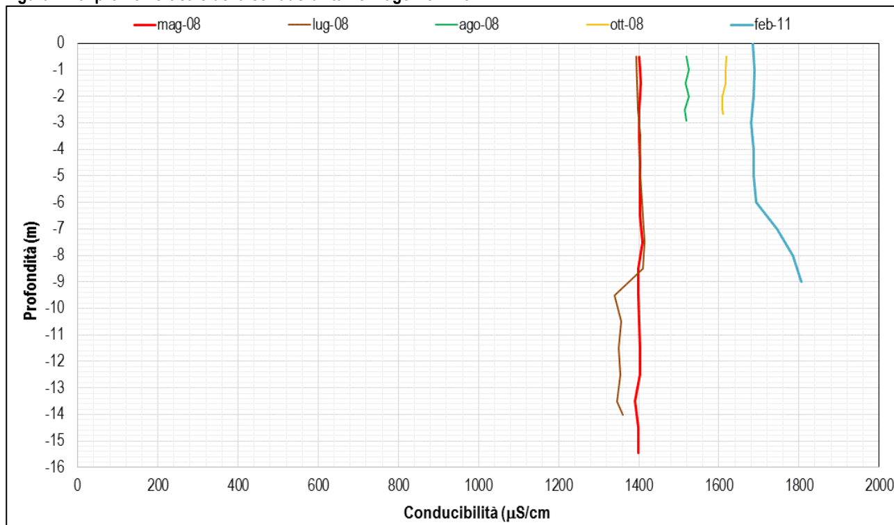
Figura 4-13: profilo verticale della conducibilità nel Lago Pozzillo
