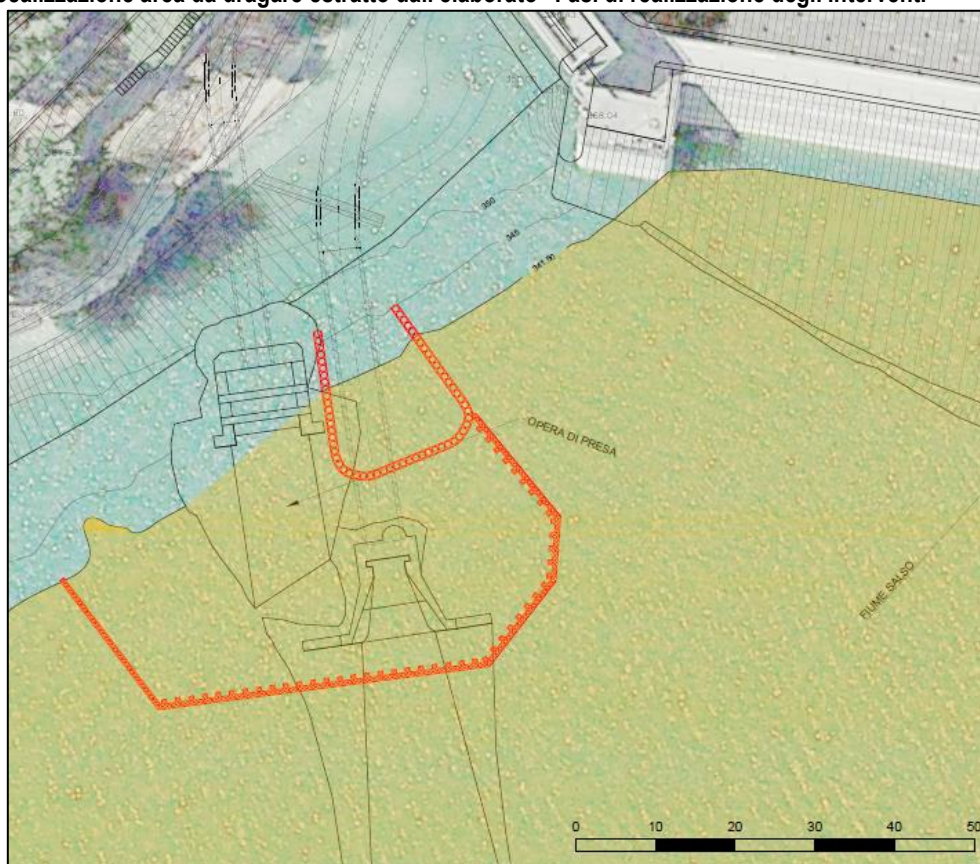
Figura 3-10: localizzazione area da dragare estratto dall'elaborato "Fasi di realizzazione degli interventi"
