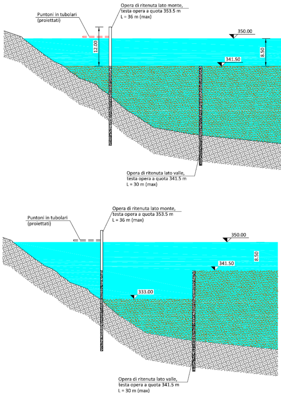
Figura 3-11: rimozione dei sedimenti estratti dall'elaborato "Opere di difesa e dragaggio: Fasi di realizzazione"
