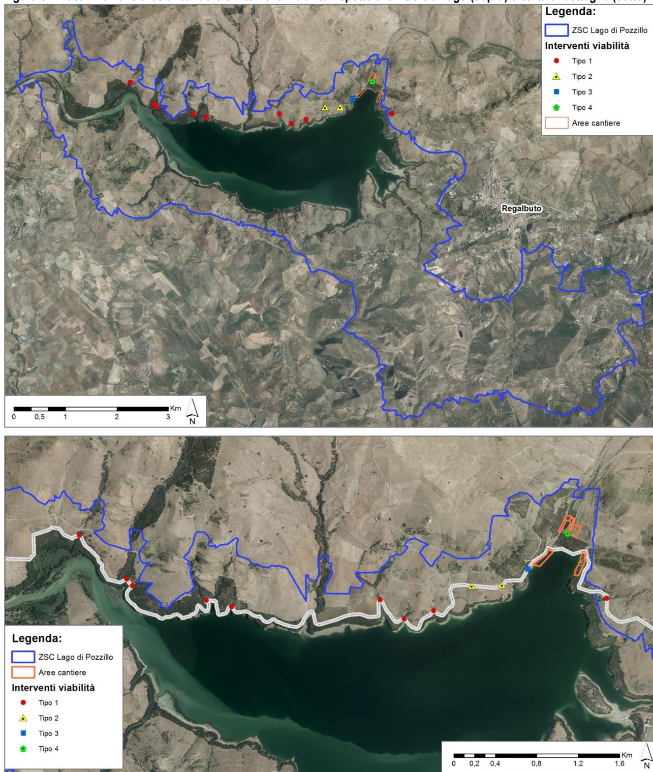
Figura 3-4: localizzazione aree di cantiere e interventi viabilità rispetto alla ZSC e al lago (sopra) e carta di dettaglio (sotto)
