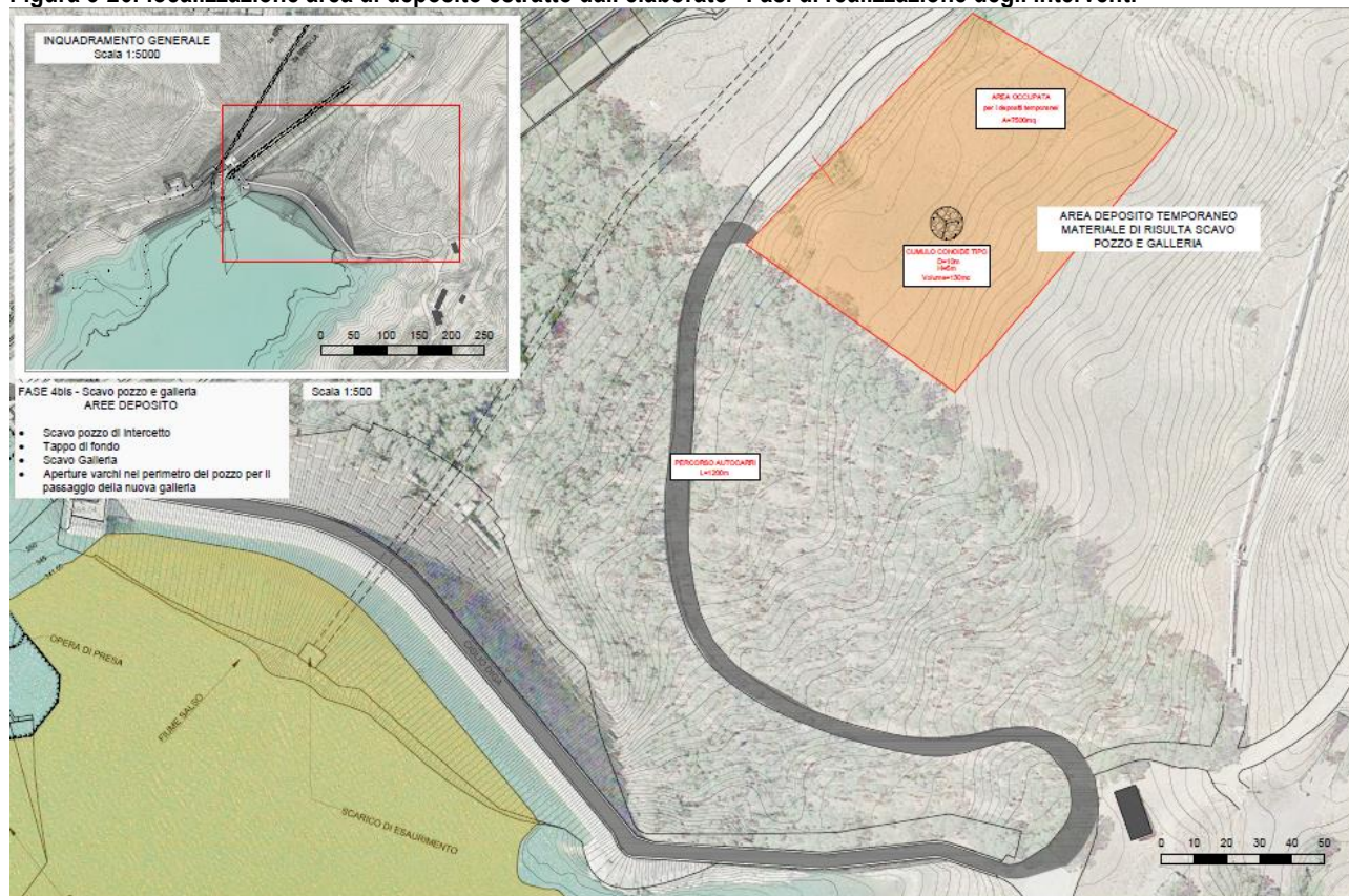
Figura 3-26: localizzazione area di deposito estratto dall'elaborato "Fasi di realizzazione degli interventi"
