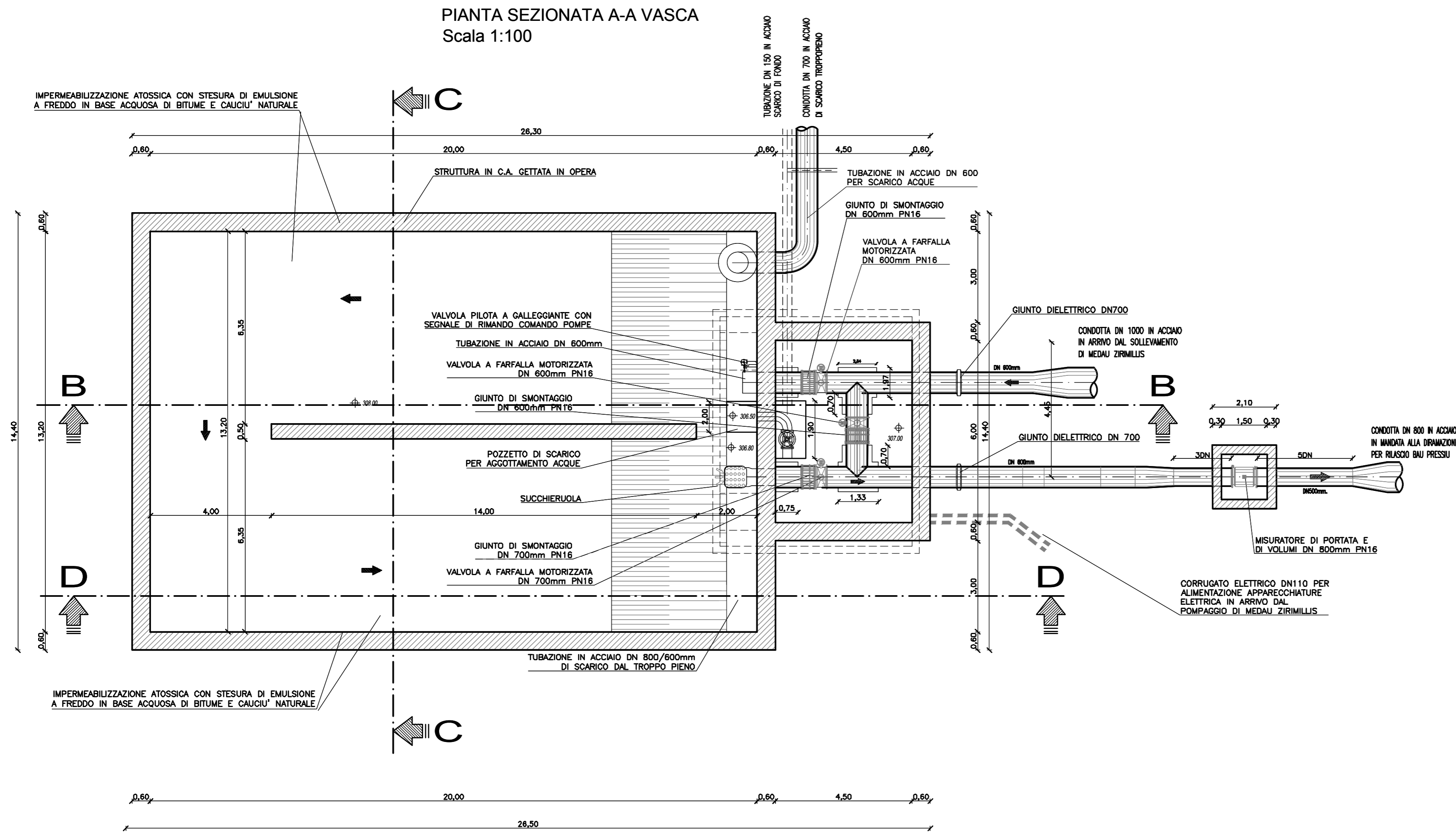
PIANTA VASCA Scala 1:100
